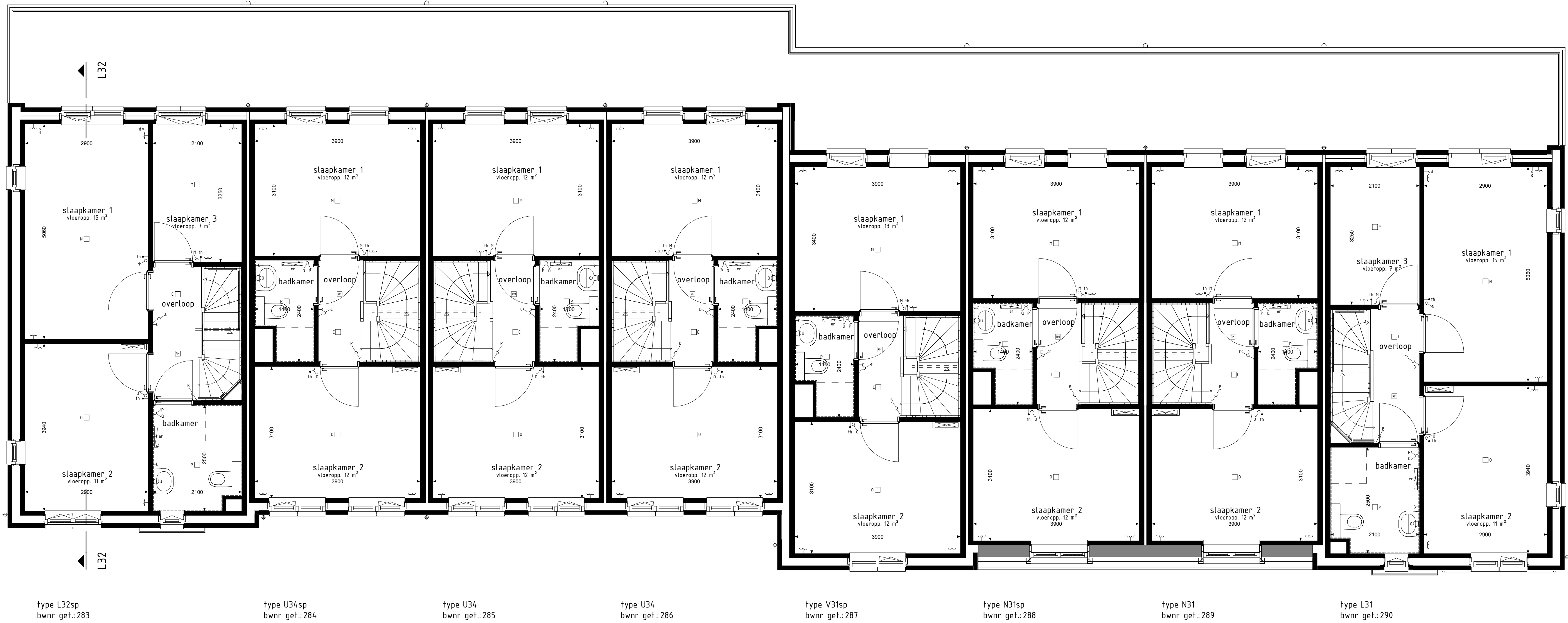
1e VERDIEPING
