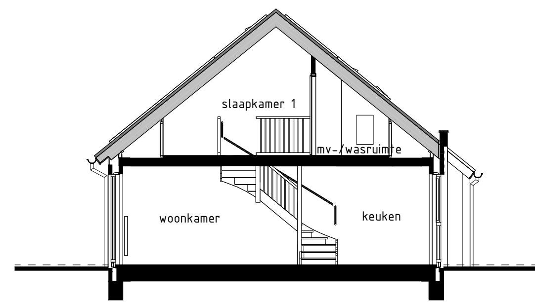
type H2, H2s bwnr get.:139 bwnr gesp.:135 DOORSNEDE H2-H2
