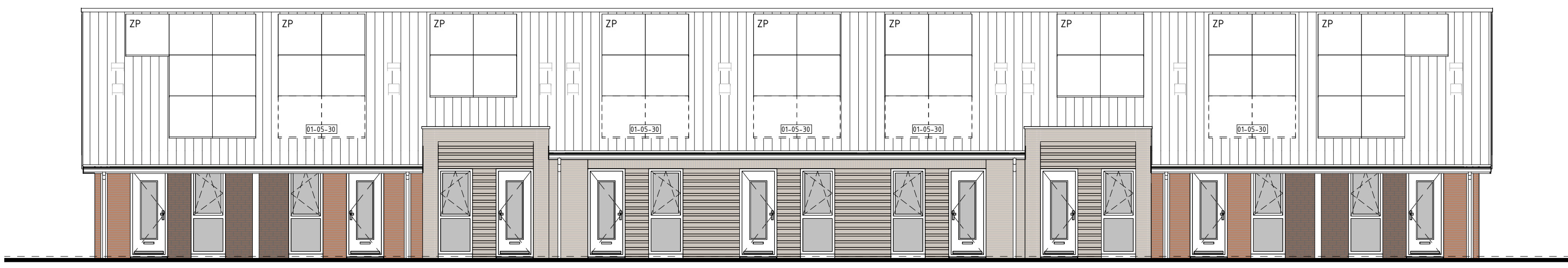
type G1 bwnr get.:133 VOORGEVEL type H1s bwnr get.:134 type H2s bwnr get.:135 type H3 bwnr get.:136 type H3 bwnr get.:137 type H3s bwnr get.:138 type H2 bwnr get.:139 type H1 bwnr get.:140 type G2s bwnr get.:141
