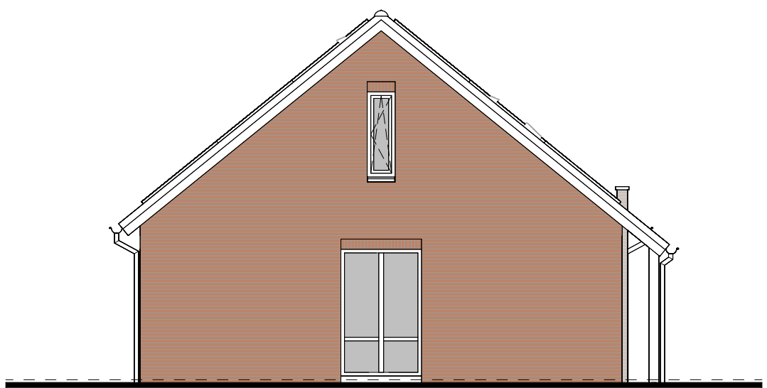
type G1 bwnr get.:133 LINKERGEVEL
