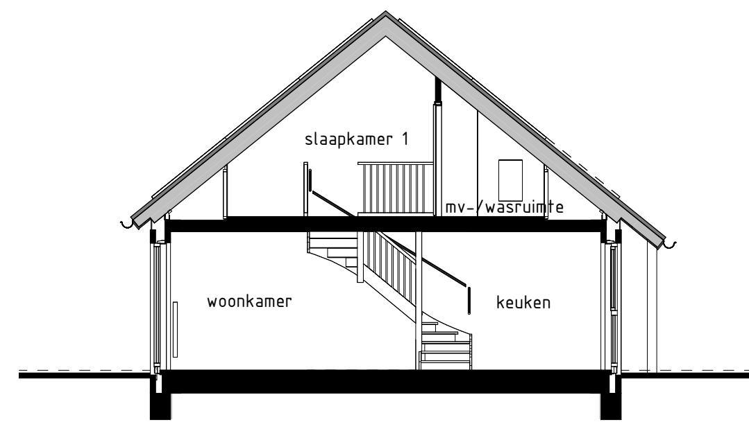
type G2s, H1, H1s bwnr get.:140 bwnr gesp.:134, 141 DOORSNEDE H1-H1
