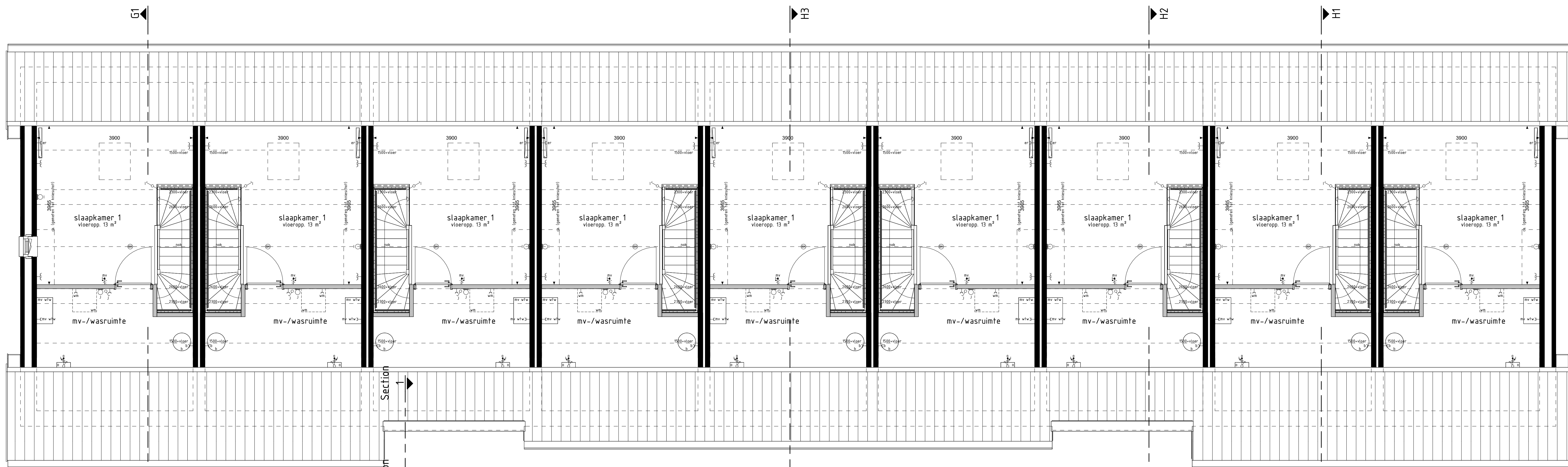
type G1 bwnr get.:133 1e VERDIEPING type H1s bwnr get.:134 type H2s bwnr get.:135 type H3 bwnr get.:136 type H3 bwnr get.:137 type H3s bwnr get.:138 type H2 bwnr get.:139 type H1 bwnr get.:140 type G2s bwnr get.:141
