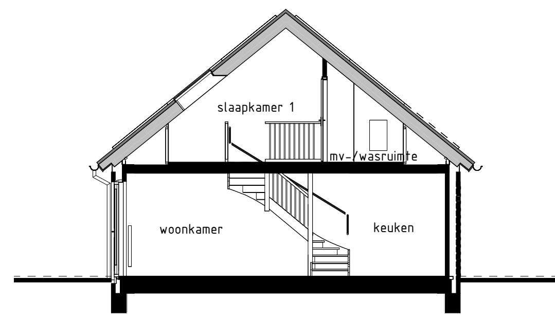
type H3 H3s bwnr get.:137, 138 bwnr gesp.:138 DOORSNEDE H3-H3
