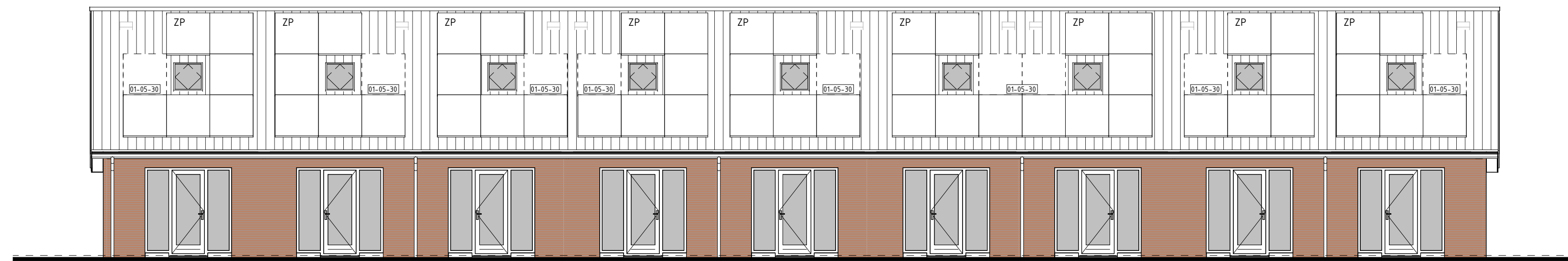
type G2s bwnr get.:141 ACHTERGEVEL type H1 bwnr get.:140 type H2 bwnr get.:139 type H3s bwnr get.:138 type H3 bwnr get.:137 type H3 bwnr get.:136 type H2s bwnr get.:135 type H1s bwnr get.:134 type G1 bwnr get.:133
