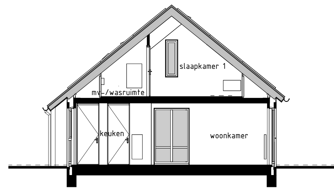
type G1 bwnr get.:133 DOORSNEDE G1-G1
