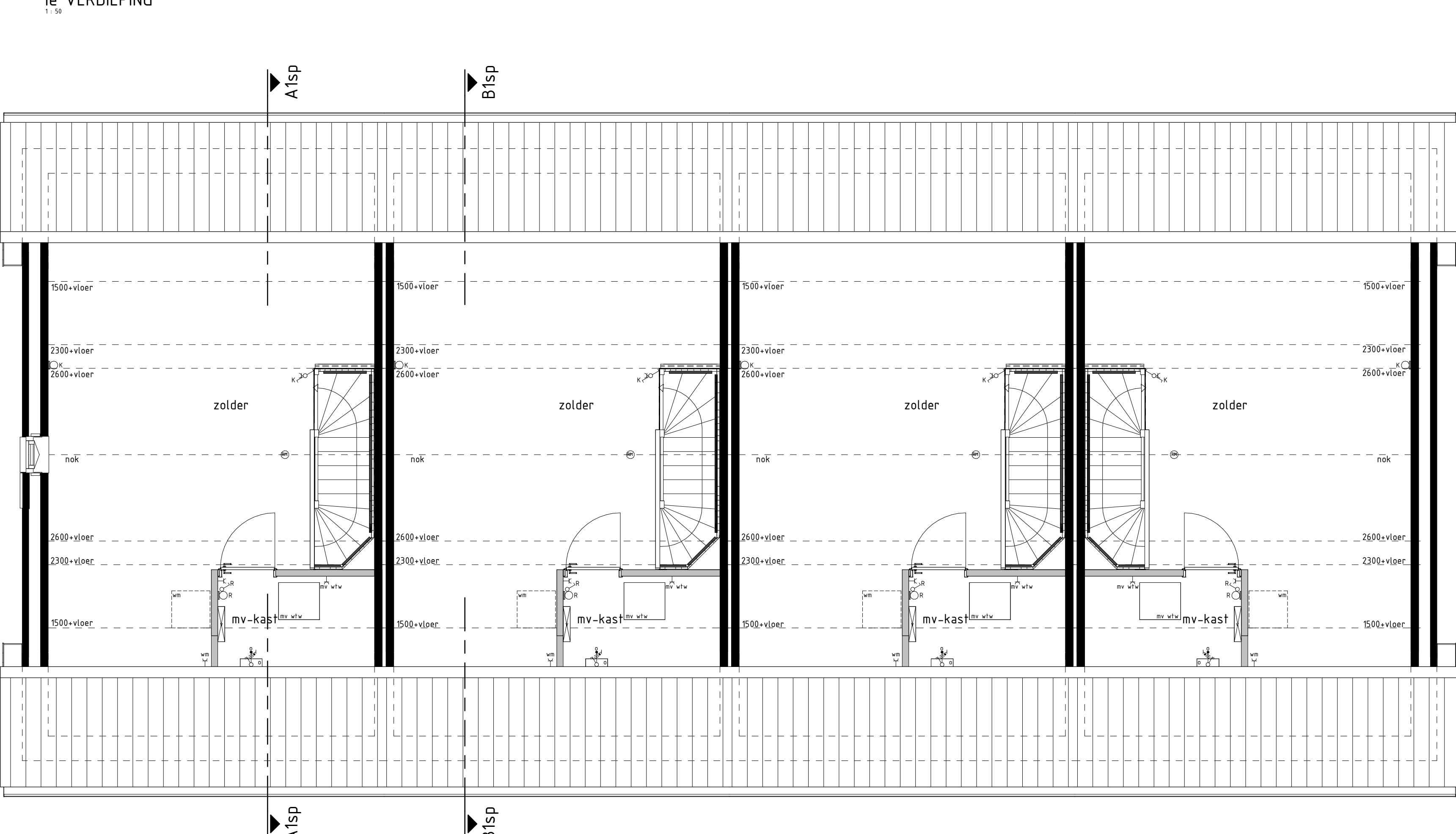
type A1sp bwnr get.:1 2e VERDIEPING
