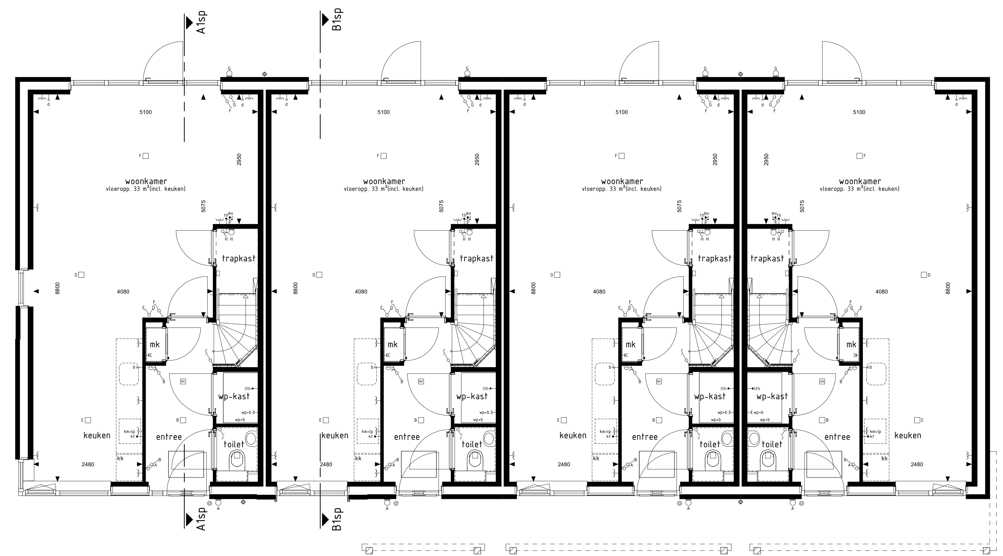
type A1sp bwnr get.:1 BEGANE GROND
