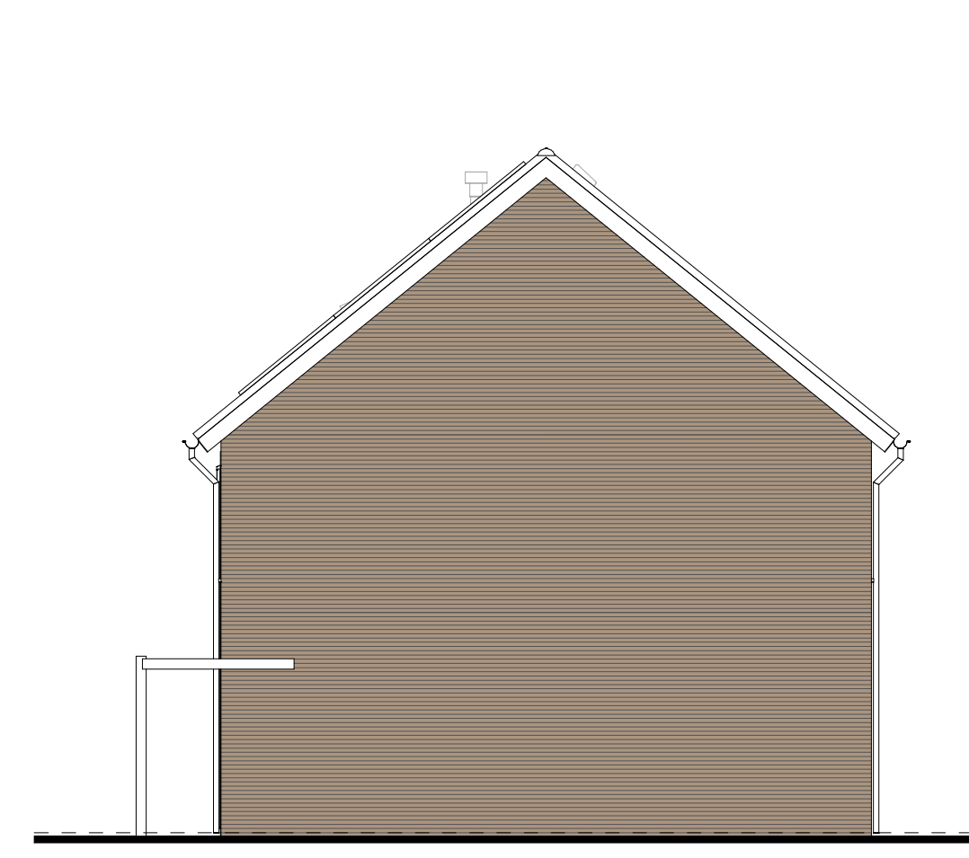
type A2 bwnr get.:4 RECHTERGEVEL
