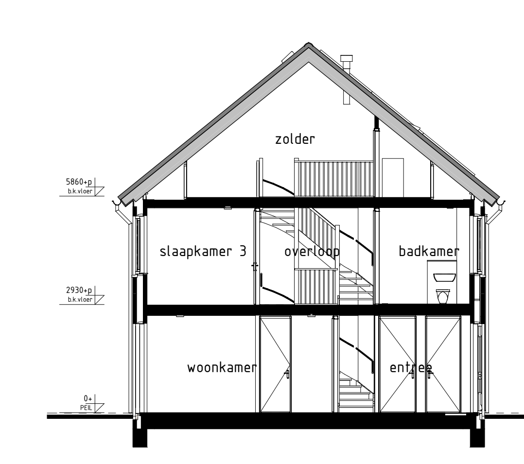
type A1sp, A2, B2sp bwnr get.:1, 3 bwnr gesp.:4 DOORSNEDE A1sp-A1sp
