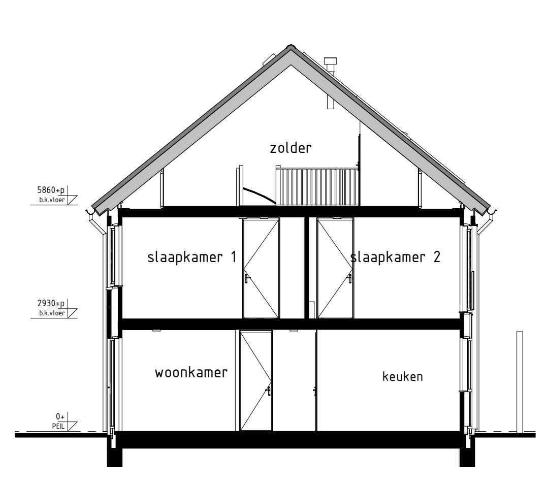
type B1sp bwnr get.:2 DOORSNEDE B1sp-B1sp
