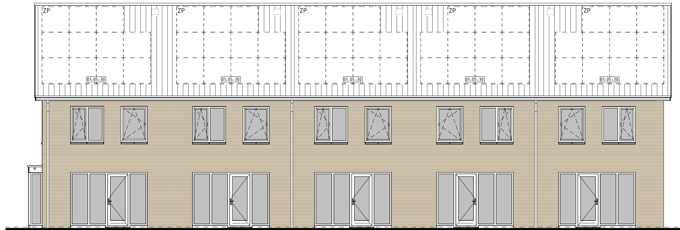
type A2 bwnr get.:84 ACHTERGEVEL 1:100
