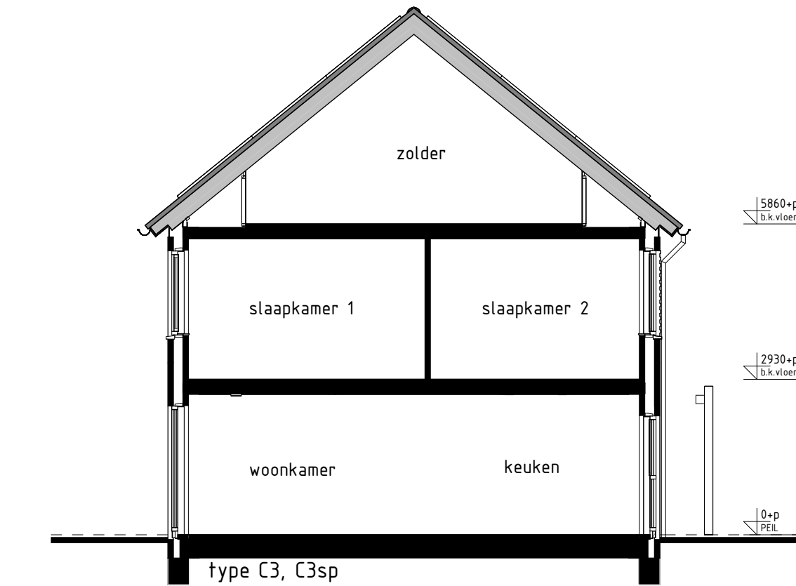
type C3, C3sp bwnr get.:83 bwnr gesp.:81 DOORSNEDE C3-C3 1:100
