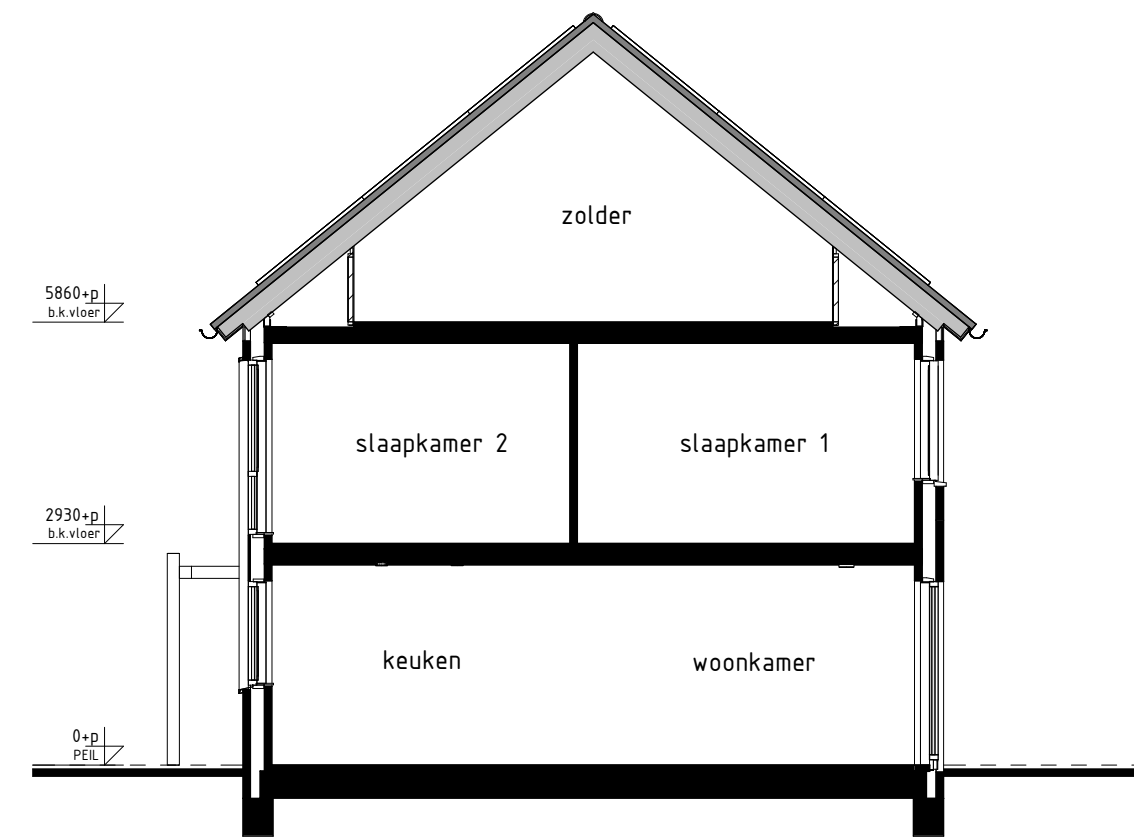
type A3sp bwnr get.:80 DOORSNEDE A3sp-A3sp 1:100
