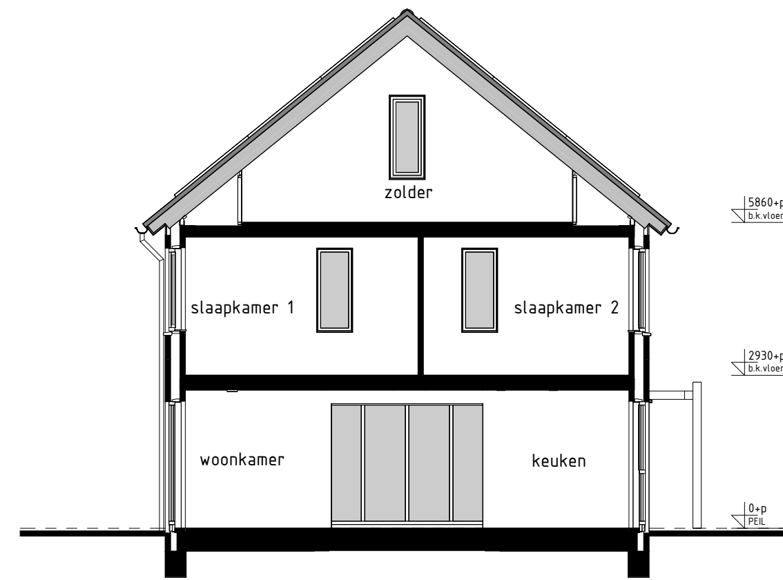
type A2 bwnr get.:84 DOORSNEDE A2-A2 1:100
