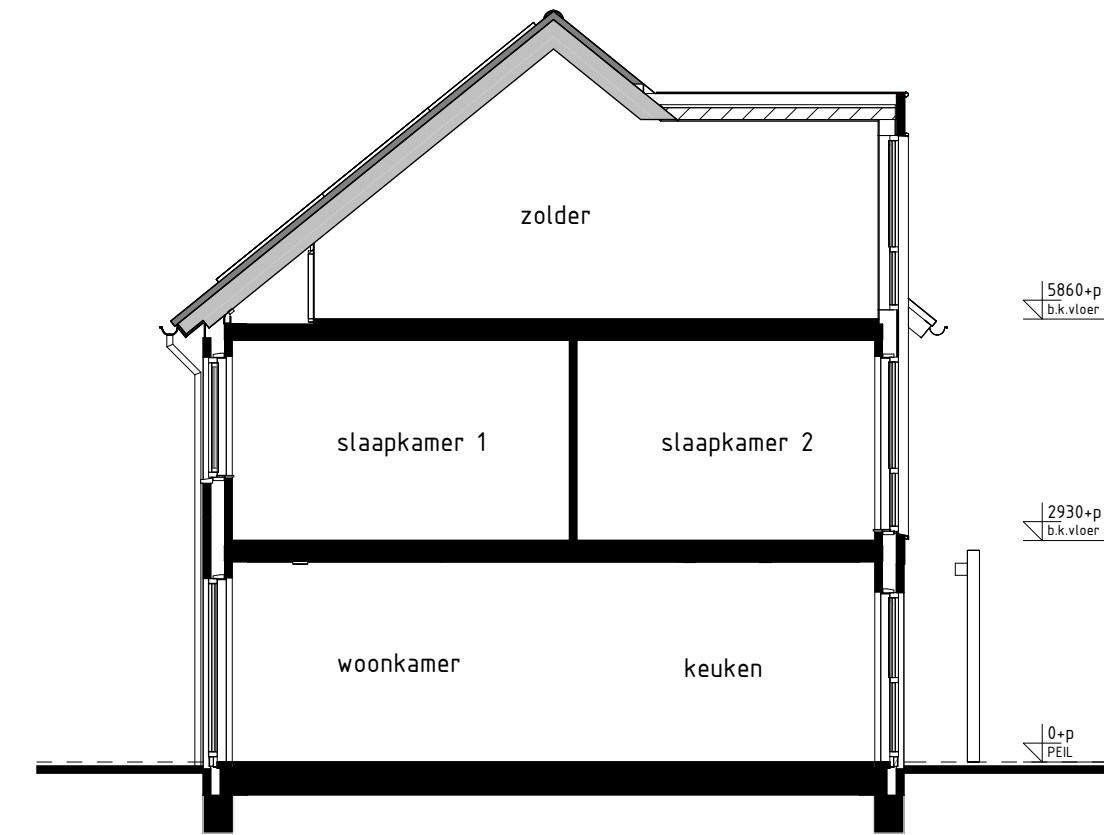
type B2 bwnr get.:82 DOORSNEDE B2-B2 1:100
