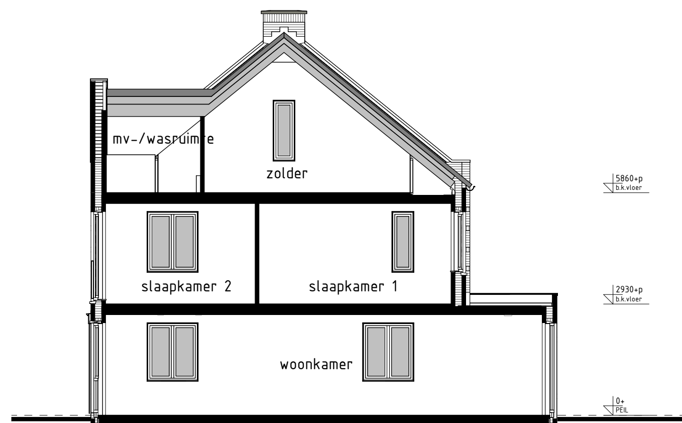
type L32sp bwnr get.:274 DOORSNEDE A-A 1:50
