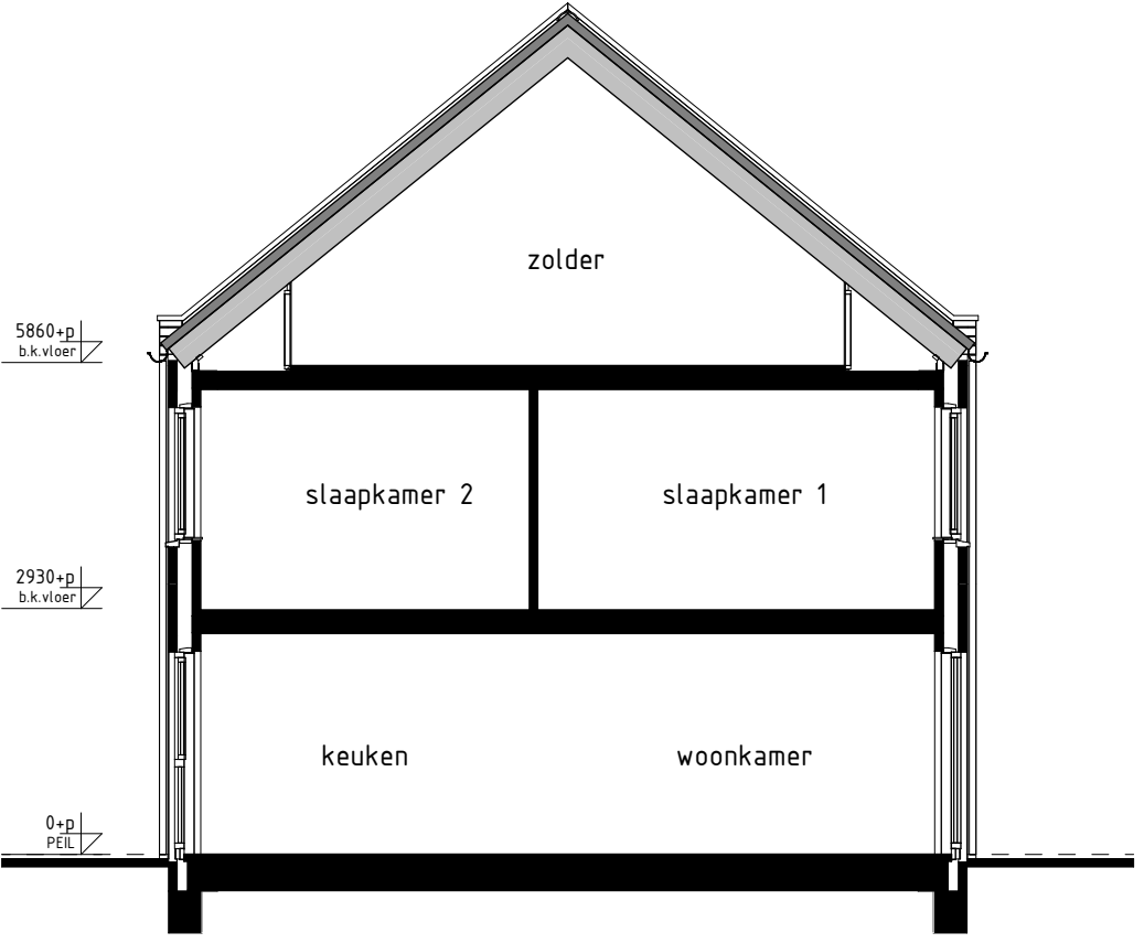
DOORSNEDE I2sp-I2sp
