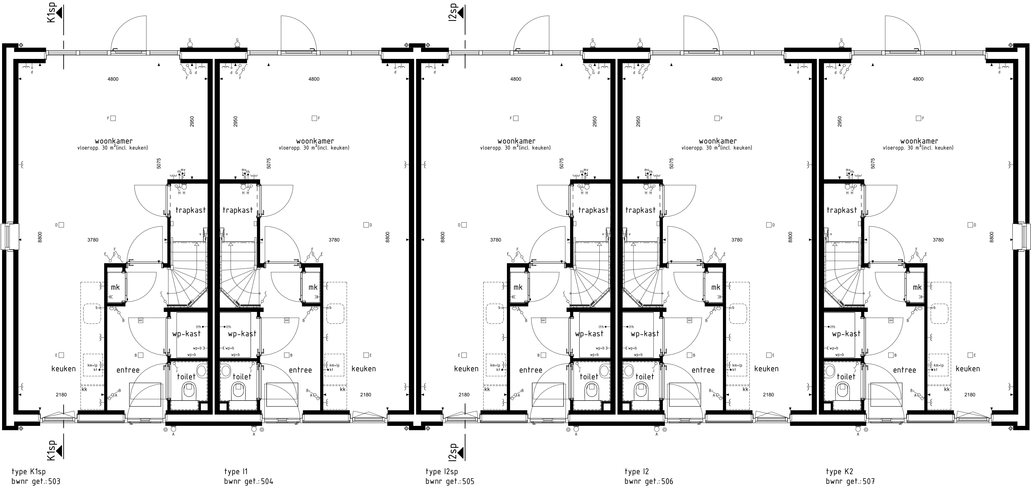
BEGANE GROND
