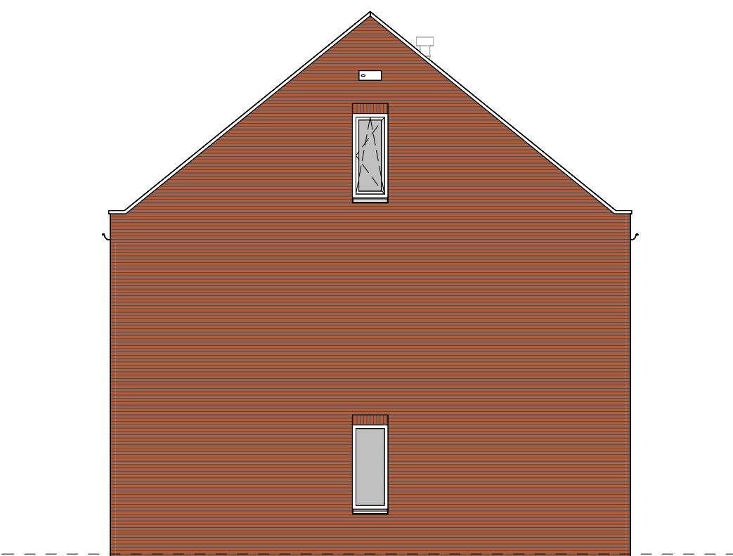
LINKERGEVEL
