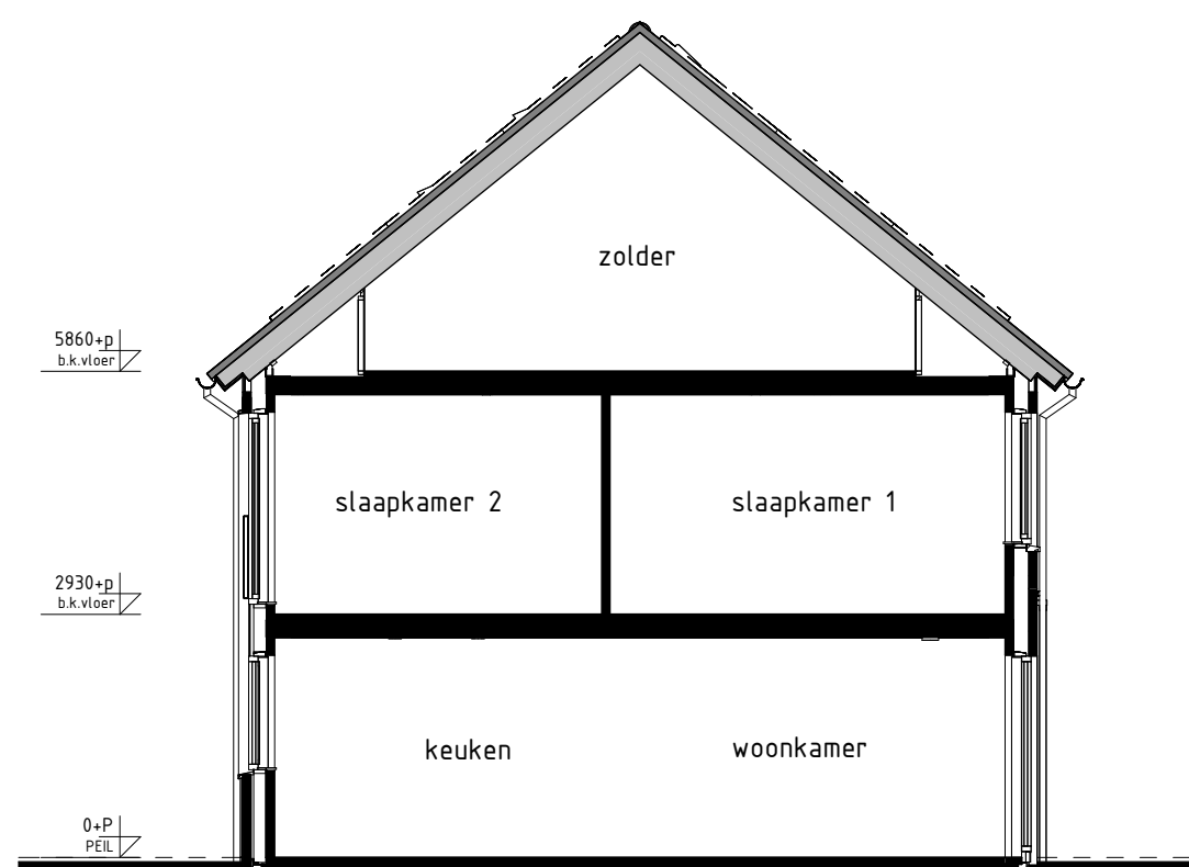
type B2sp, B3sp bwnr get.:226, 228 DOORSNEDE B2sp-B2sp
