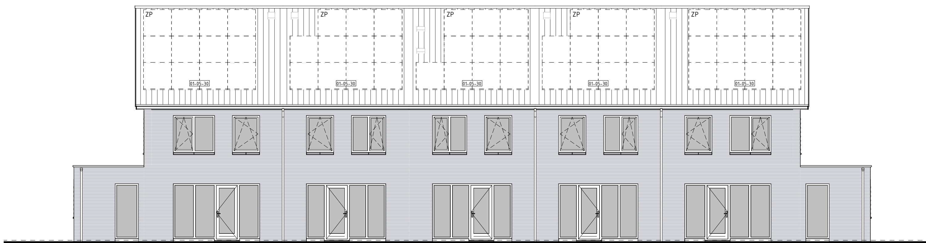
type H1 bwnr get.:229 ACHTERGEVEL type B3sp bwnr get.:228 type P1sp bwnr get.:227 type B2sp bwnr get.:226 type H1sp bwnr get.:225
