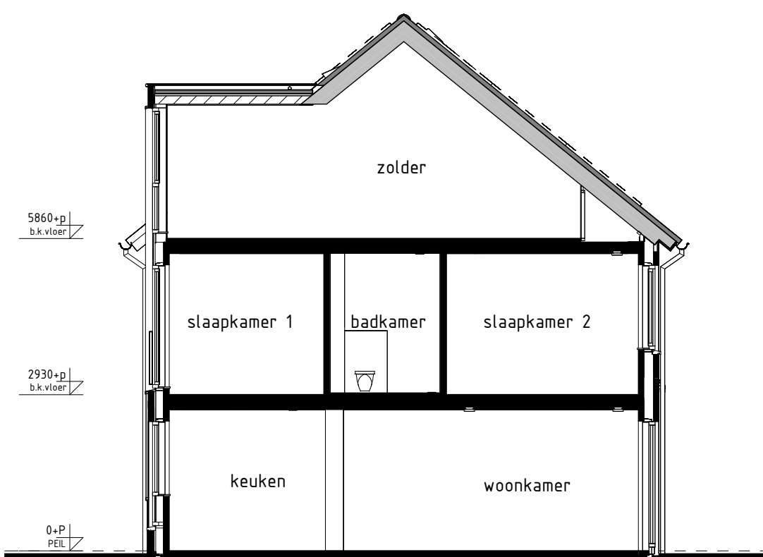
type P1sp bwnr get.:227 DOORSNEDE P1sp-P1sp
