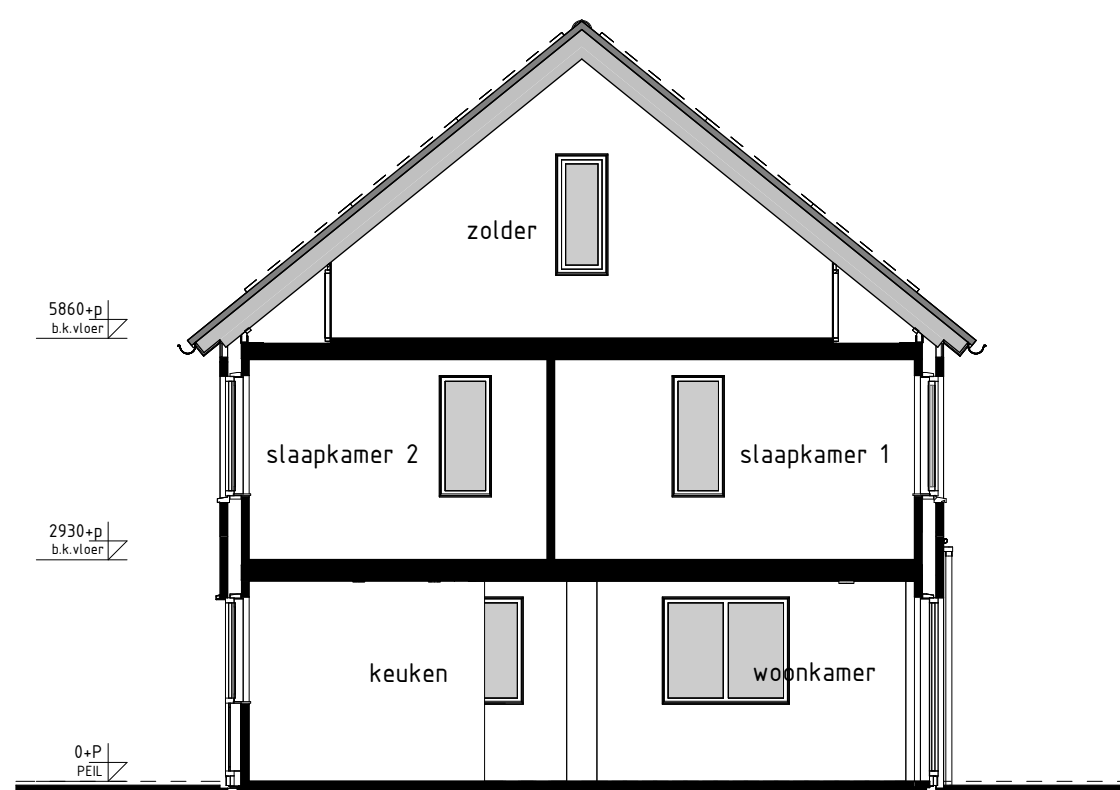
type H1, H1sp bwnr get.:225, 229 DOORSNEDE H1sp-H1sp
