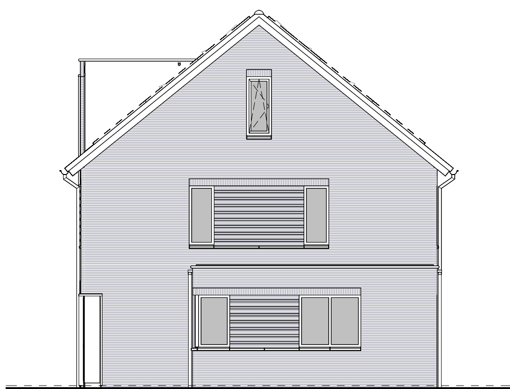
type H1 bwnr get.:229 RECHTERGEVEL
