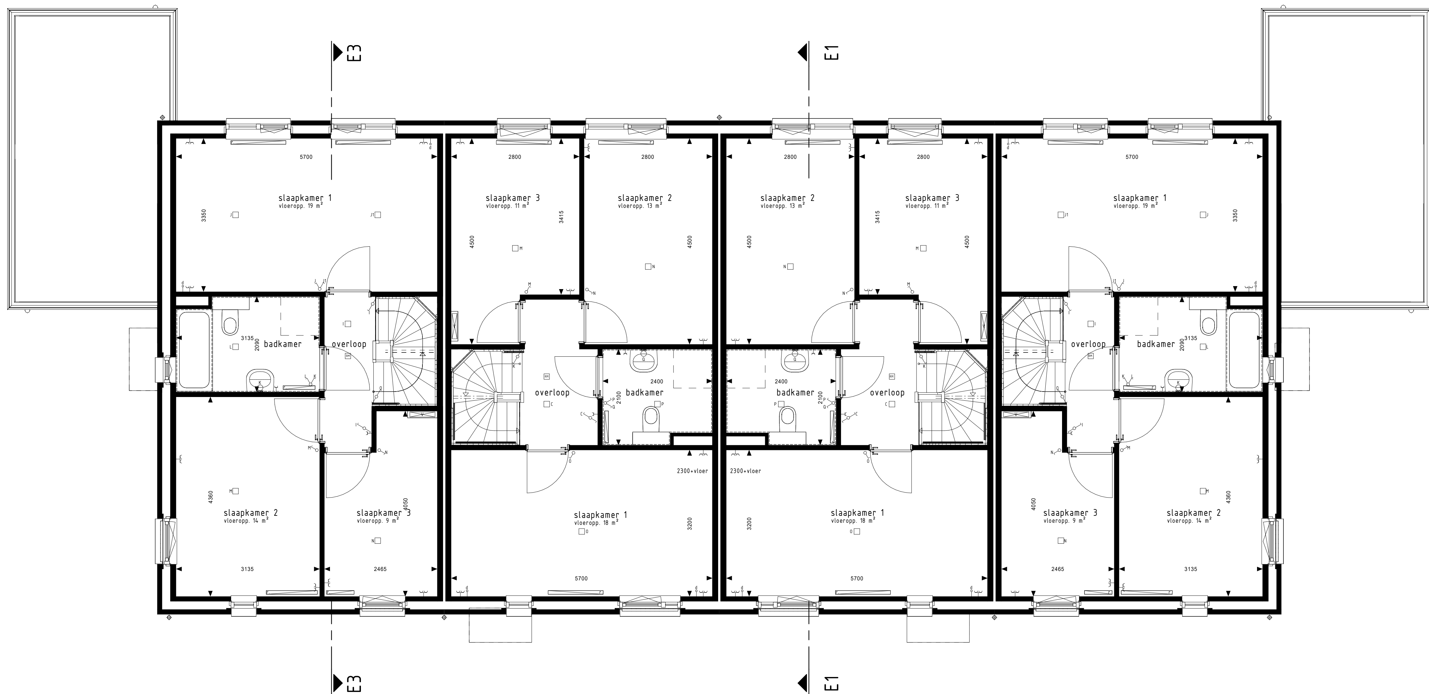
type D1 bwnr get.:316 1e VERDIEPING
