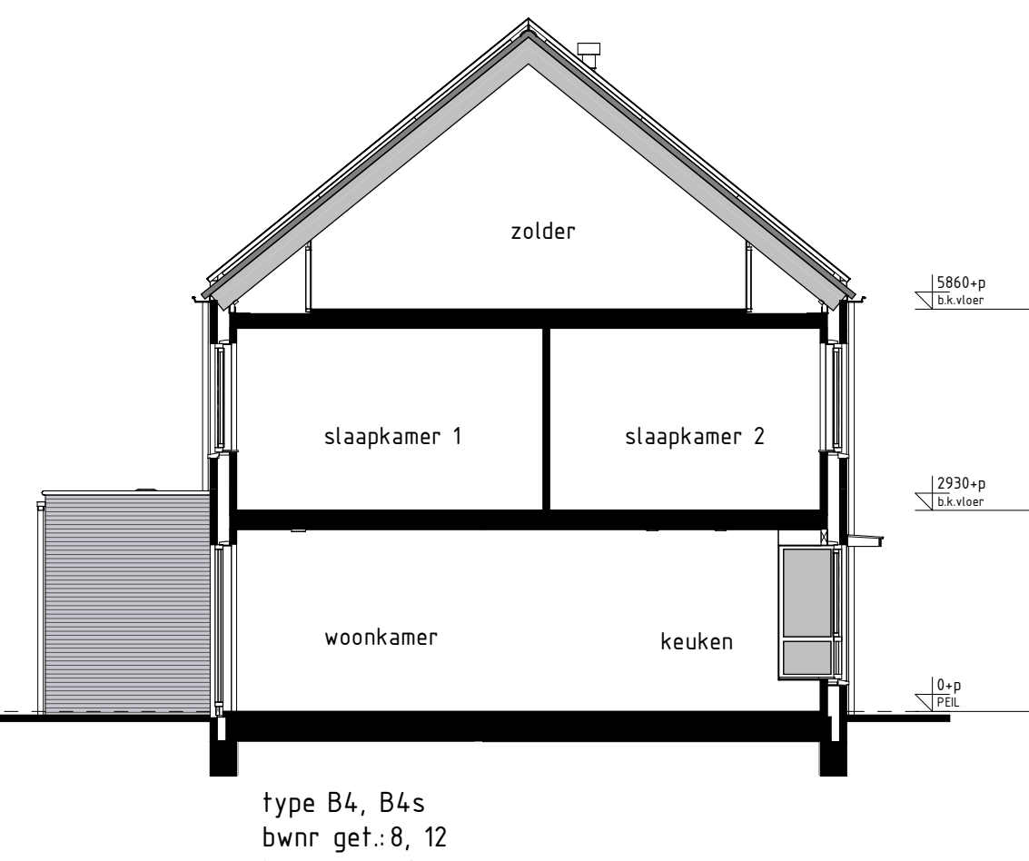
DOORSNEDE B4-B4
