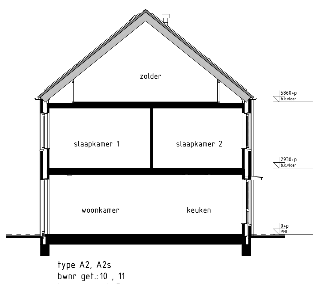
DOORSNEDE A2-A2
