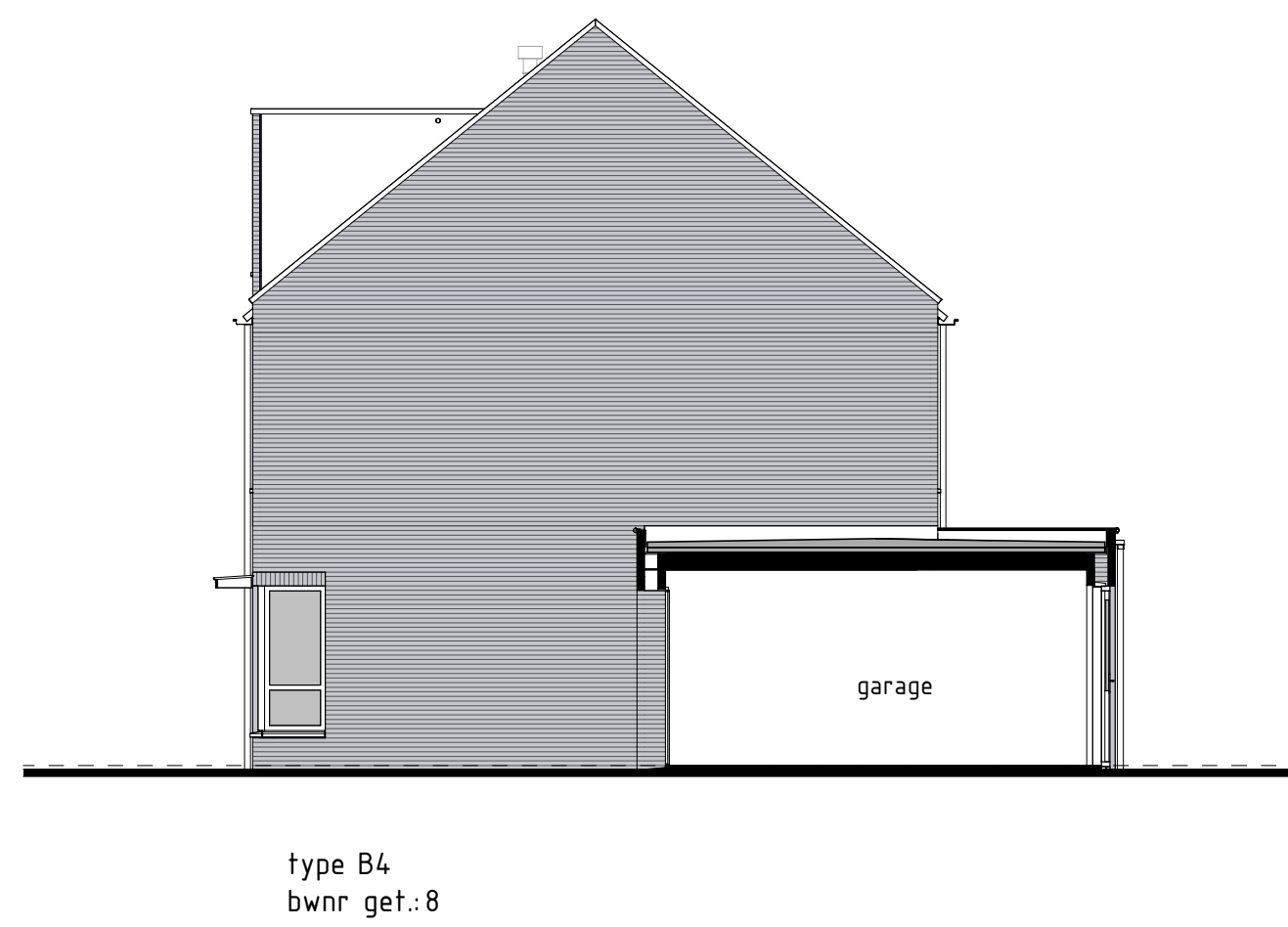
RECHTERGEVEL
