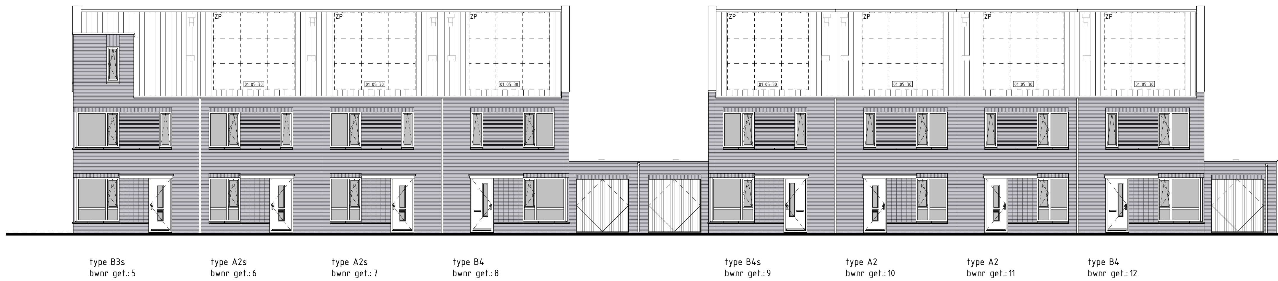
VOORGEVEL
