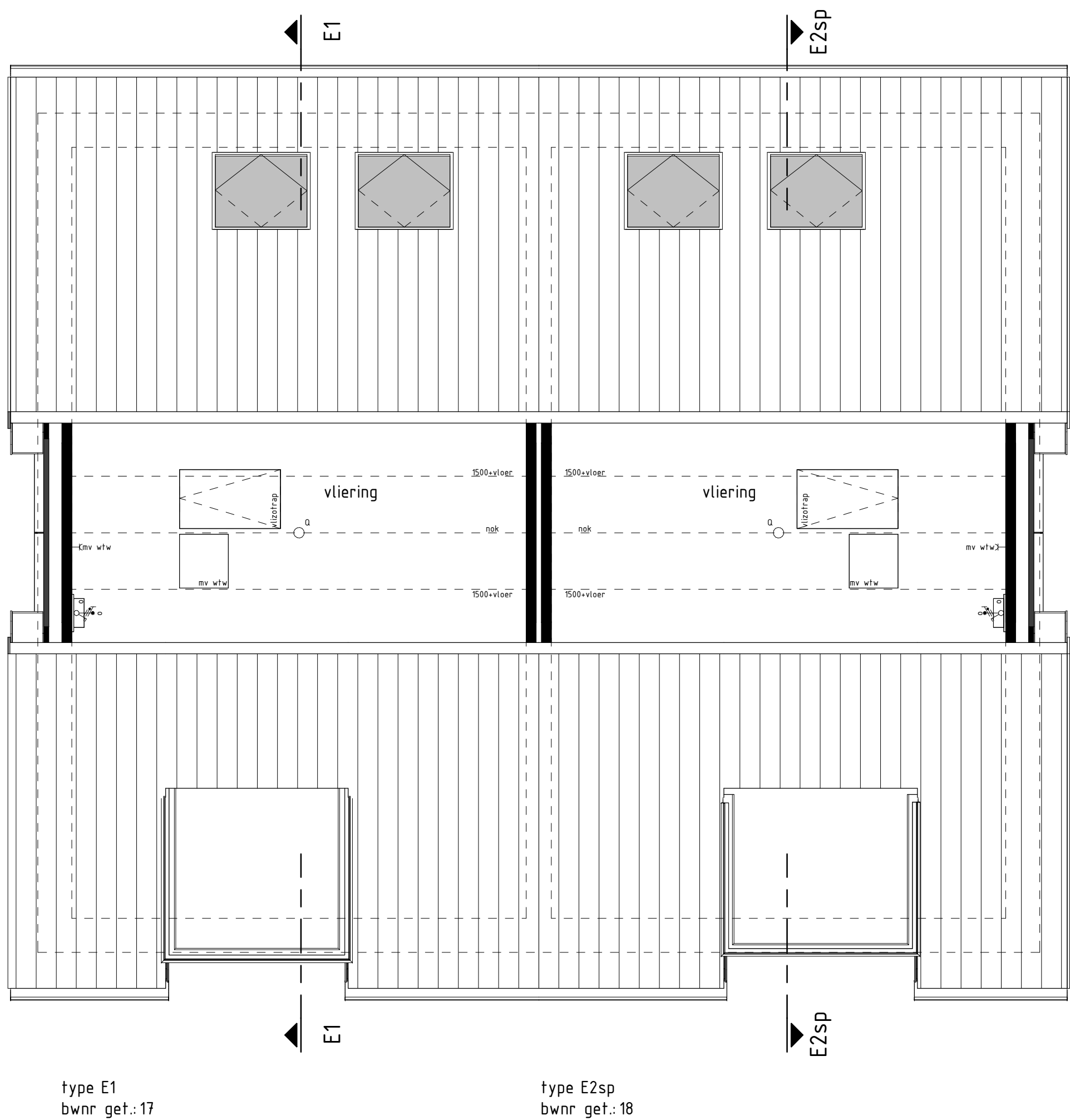
2e VERDIEPING
