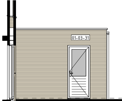
ZIJGEVEL 1: 50
