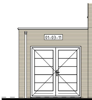
VOORGEVEL 1: 50
