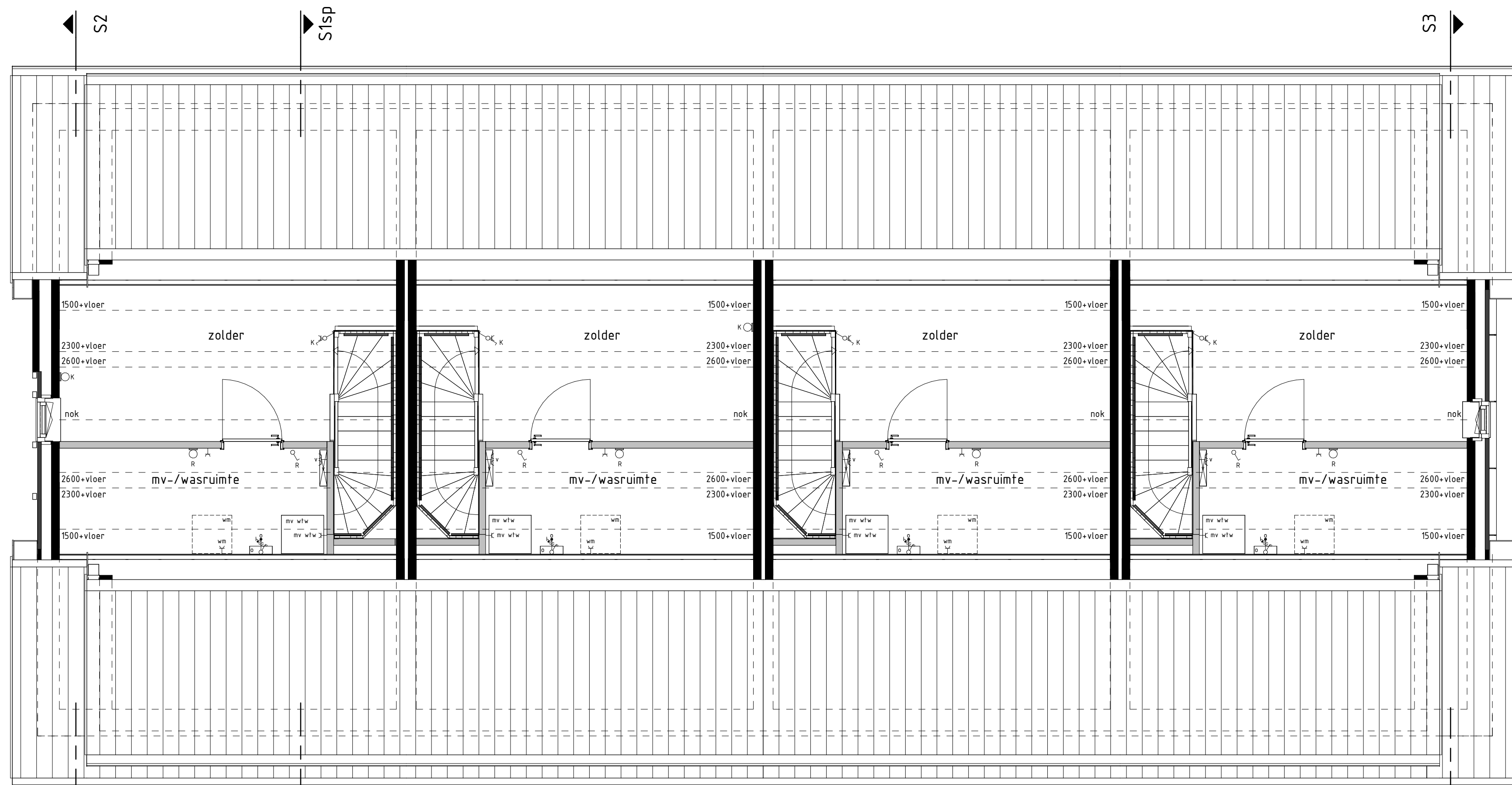
type S1sp bwnr get.:02 2e VERDIEPING 1:50
