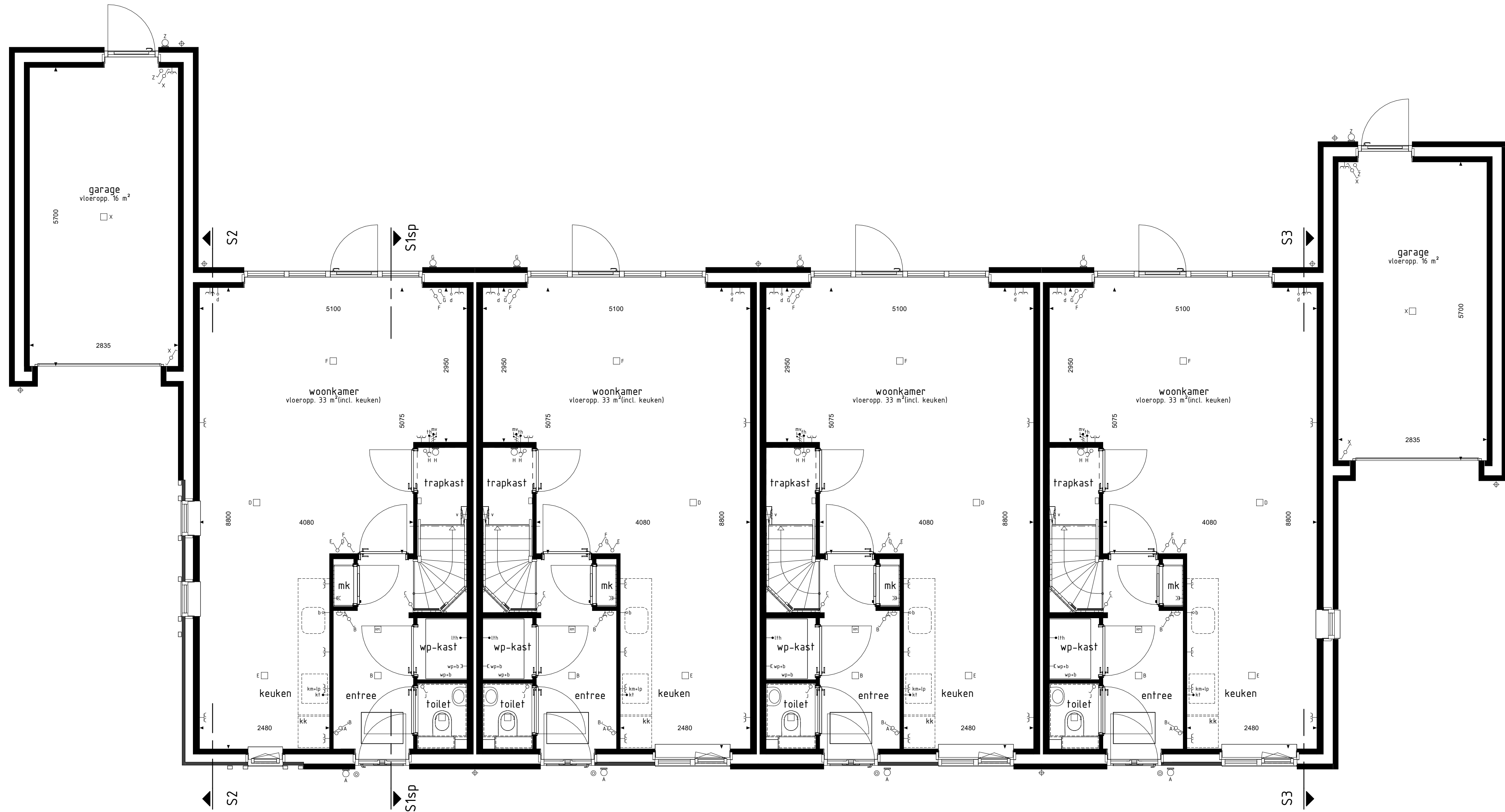
type S1sp bwnr get.:02 BEGANE GROND 1:50
