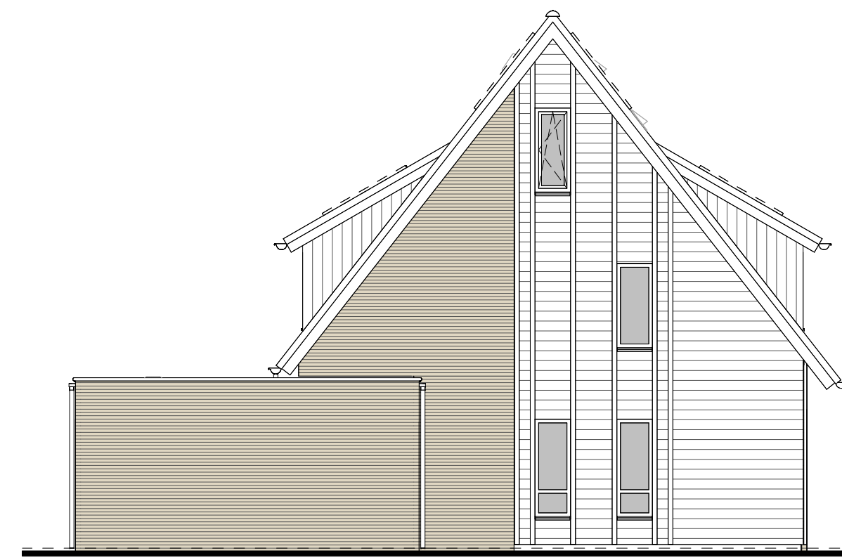
type S1sp bwnr get.:02 LINKERGEVEL 1:50
