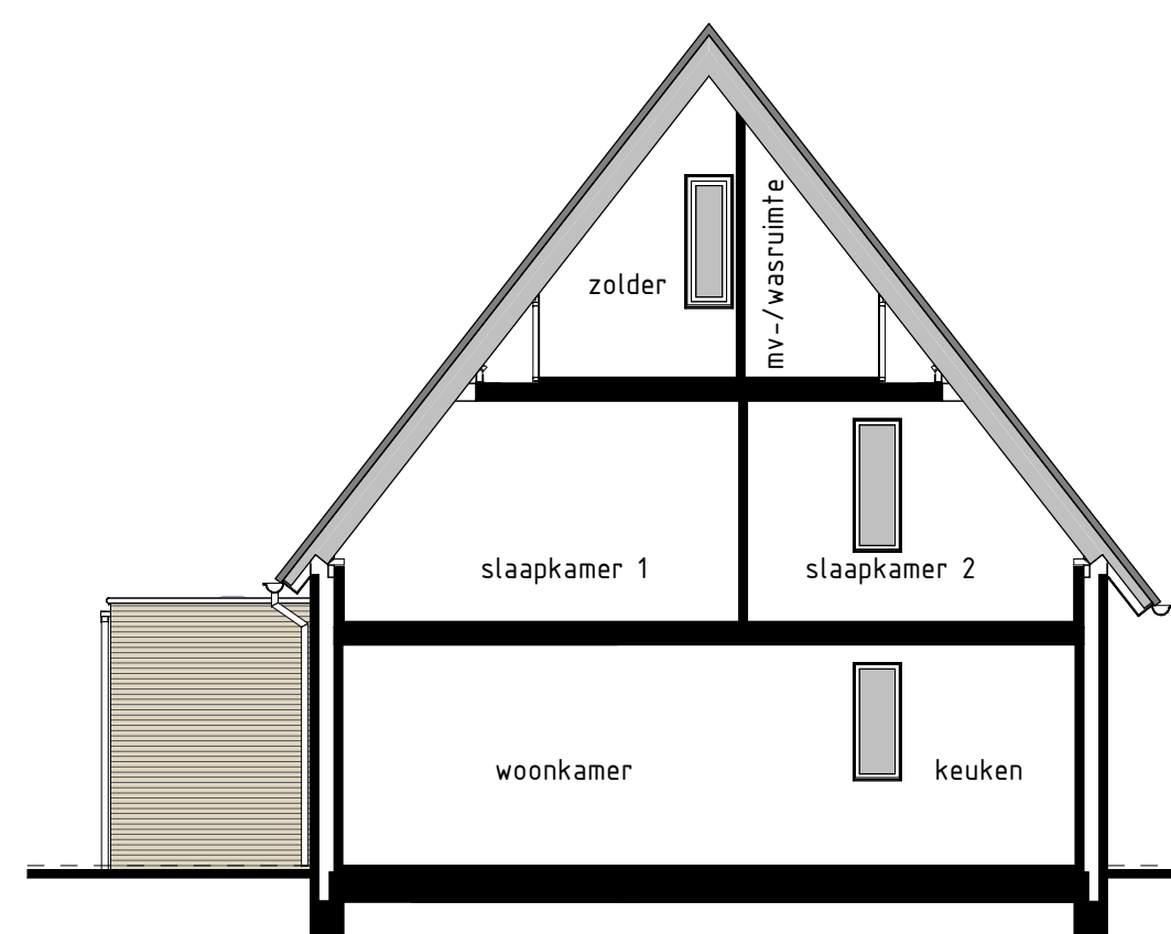
type S2 bwnr get.:05 DOORSNEDE S2-S3 1:50
