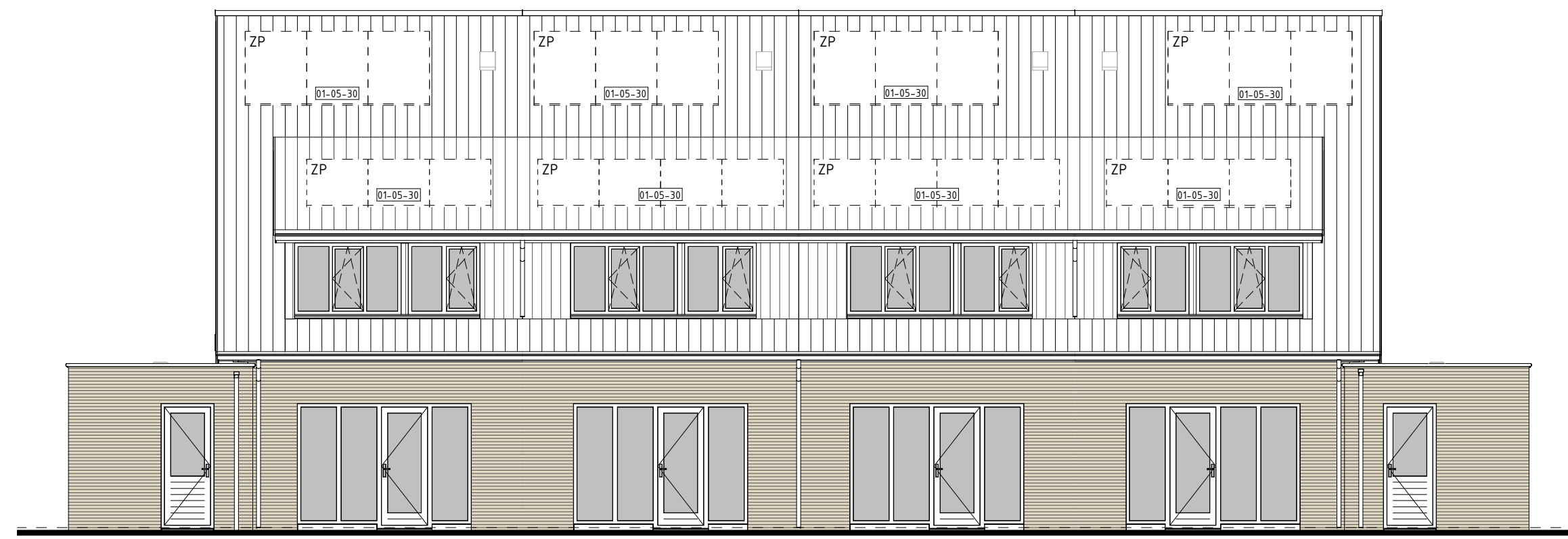
type S2 bwnr get.:05 type T1 bwnr get.:04 type T1 bwnr get.:03 type S1sp bwnr get.:02 ACHTERGEVEL 1:50
