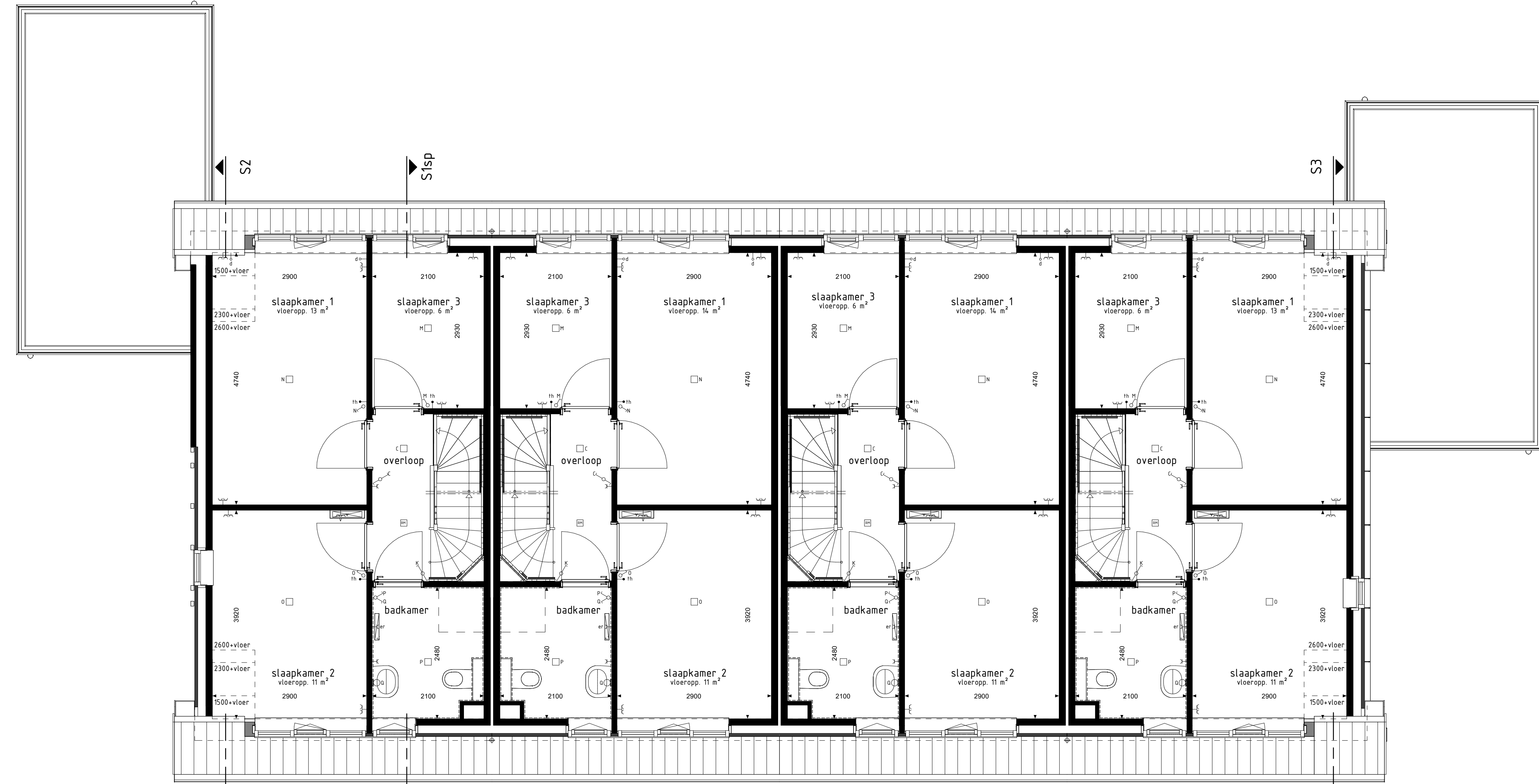
type S1sp bwnr get.:02 1e VERDIEPING 1:50
