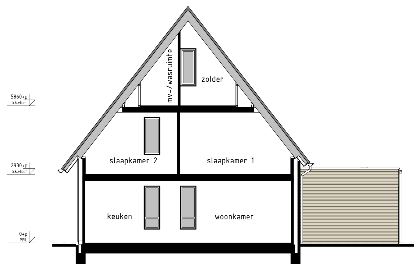
type S1sp bwnr get.:02 DOORSNEDE S2-S2 1:50
