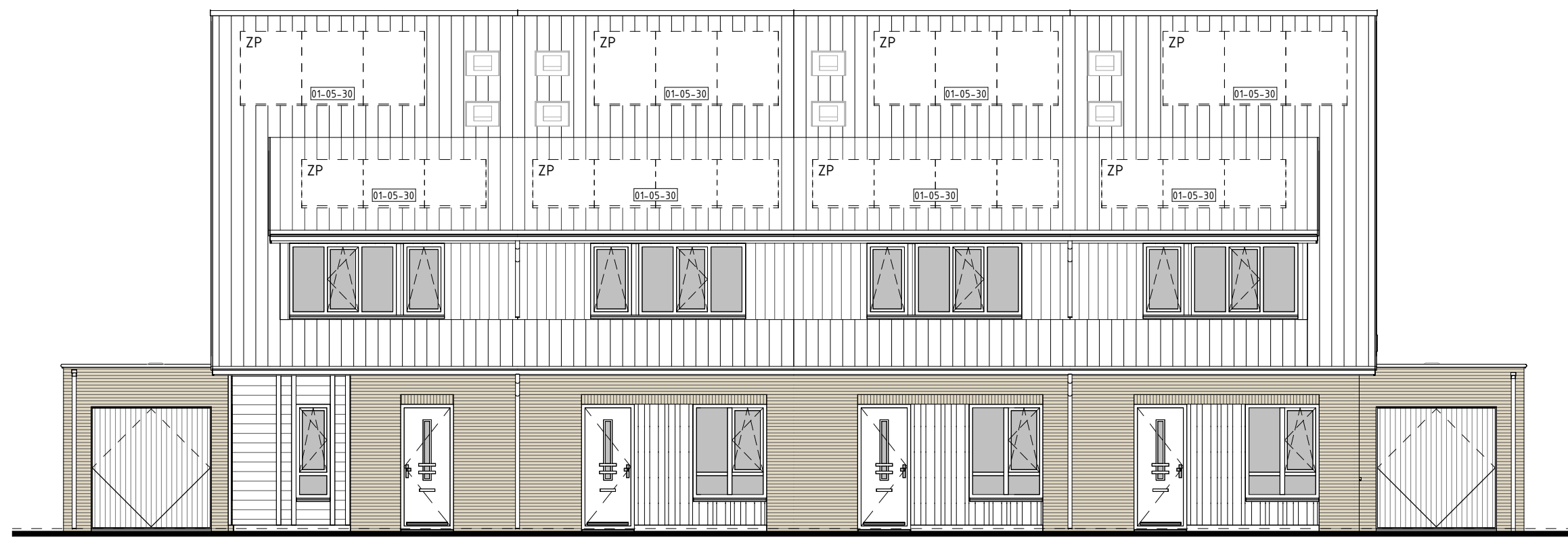
type S1sp bwnr get.:02 VOORGEVEL 1:50
