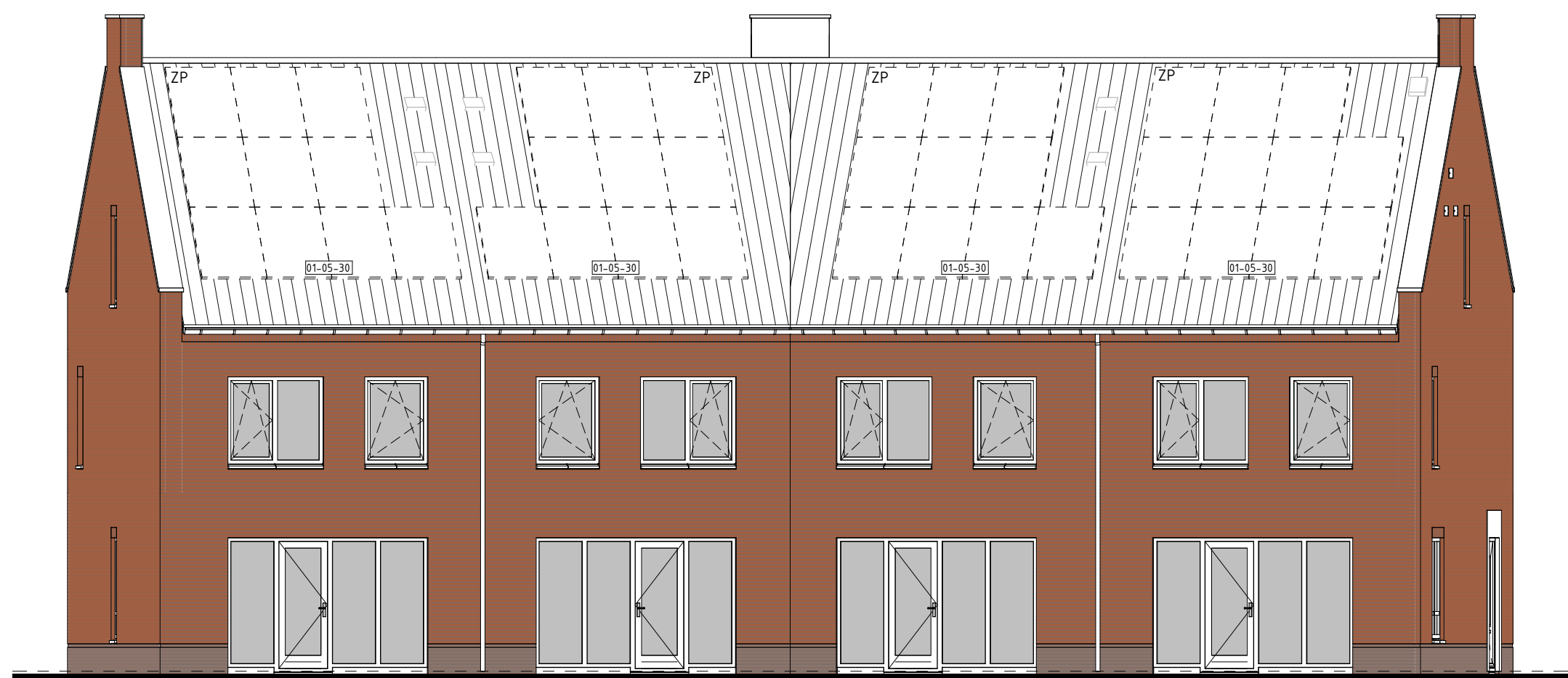
type E3 bwnr get.:17 type H1sp bwnr get.:16 type H1 bwnr get.:15 type I1 bwnr get.:14 ACHTERGEVEL
