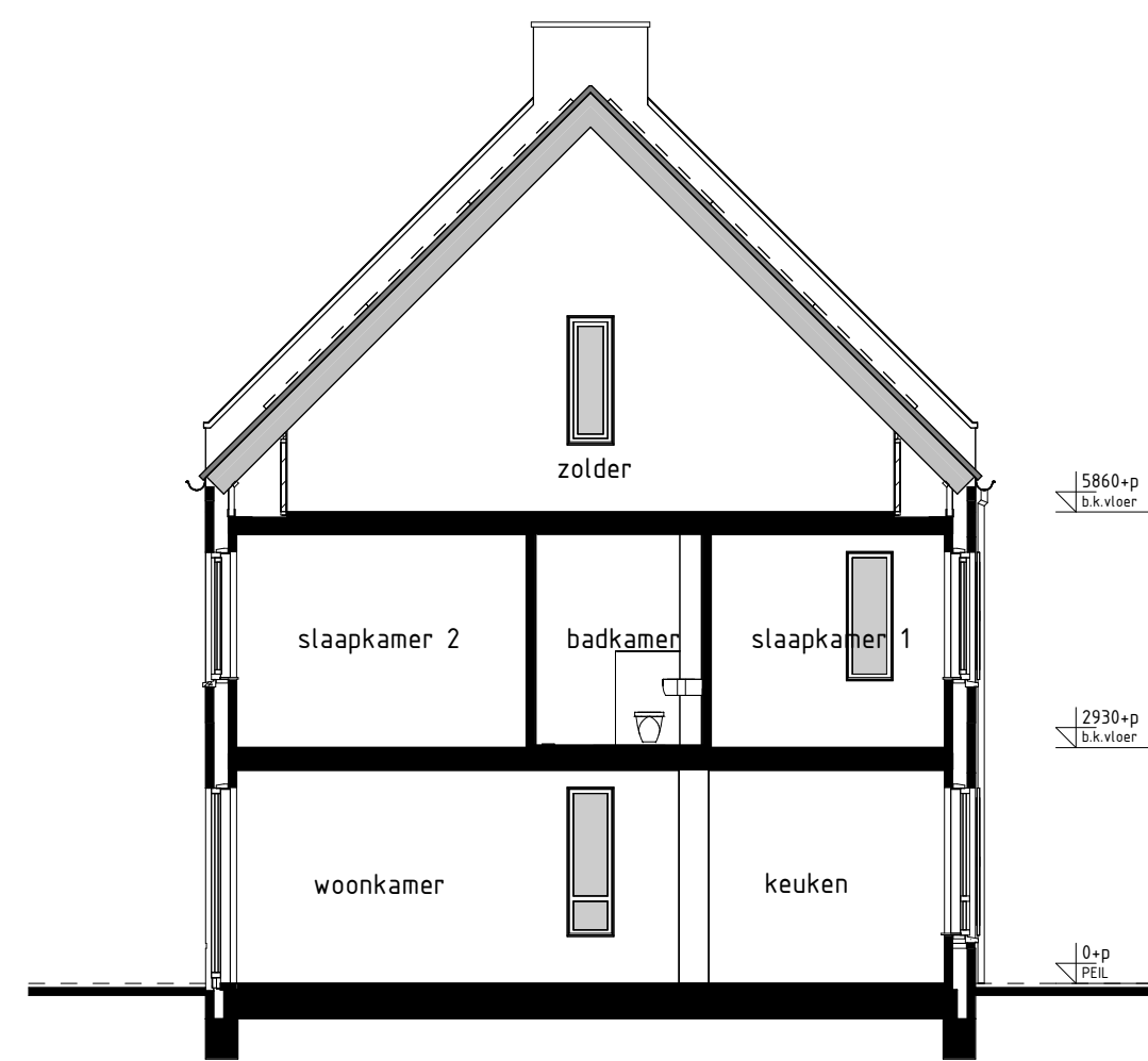
type E3 bwnr get.:17 DOORSNEDE E3-E3
