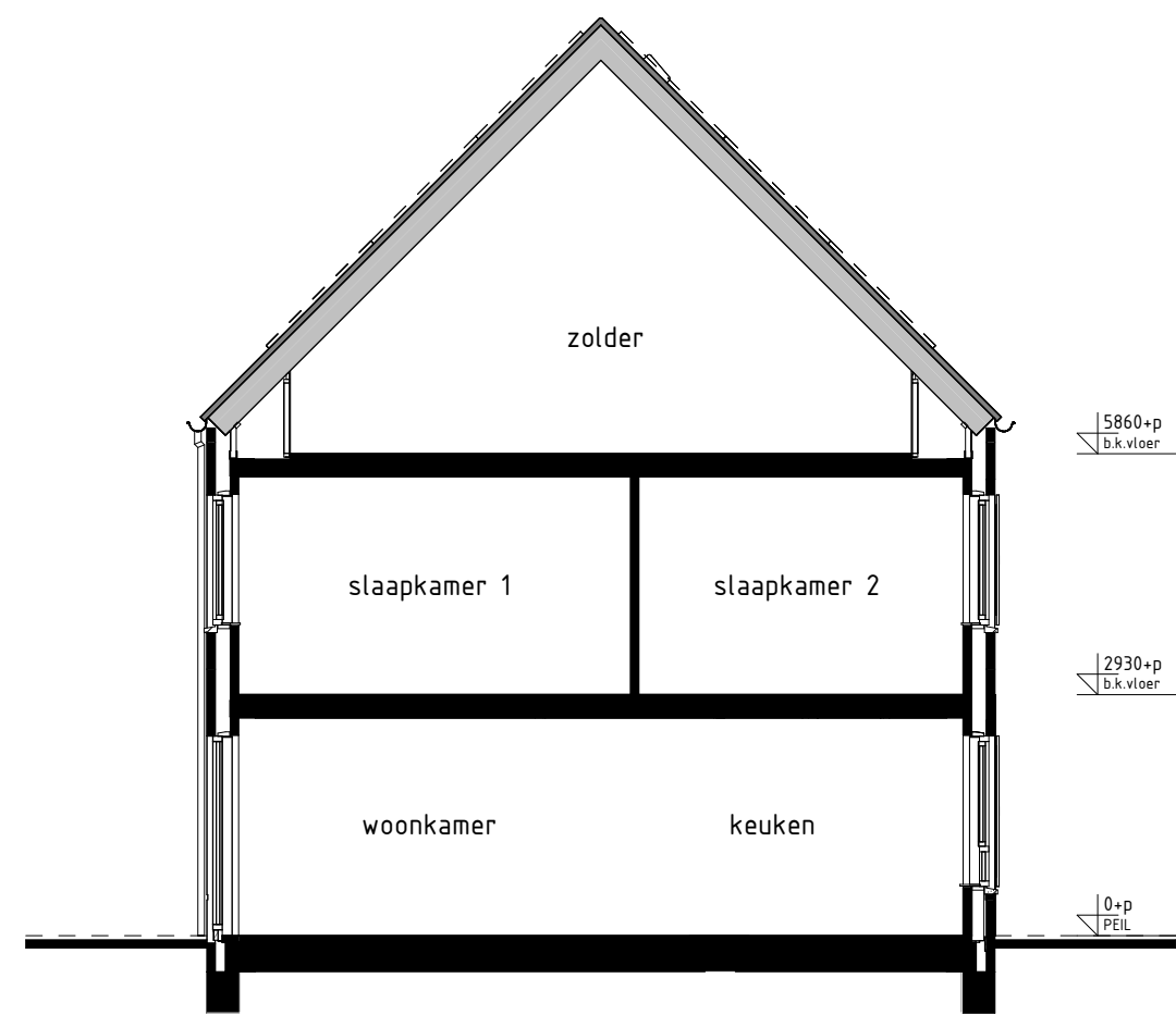
type I1 bwnr get.:14 DOORSNEDE I1-I1
