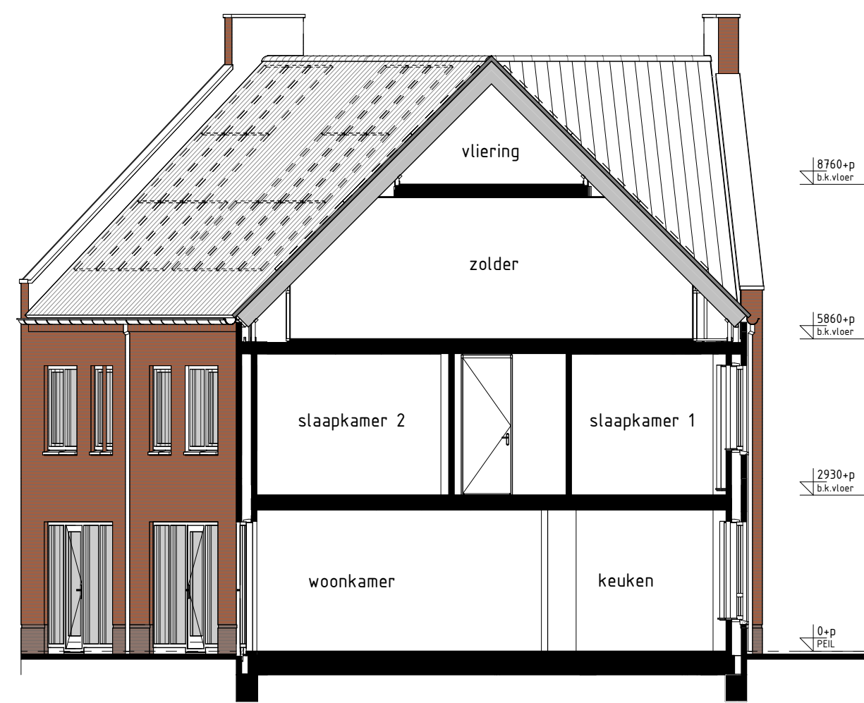
type H1 & H1sp bwnr get.:15 bwnr gesp.:16 DOORSNEDE H1-H1
