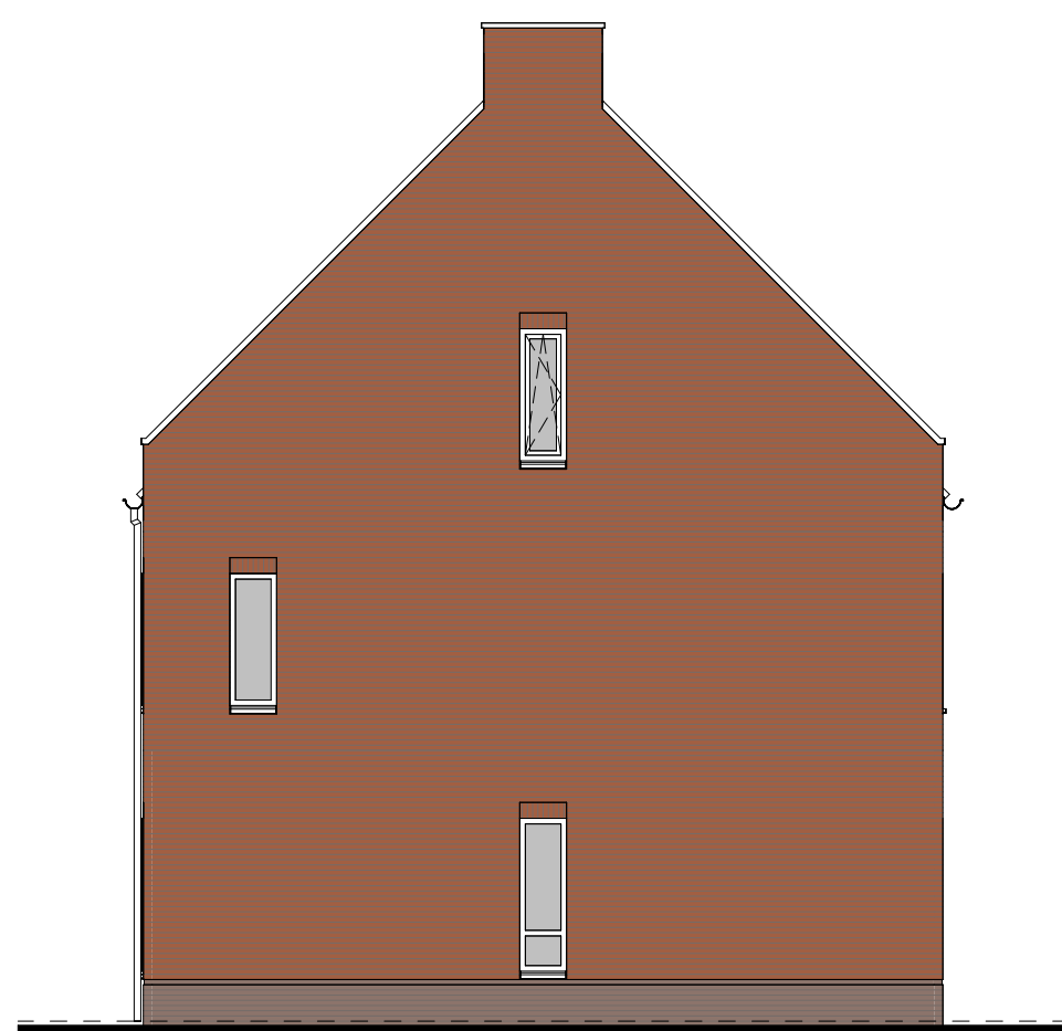
type E3 bwnr get.:17 RECHTERGEVEL
