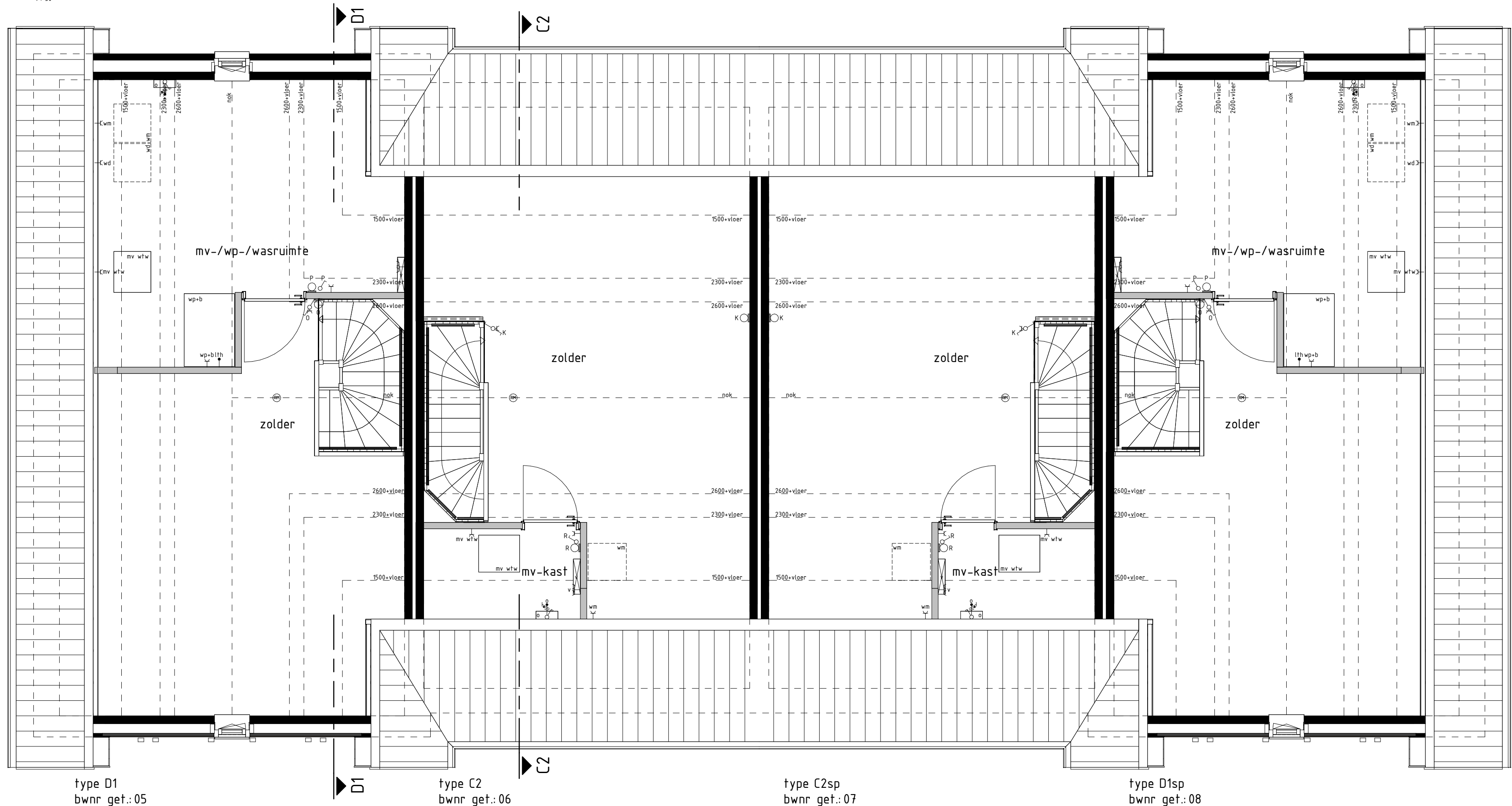
2e VERDIEPING
