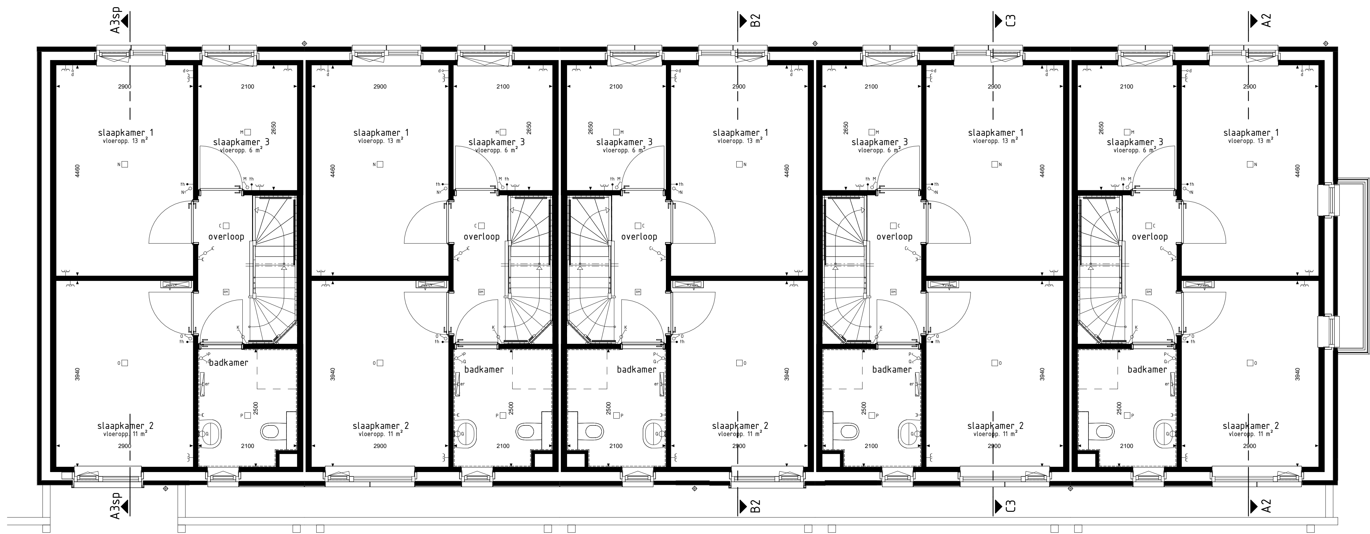
type A3sp bwnr get.:80 type C3sp bwnr get.:81 type B2 bwnr get.:82 type C3 bwnr get.:83 type A2 bwnr get.:84 1E VERDIEPING 1:50
