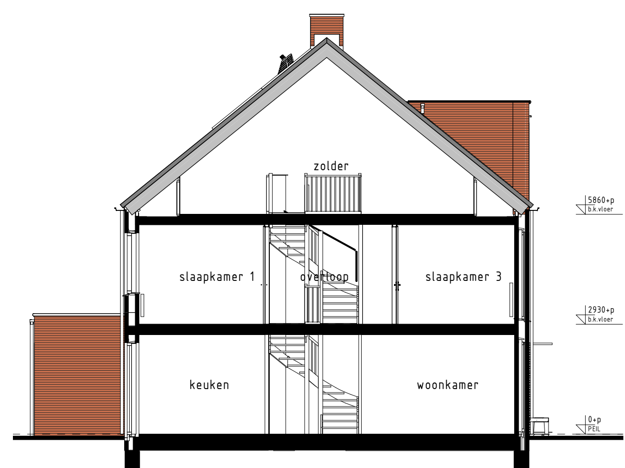
type E3sp, E6 bwnr get.:414 bwnr gesp.:416 DOORSNEDE E3-E3 1.00
