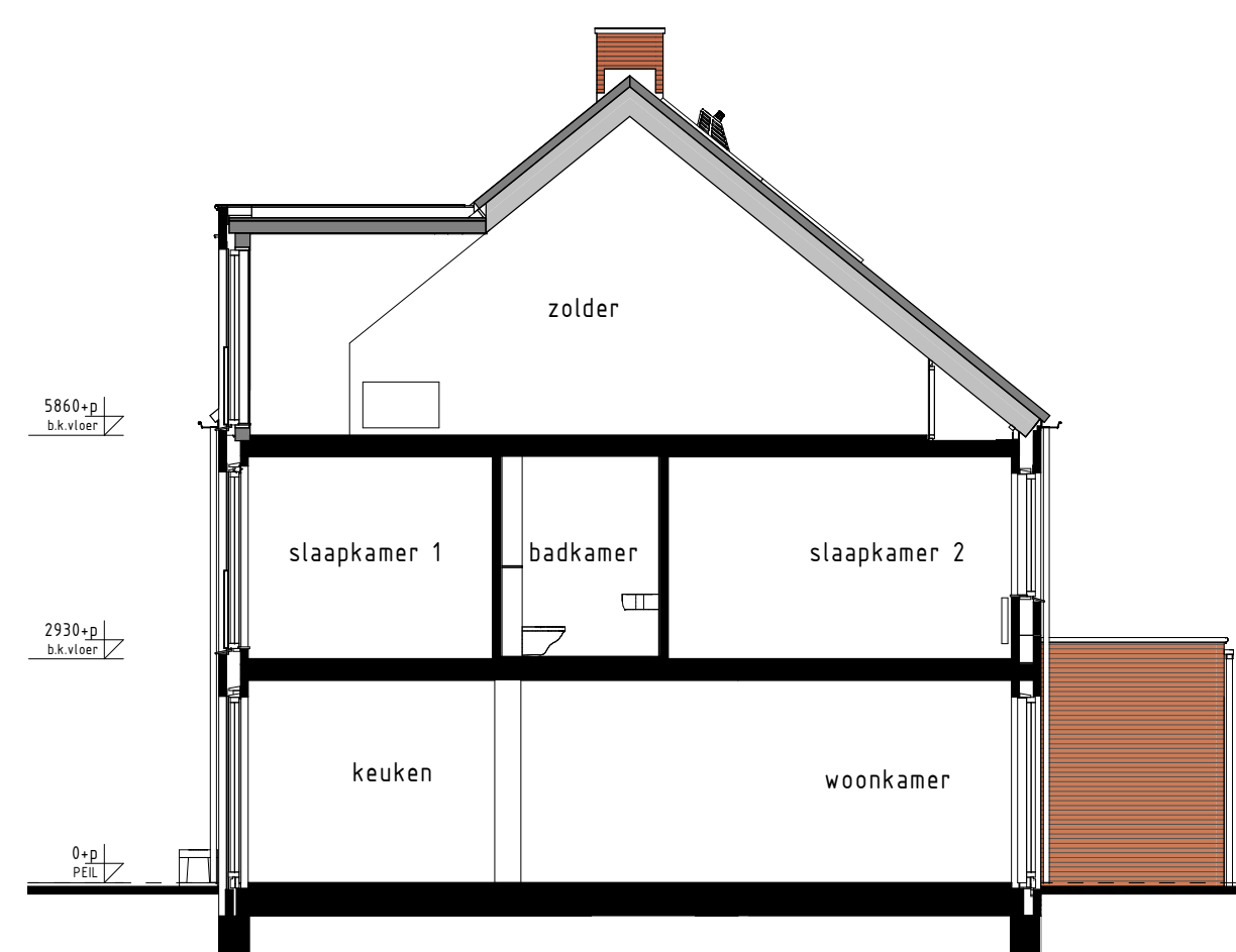
type E1sp bwnr get.:415 DOORSNEDE E1-E1 1.00
