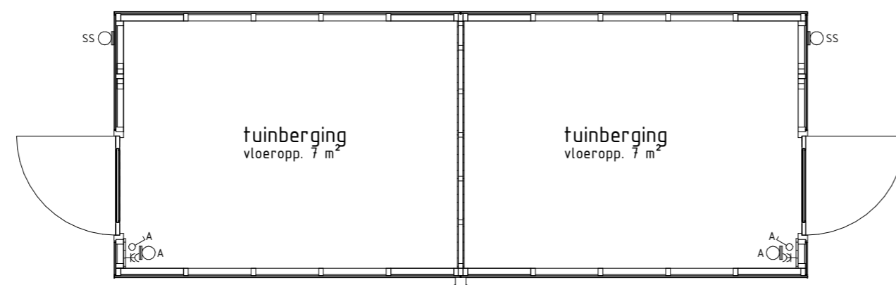
PLATTEGROND 1:50 bwnr get.: 214,221 bwnr get.: 215,222
