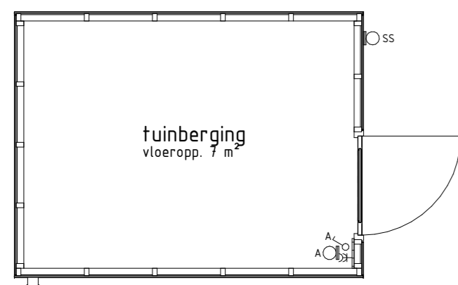
PLATTEGROND 1:50 bwnr get.: 223
