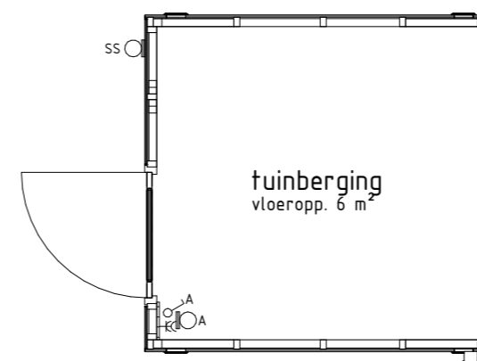
PLATTEGROND 1:50 bwnr get.: 242
