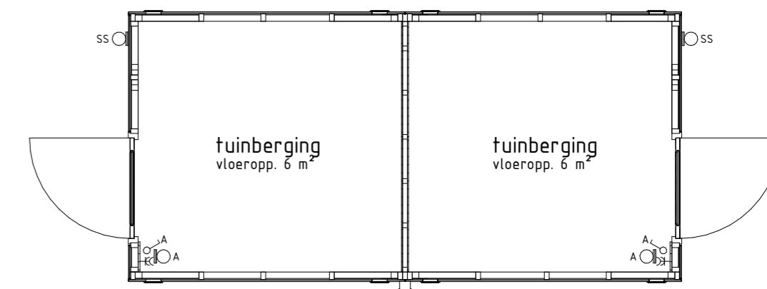
PLATTEGROND 1:50 bwnr get.: 234,236,238,240,243 bwnr get.: 235,237,239,241,244
