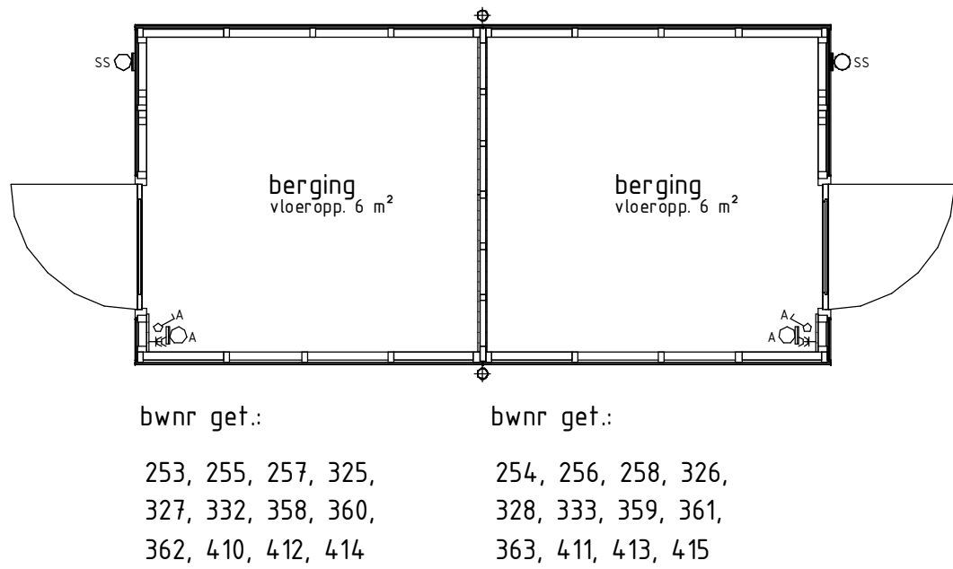
PLATTEGROND 1 : 50
