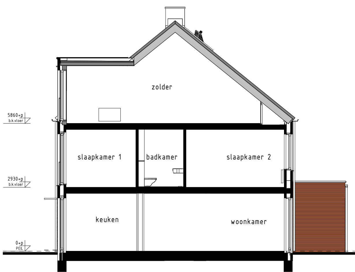
type E1, E1sp bwnr get.:317, 318 DOORSNEDE E1-E1
