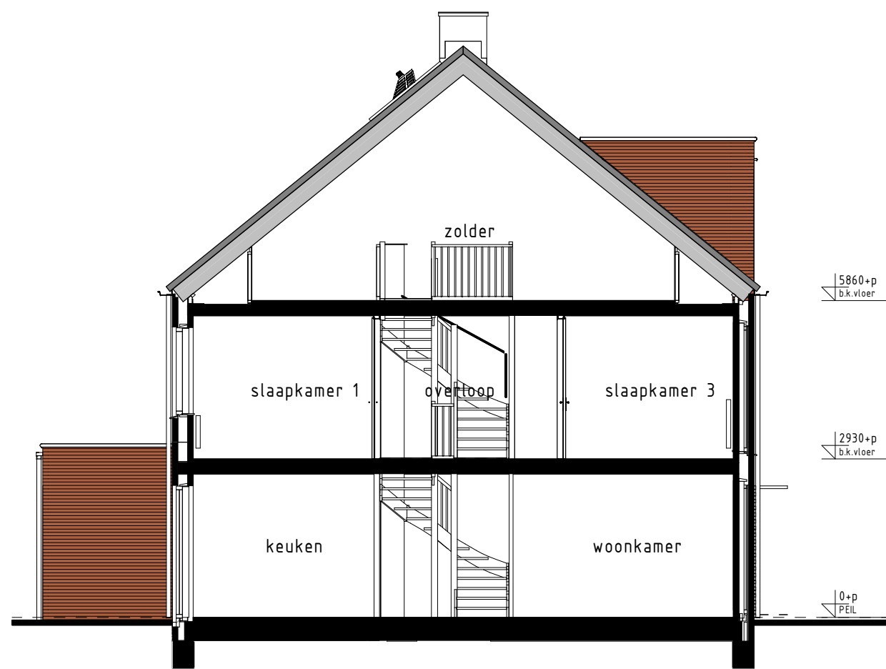
type D1, D1sp bwnr get.:316, 319 DOORSNEDE E3-E3
