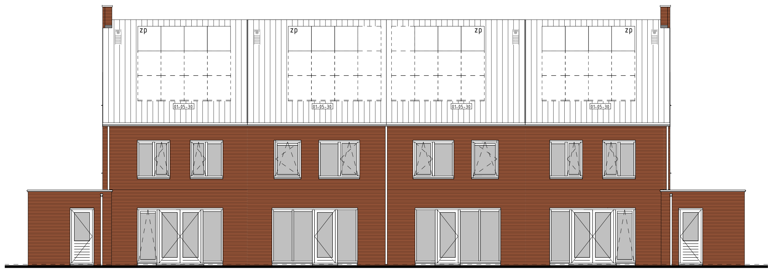
type D1sp bwnr get.:319 type E1sp bwnr get.:318 type E1 bwnr get.:317 type D1 bwnr get.:316 ACHTERGEVEL
