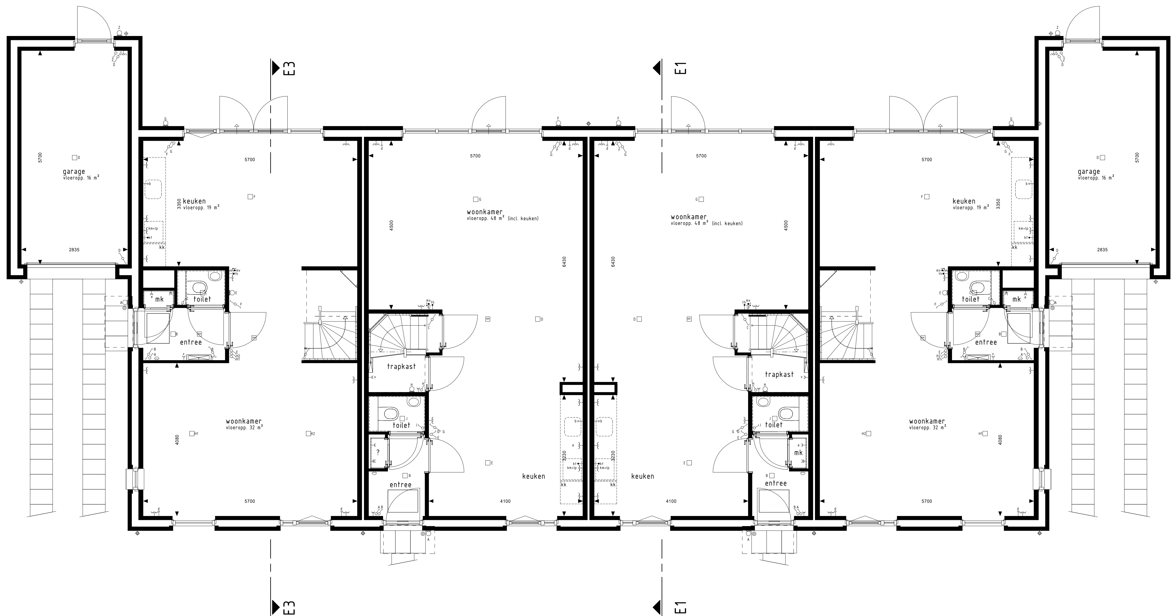
type D1 bwnr get.:316 type E1 bwnr get.:317 type E1sp bwnr get.:318 type D1sp bwnr get.:319 BEGANE GROND
