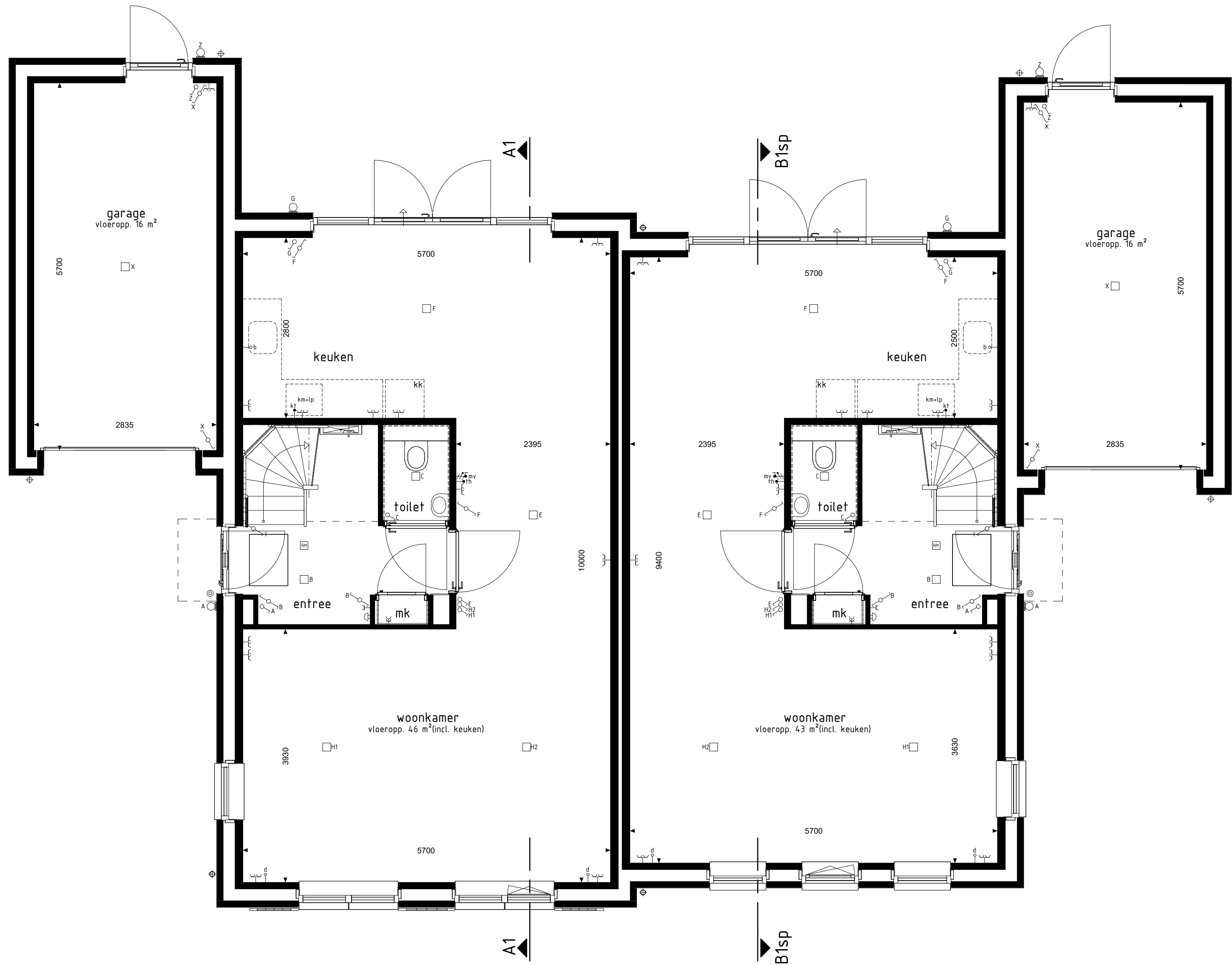
type A1 bwnr get.:1 BEGANE GROND
