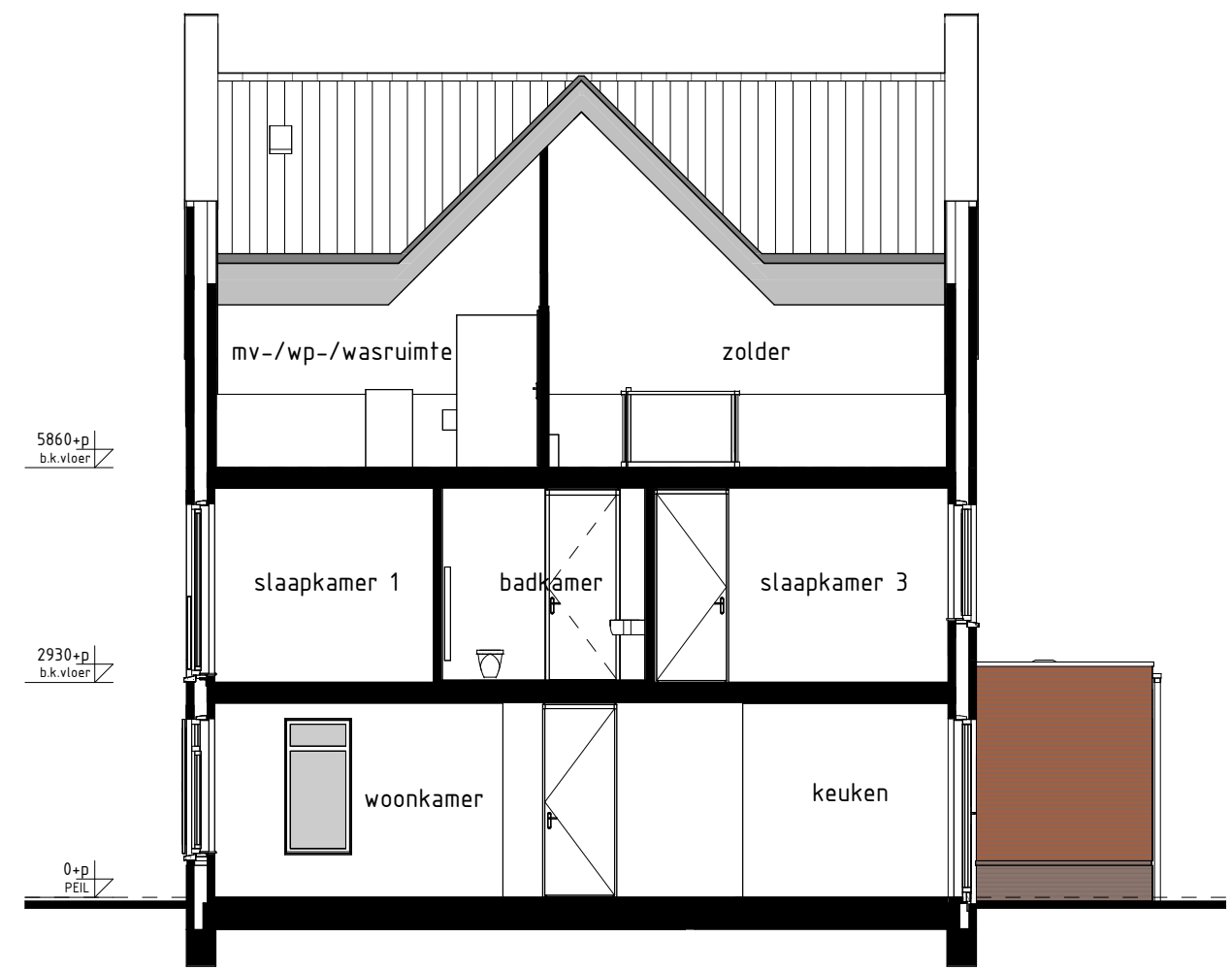
type A1 bwnr get.:1 DOORSNEDE A1-A1
