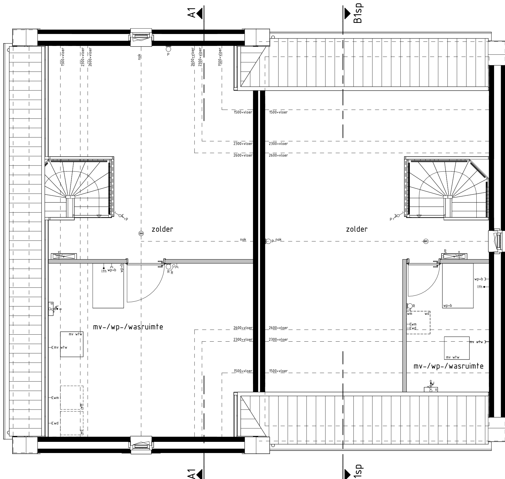
type A1 bwnr get.:1 2e VERDIEPING
