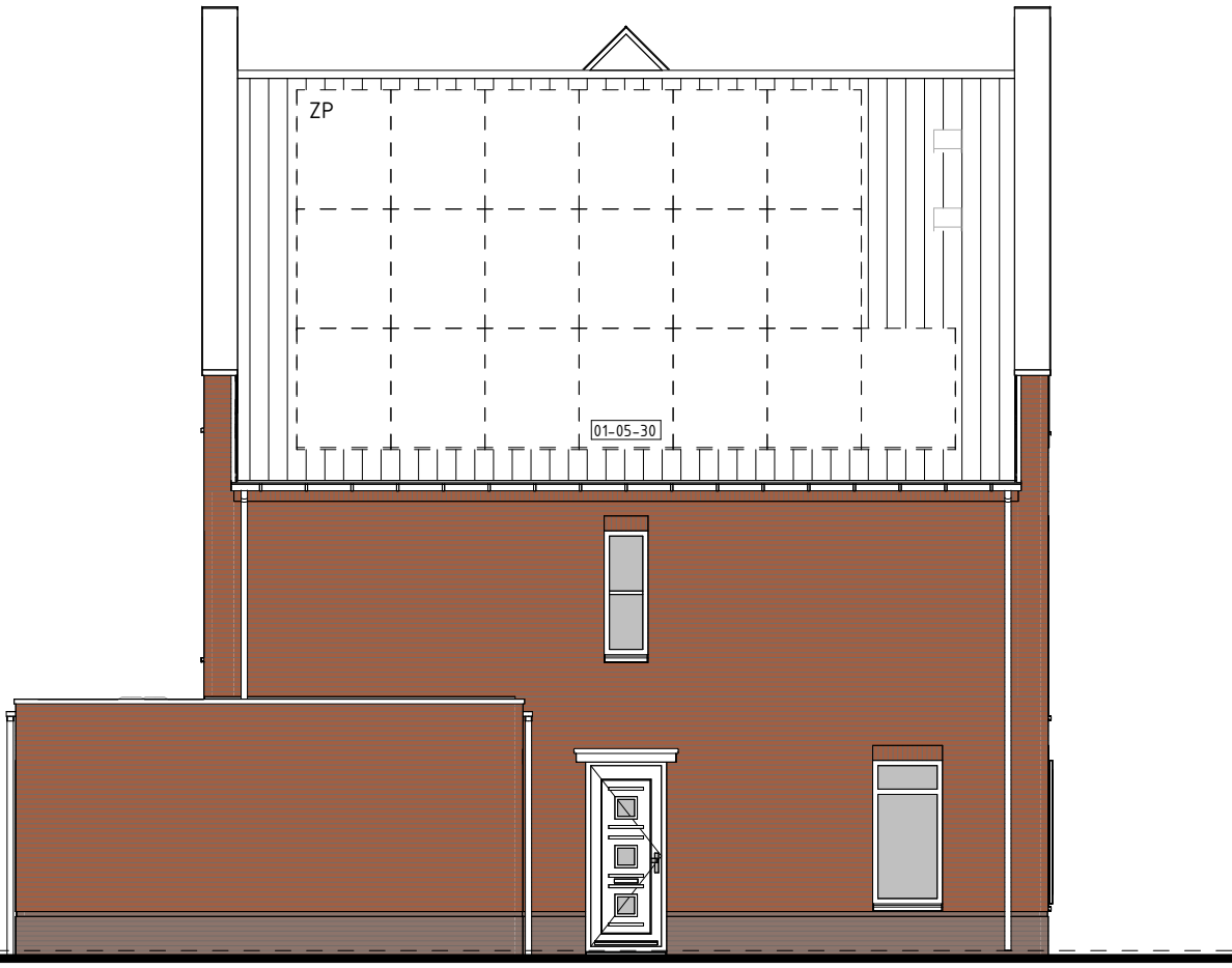
type A1 bwnr get.:1 LINKERGEVEL
