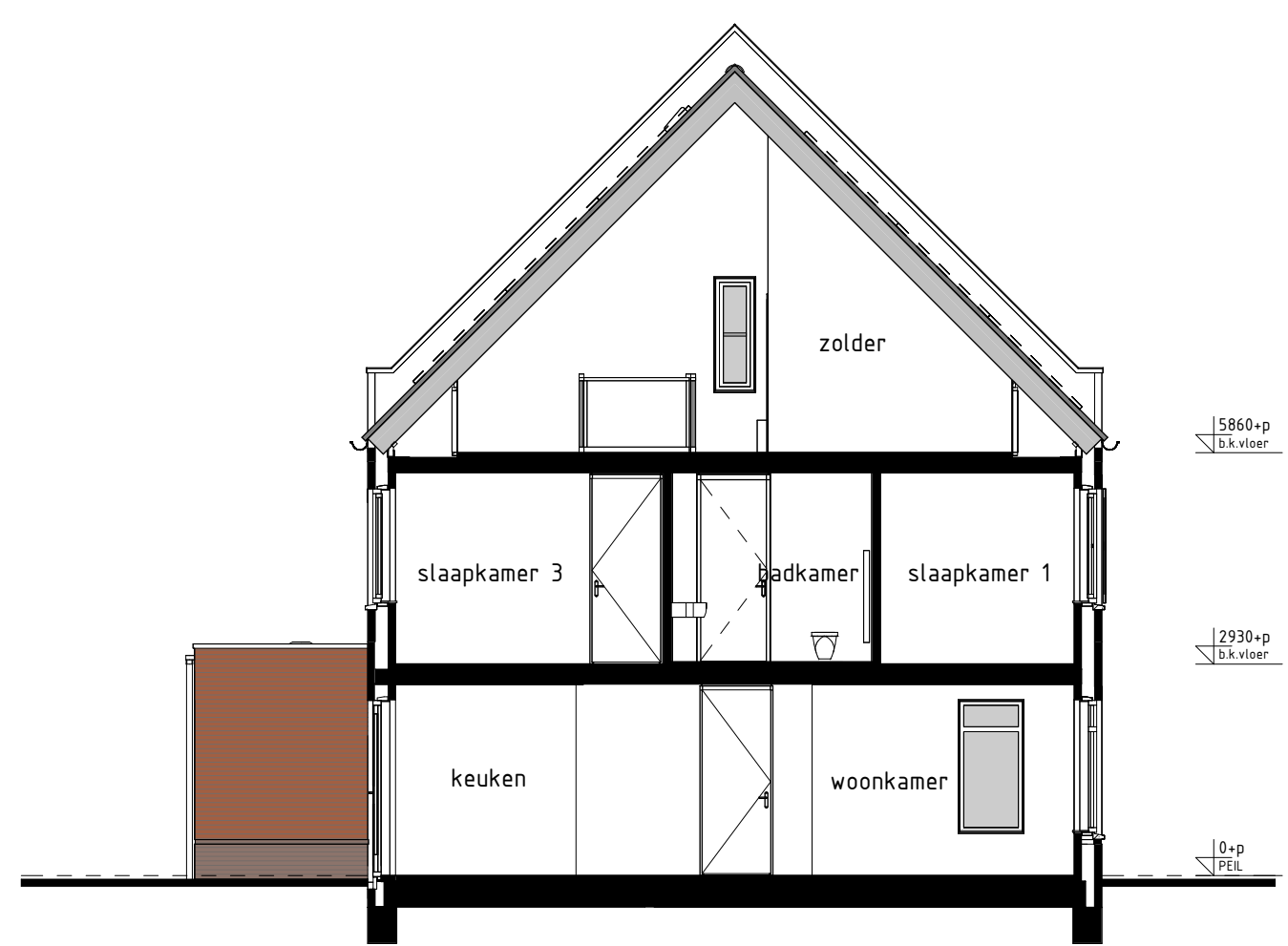
type B1sp bwnr get.:2 DOORSNEDE B1sp-B1sp
