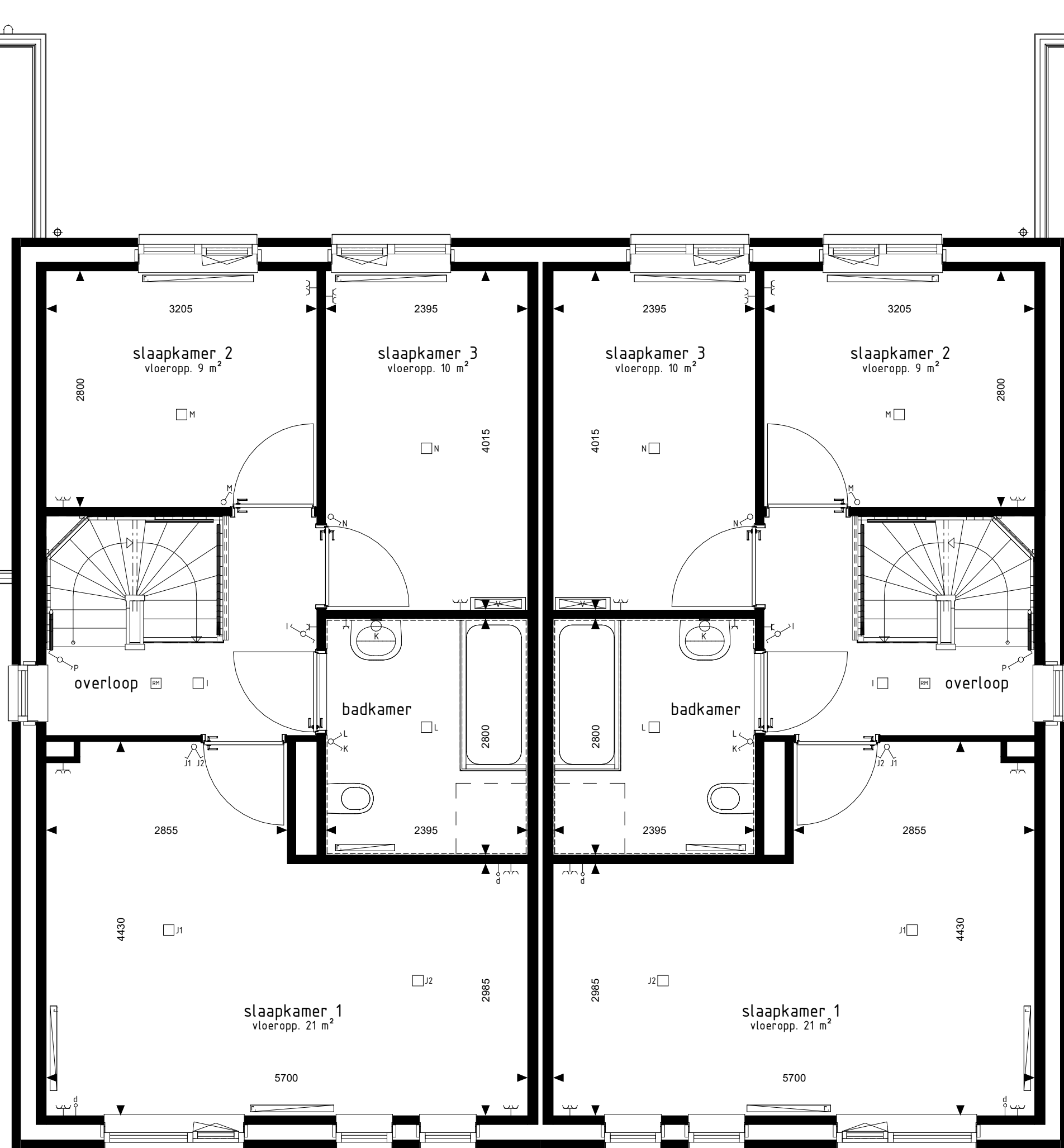
type B2 bwnr get.: 11 type B2sp bwnr get.: 12
