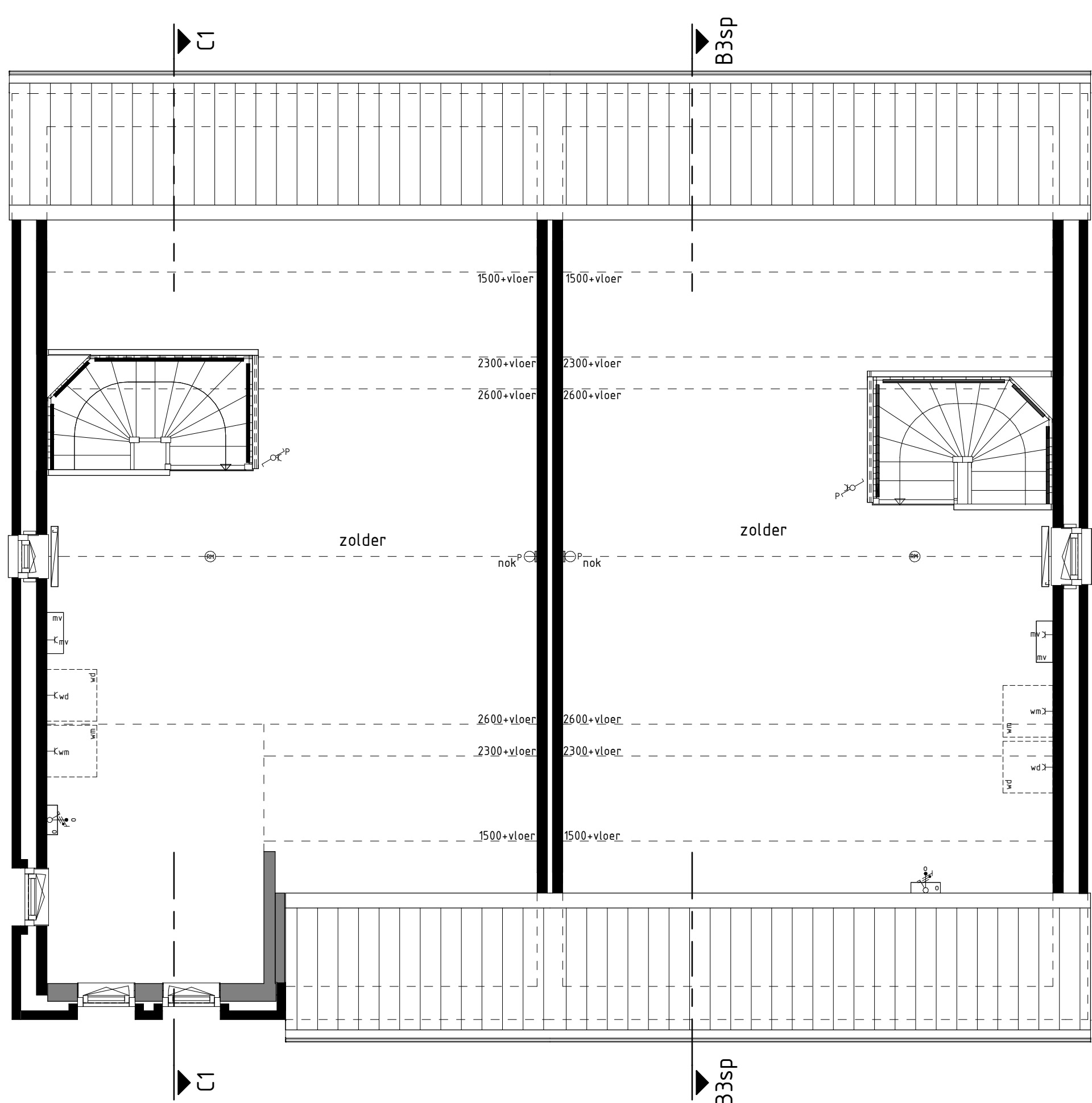
type C1 bwnr get.: 9 type B3sp bwnr get.: 10 2e VERDIEPING
