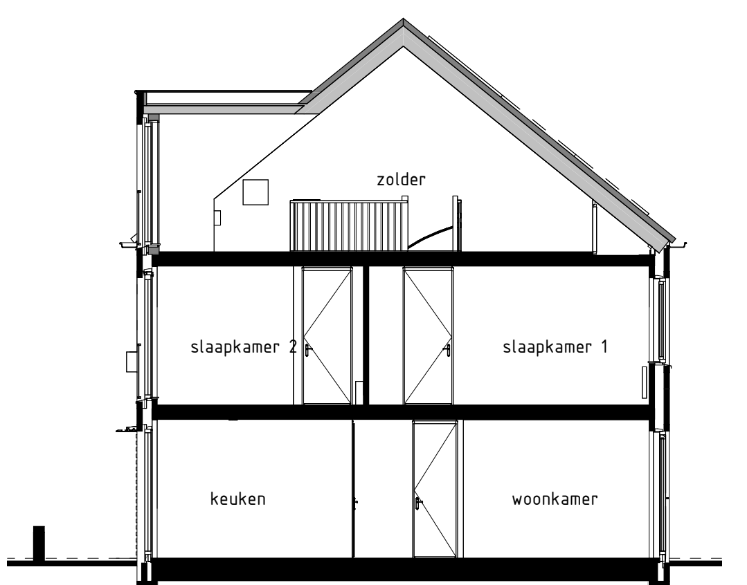
type B3 bwnr get.:549 DOORSNEDE B3-B3 1:50
