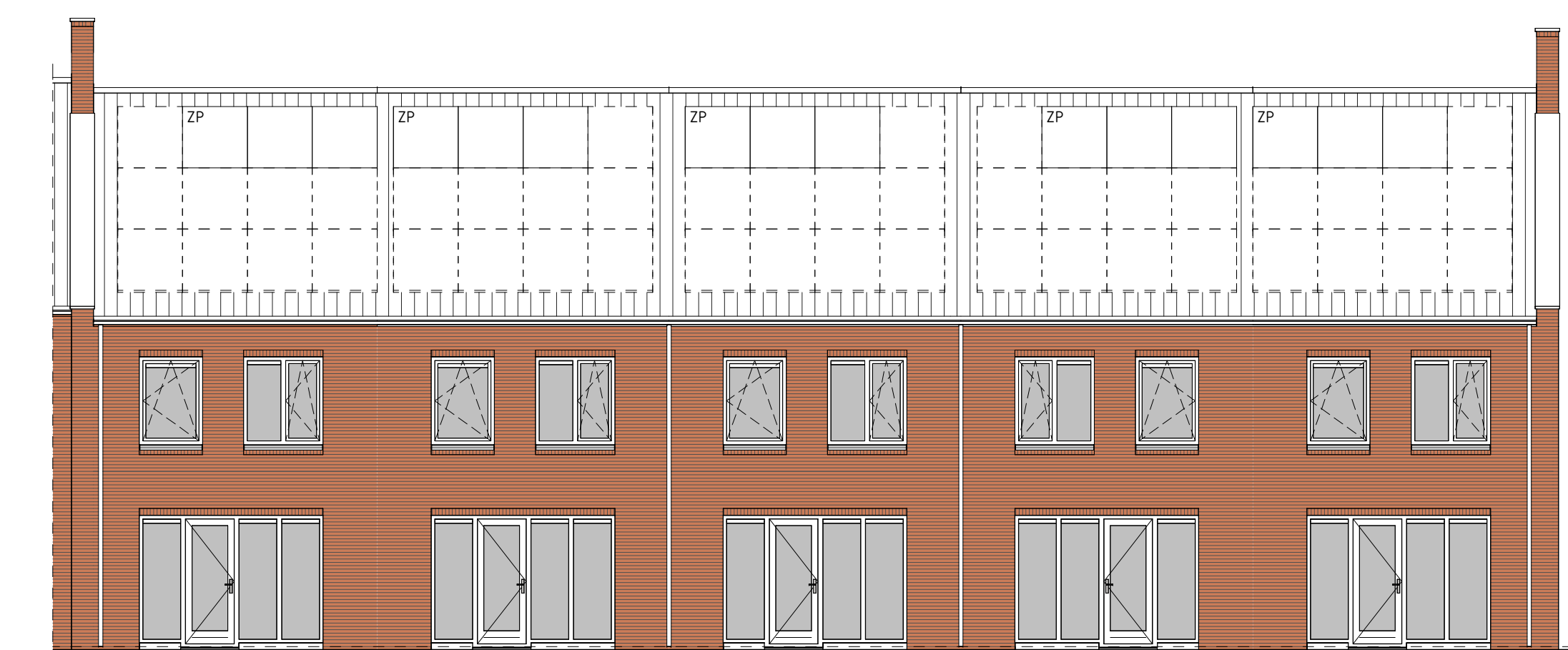
type B4sp bwnr get.:552 type B4sp bwnr get.:551 type B4sp bwnr get.:550 type B3 bwnr get.:549 type A1sp bwnr get.:548 ACHTERGEVEL 1:50
