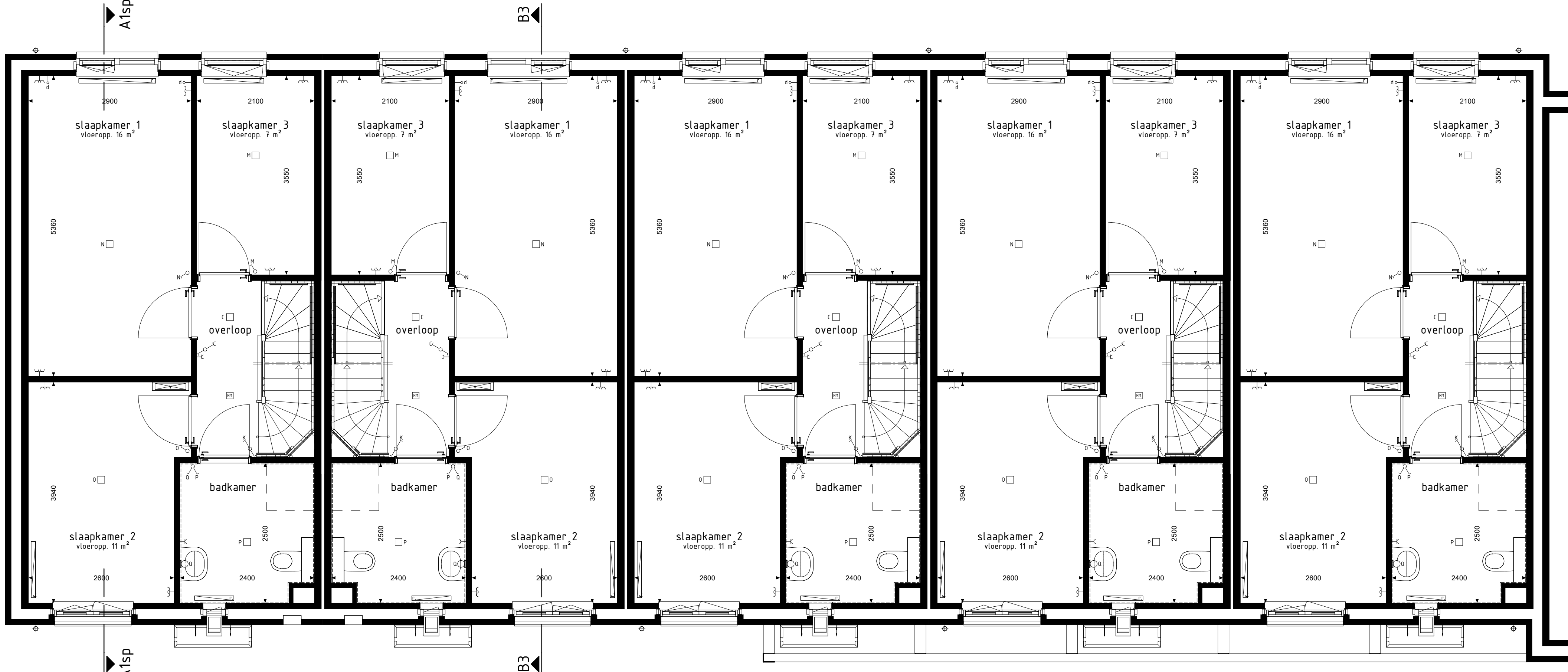
type A1sp bwnr get.:548 type B3 bwnr get.:549 type B4sp bwnr get.:550 type B4sp bwnr get.:551 type B4sp bwnr get.:552 1e VERDIEPING 1:50
