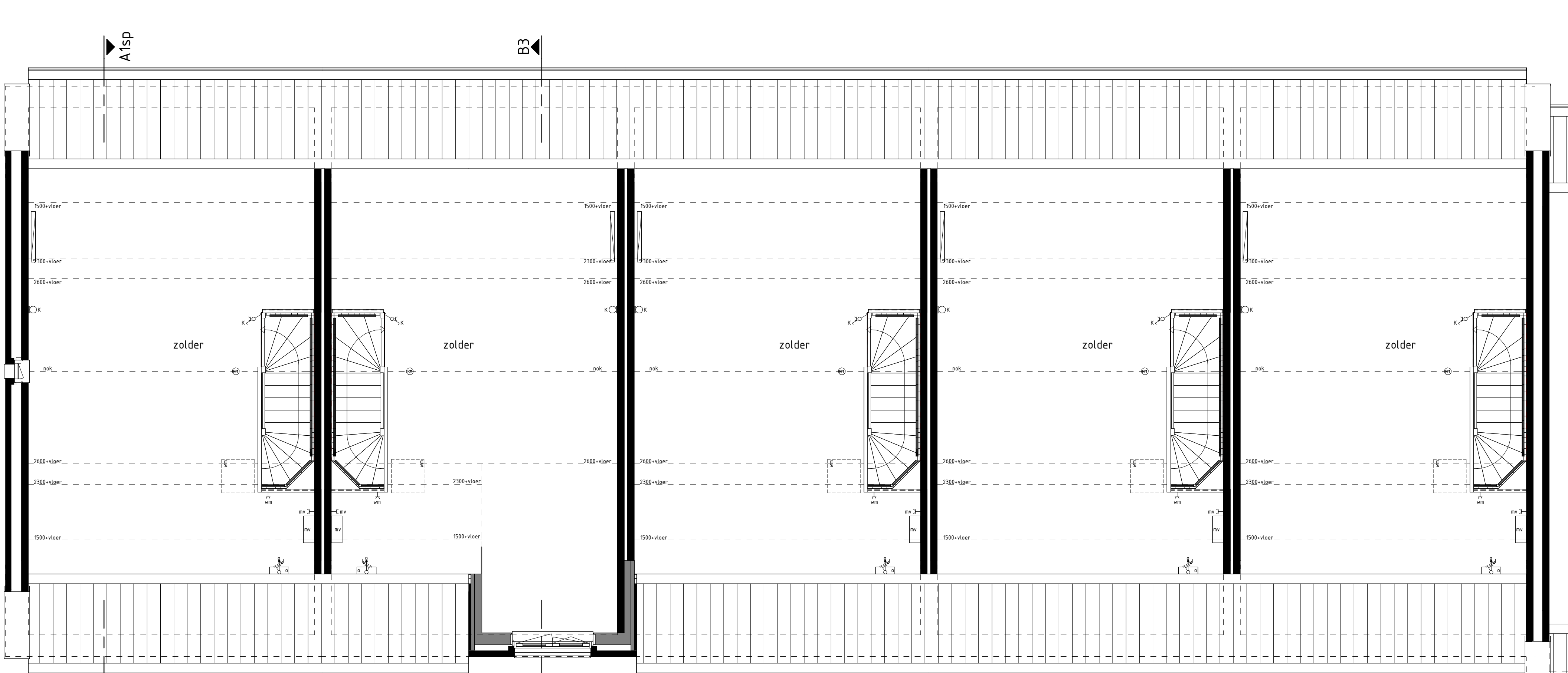
type A1sp bwnr get.:548 type B3 bwnr get.:549 type B4sp bwnr get.:550 type B4sp bwnr get.:551 type B4sp bwnr get.:552 2e VERDIEPING 1:50
