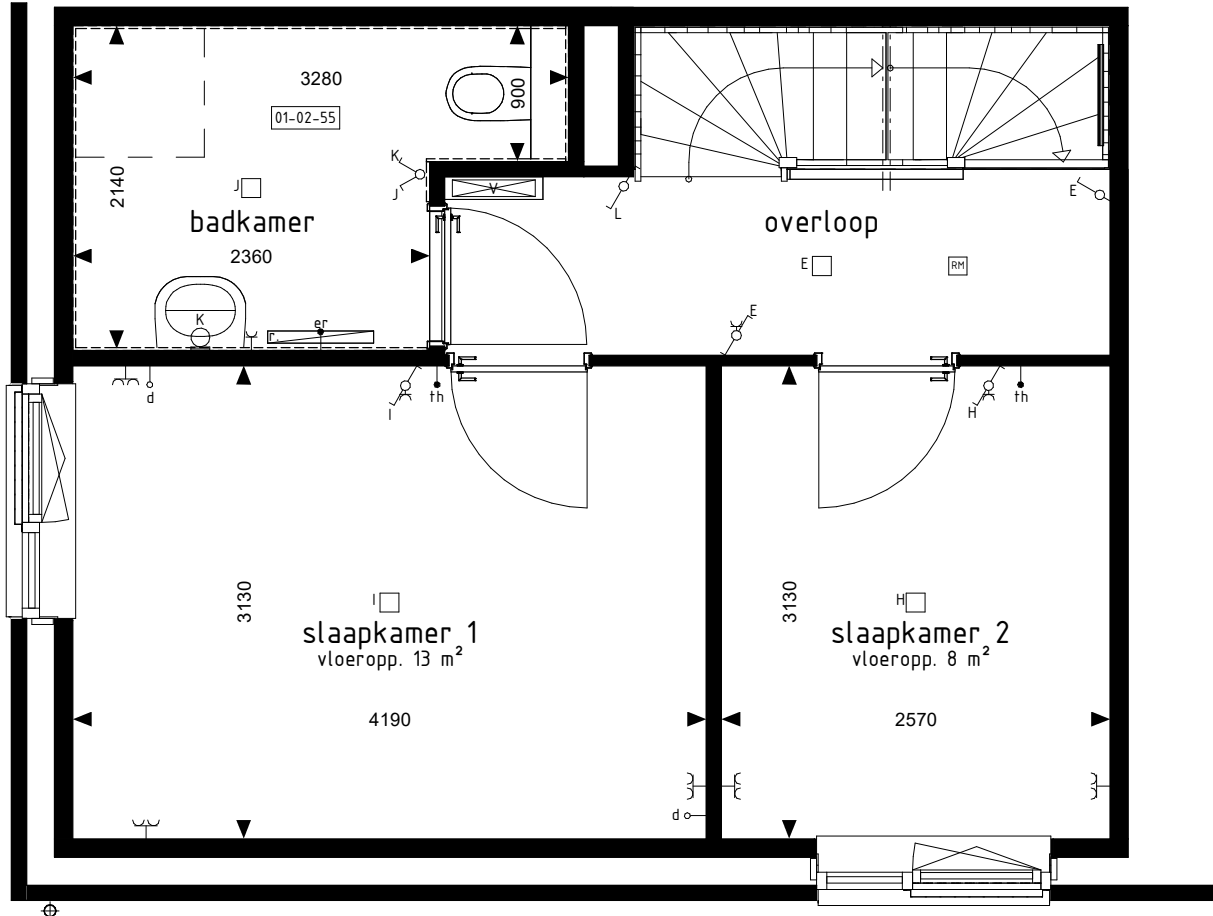
1e VERDIEPING 1:50
