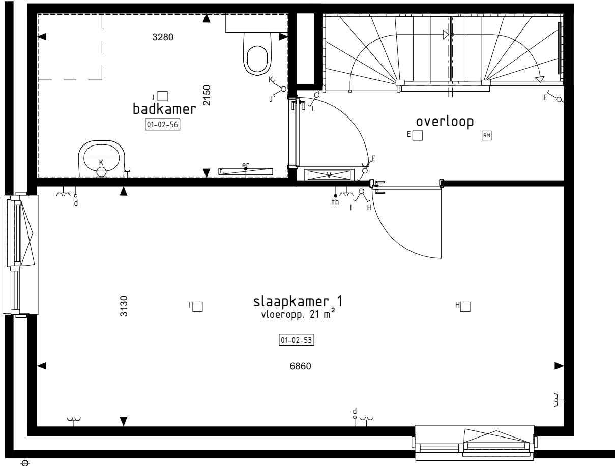
1e VERDIEPING 1:50
