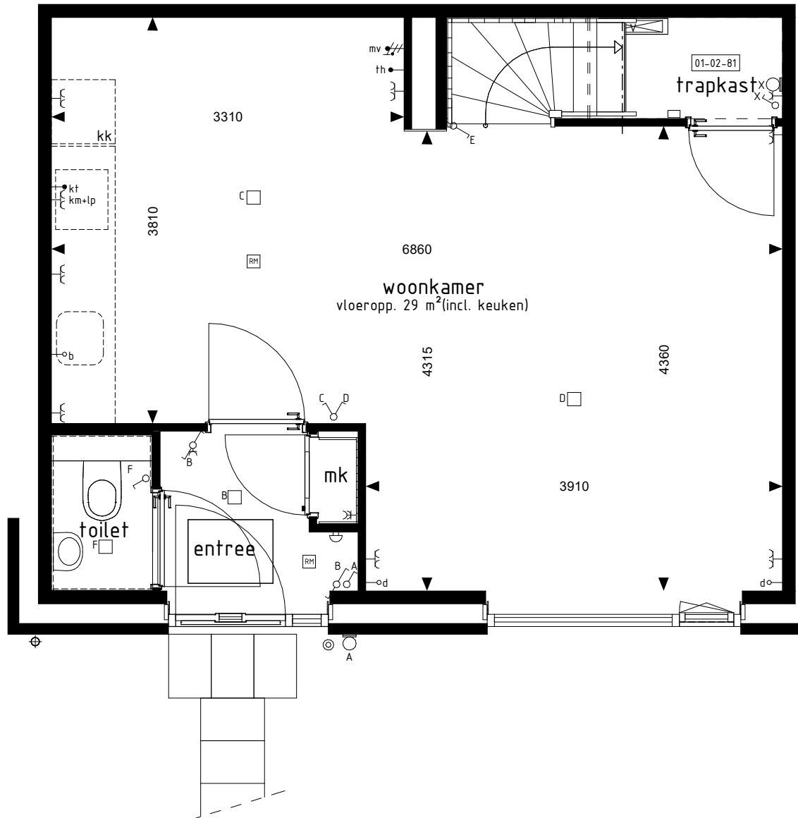
BEGANE GROND 1:50
