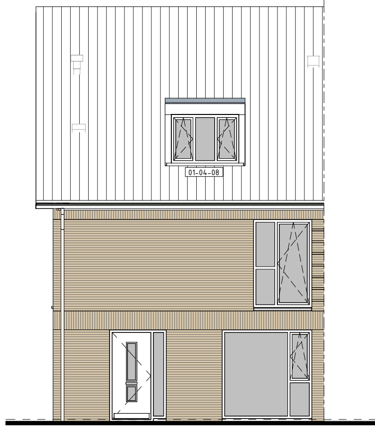
VOORGEVEL 1:100
