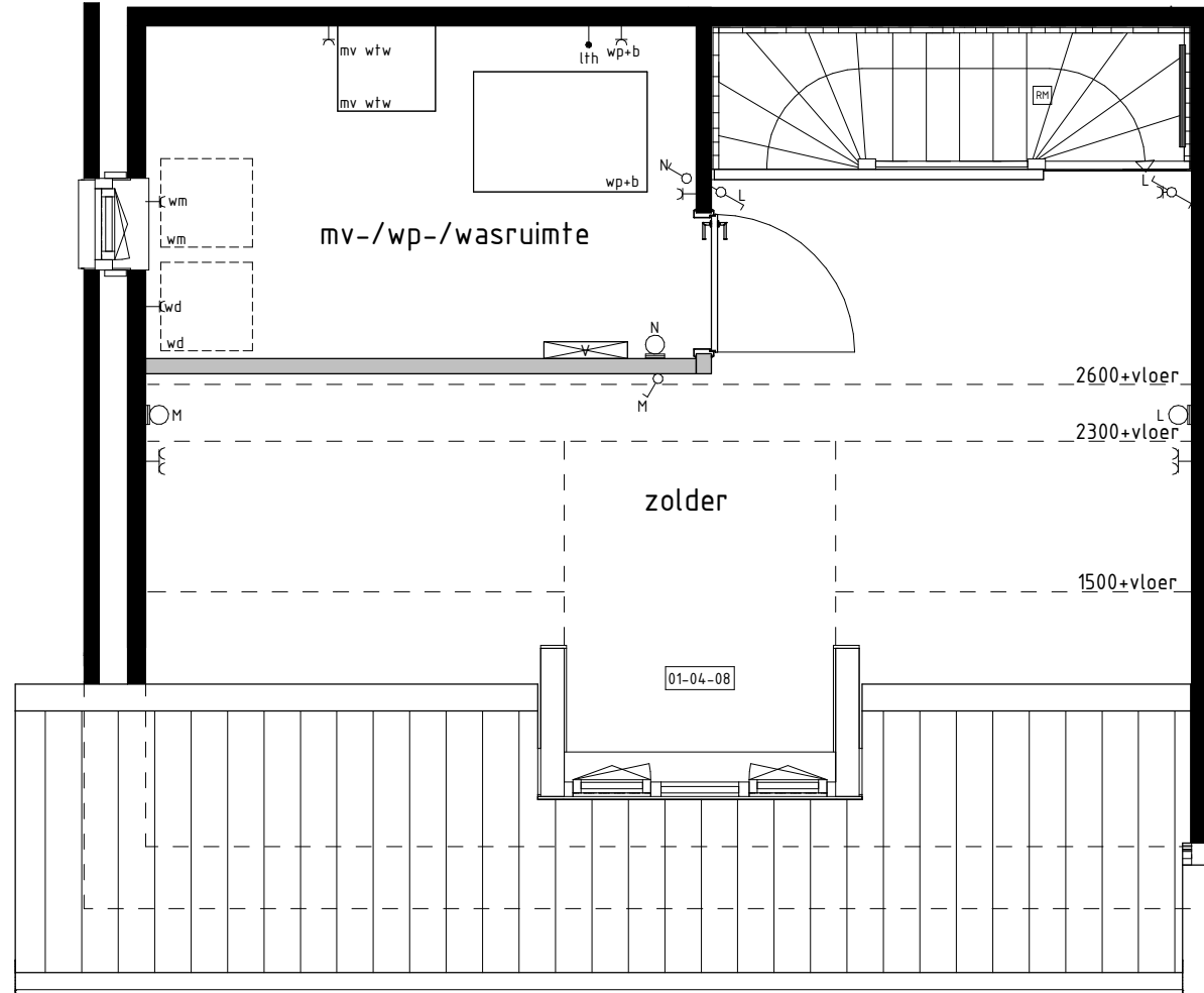
2e VERDIEPING 1:50
