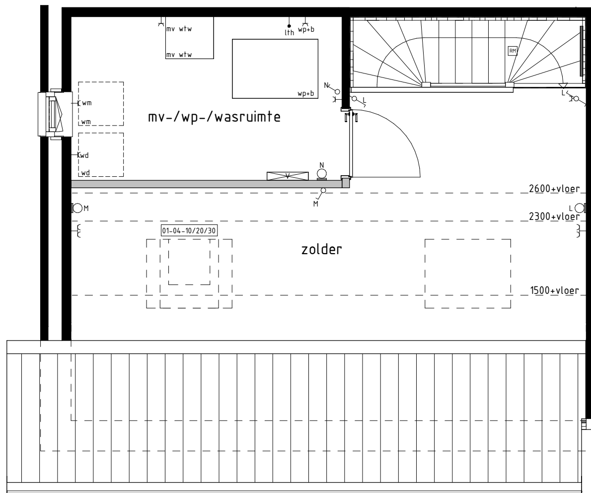
2e VERDIEPING 1:50
