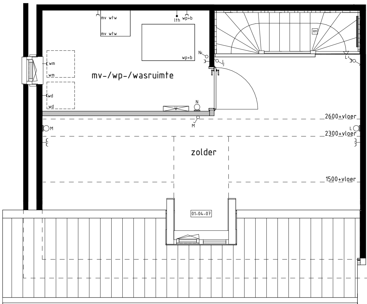
2e VERDIEPING 1:50
