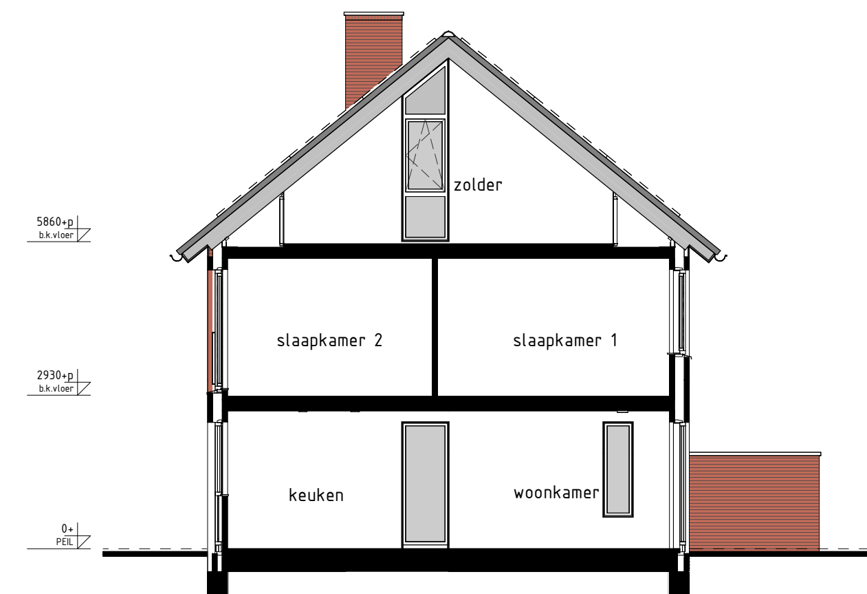
type J1sp bwnr get.: 79, 89 en 99 DOORSNEDE J1sp-J1sp
