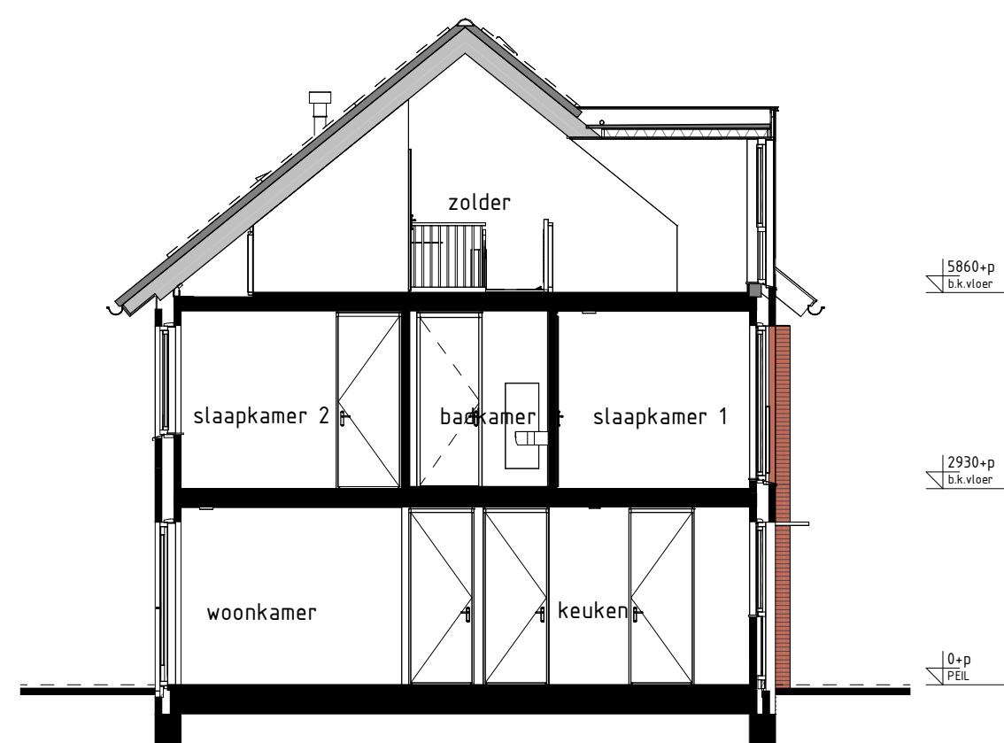
type I1sp bwnr get.: 80, 90 en 100 DOORSNEDE I1sp-I1sp
