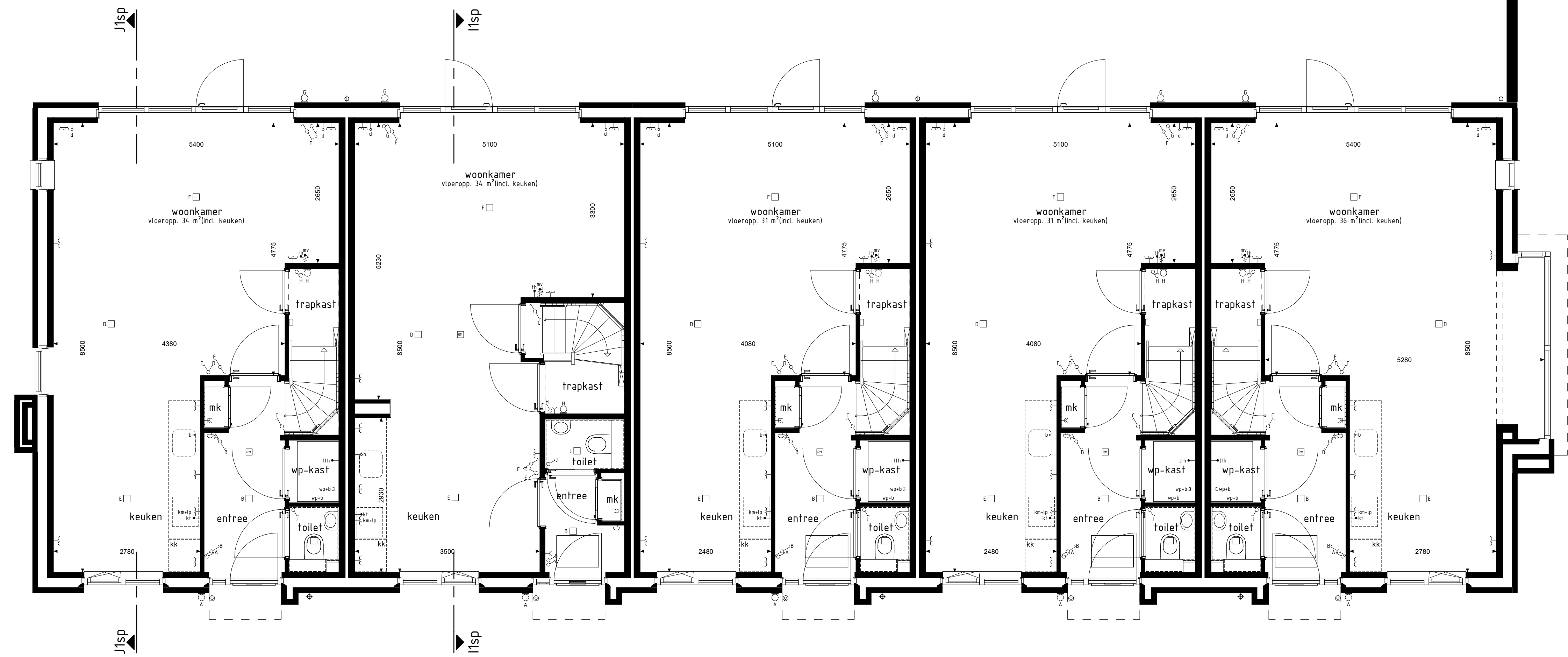
type J1sp bwnr get.: 79, 89 en 99 type I1sp bwnr get.: 80, 90 en 100 type H1sp bwnr get.: 81, 91 en 101 type H1sp bwnr get.: 82, 92 en 102 type J2 bwnr get.: 83, 93 en 103 BEGANE GROND
