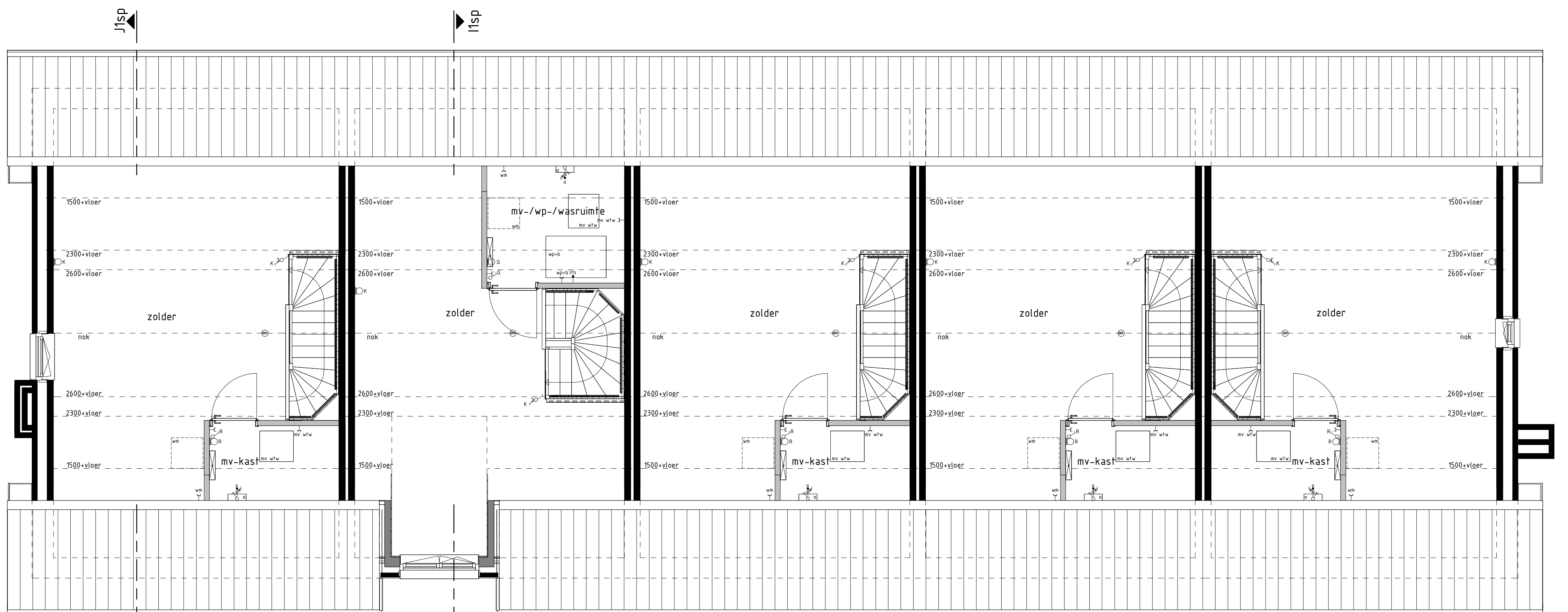
type J1sp bwnr get.: 79, 89 en 99 type I1sp bwnr get.: 80, 90 en 100 type H1sp bwnr get.: 81, 91 en 101 type H1sp bwnr get.: 82, 92 en 102 type J2 bwnr get.: 83, 93 en 103 2e VERDIEPING
