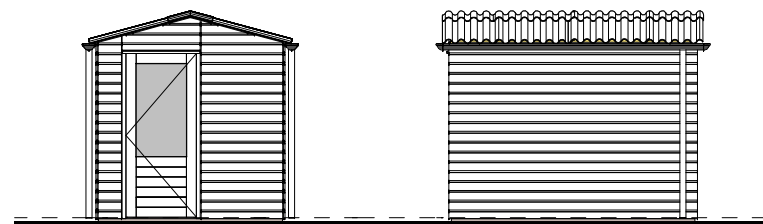
ZIJGEVEL 1 : 100 bwnr get.: 12, 16, 175 bwnr gesp.: 181
