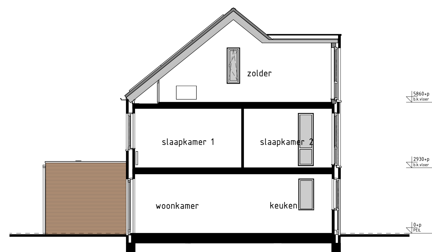
type P1 bwnr get.:736 DOORSNEDE P1-P1
