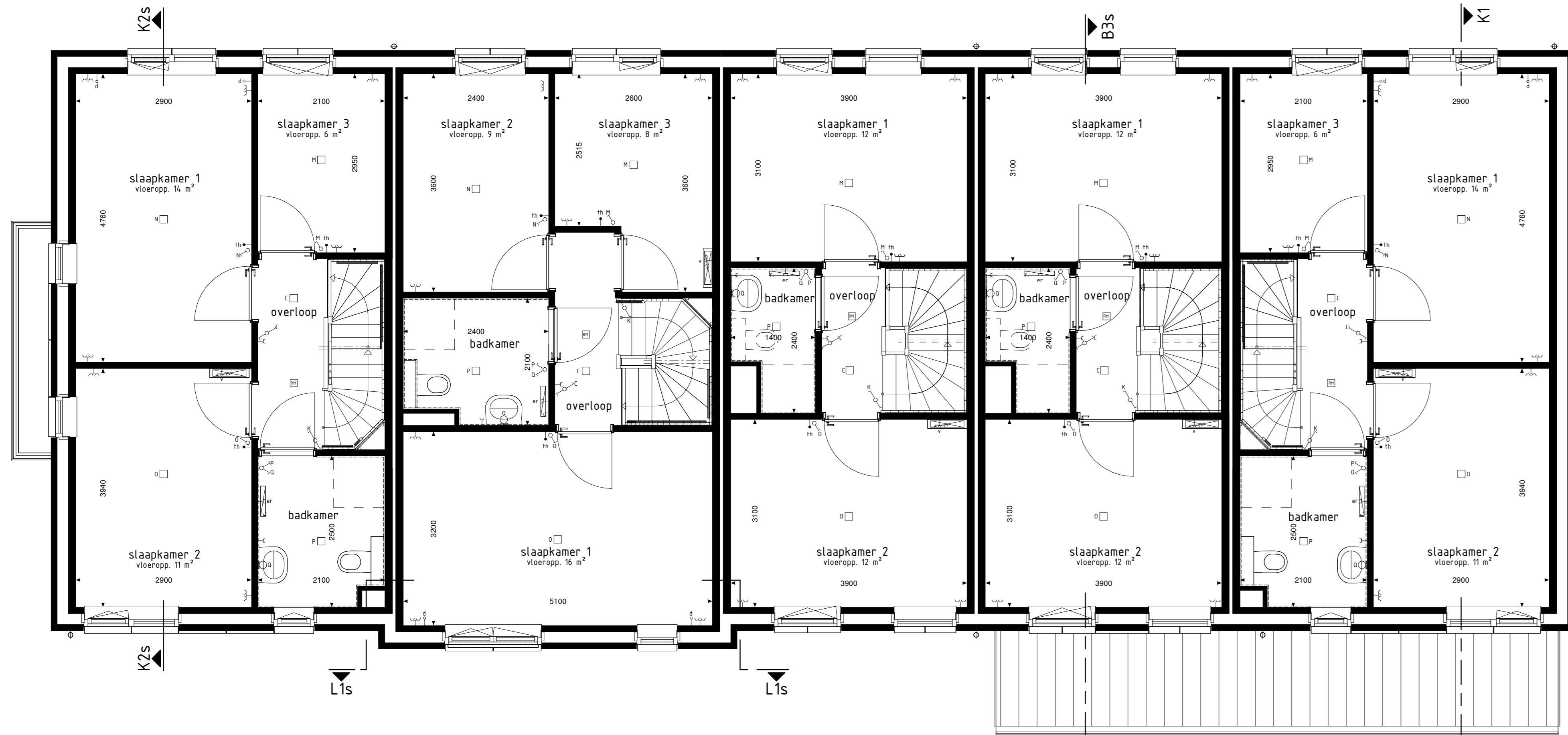
type K2s bwnr get.:179 1e VERDIEPING
