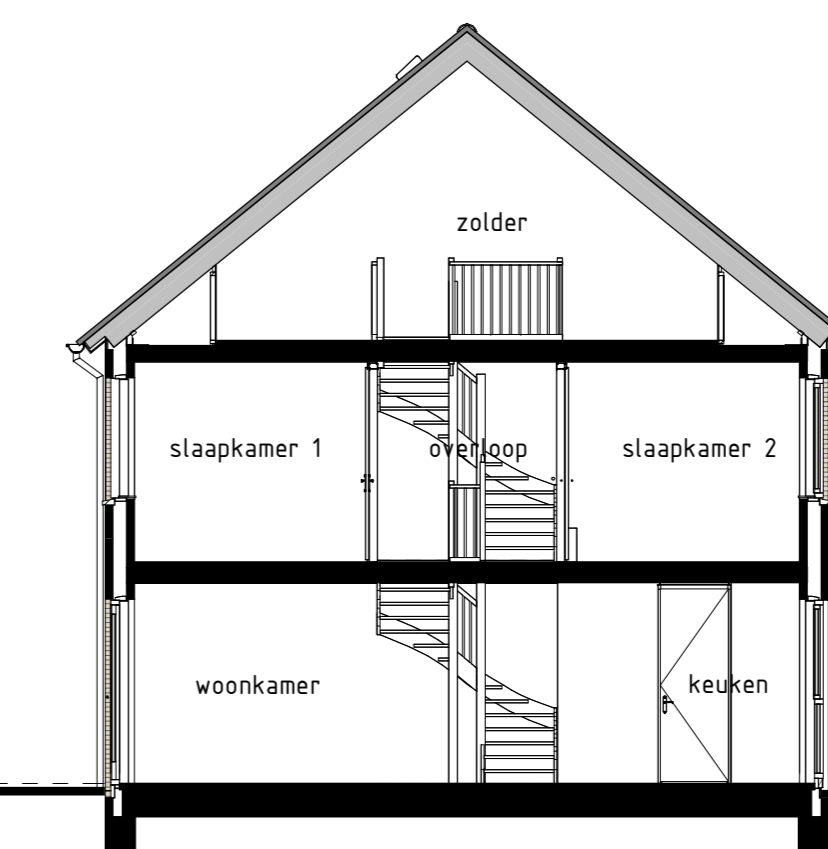
type B2s, B3s bwnr get.:181, 182 DOORSNEDE B3-B3
