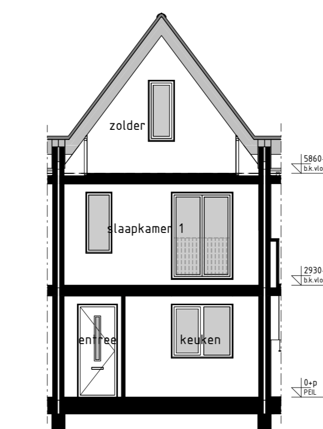
type L1s bwnr get.:180 DOORSNEDE L1s-L1s
