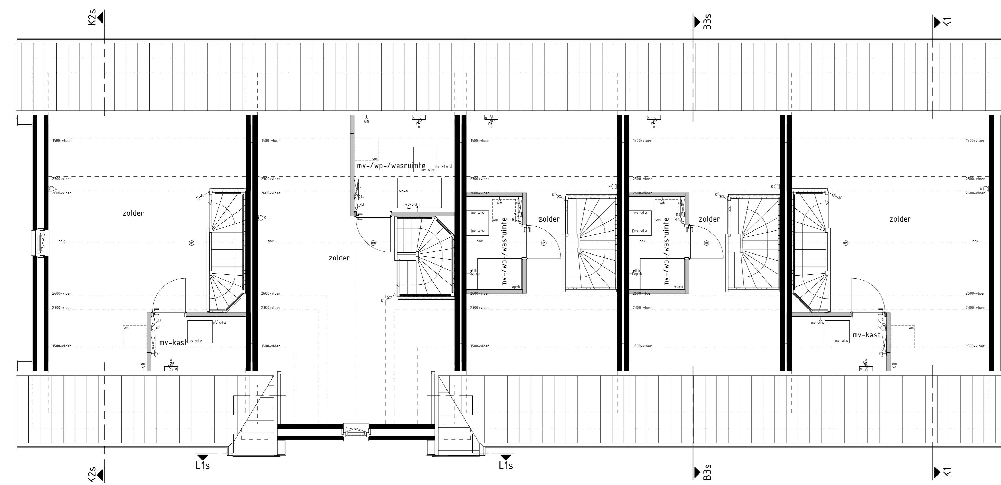
type K2s bwnr get.:179 2e VERDIEPING
