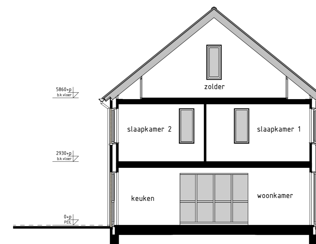
type K2s bwnr get.:179 DOORSNEDE K2s-K2s
