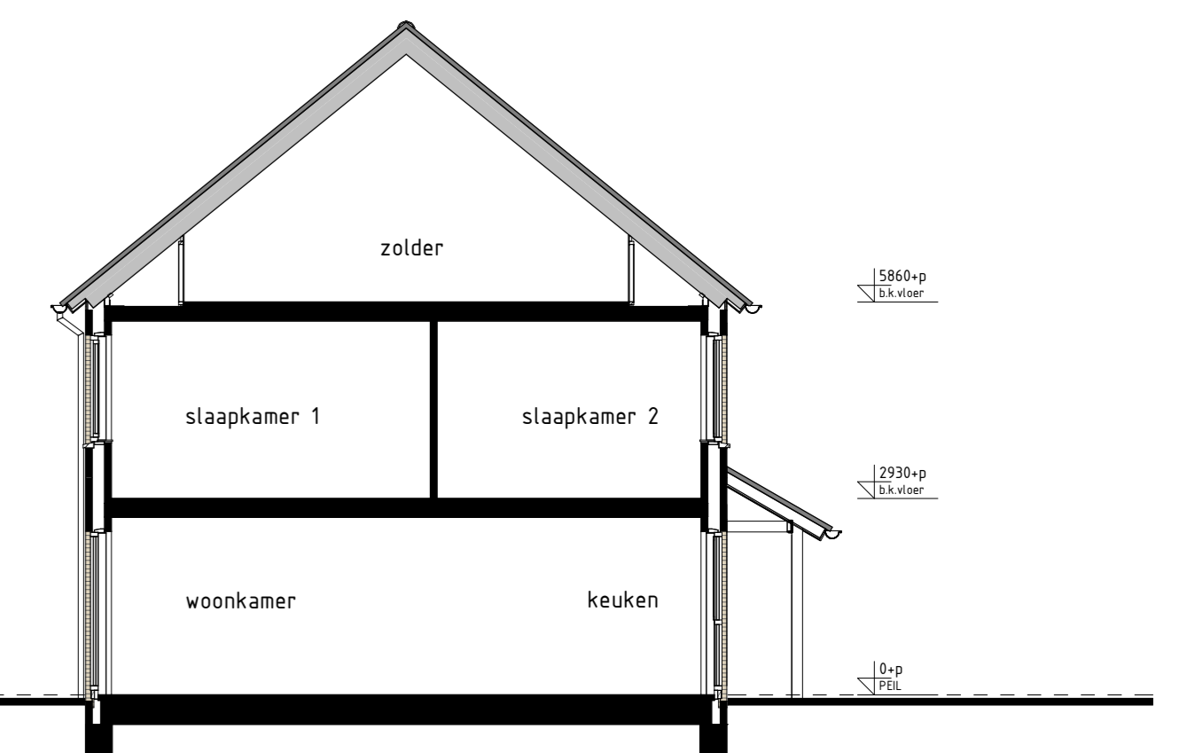
type K1 bwnr get.:183 DOORSNEDE K1-K1
