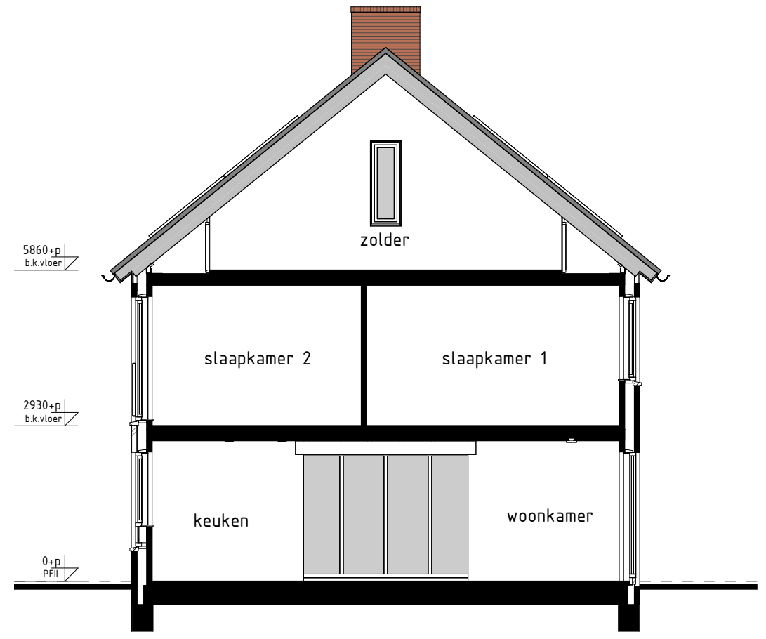
type F3sp bwnr get.: 77 DOORSNEDE F3sp-F3sp
