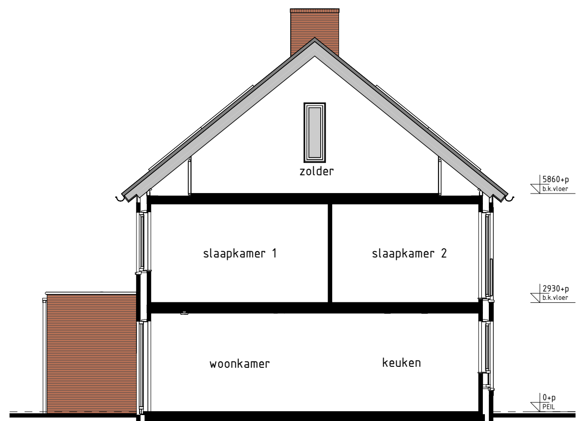
type F2sp bwnr get.: 72 DOORSNEDE F2sp-F2sp
