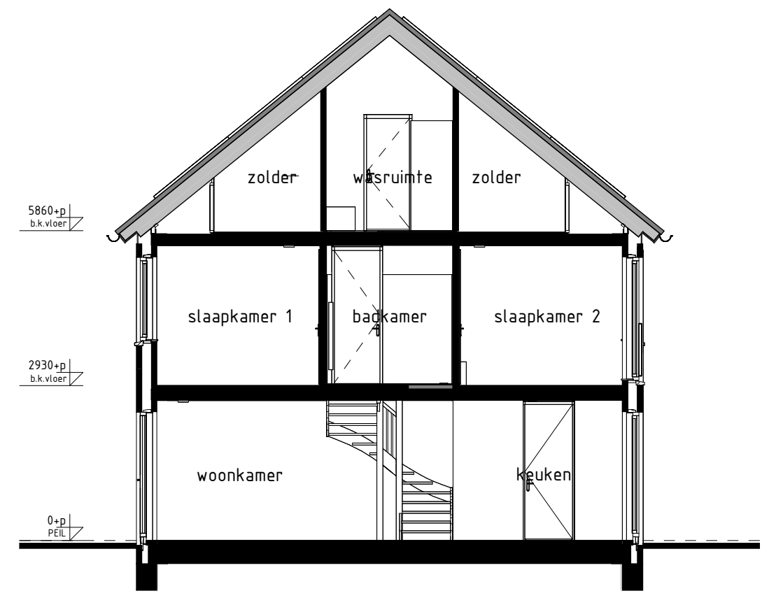
type G5, G6, G6sp bwnr get.: 76 bwnr gesp.: 73, 74, 75 DOORSNEDE G6sp-G6sp
