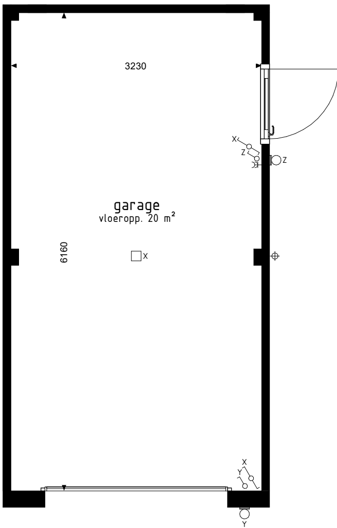
type E2sp bwnr get.: 426 BEGANE GROND 1 : 50
