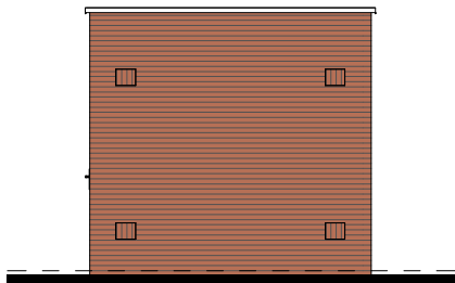
type E2sp bwnr get.: 426 ACHTERGEVEL 1 : 100
