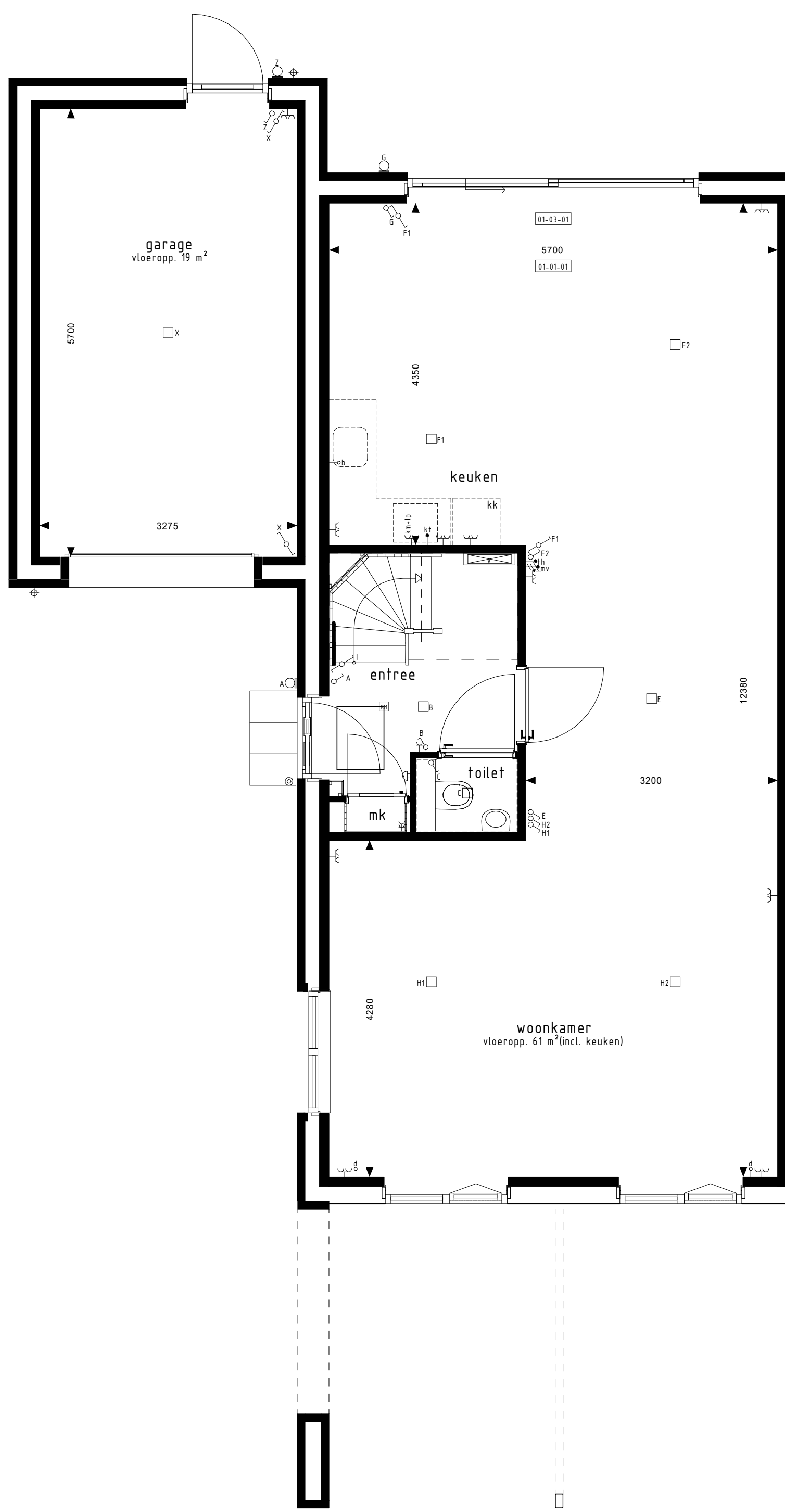
BEGANE GROND
