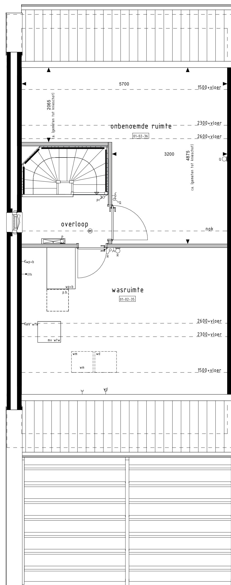
2e VERDIEPING
