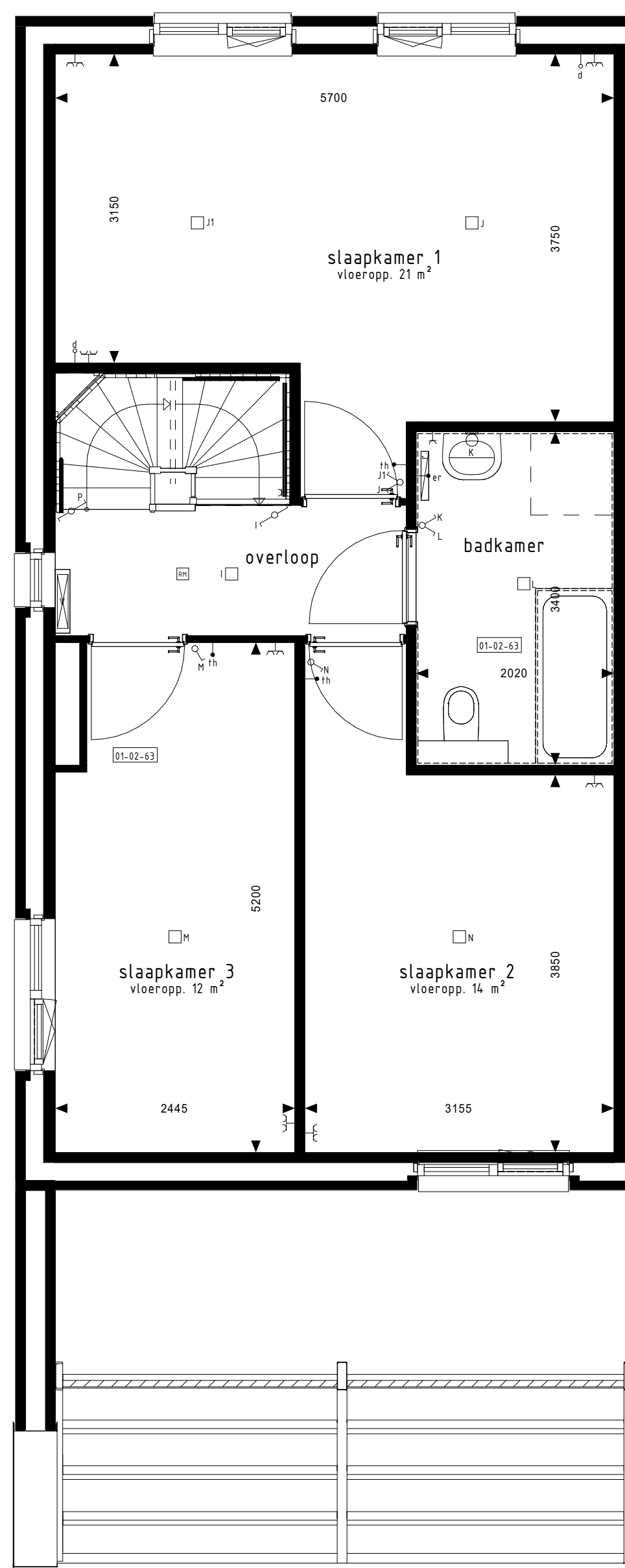
1e VERDIEPING
