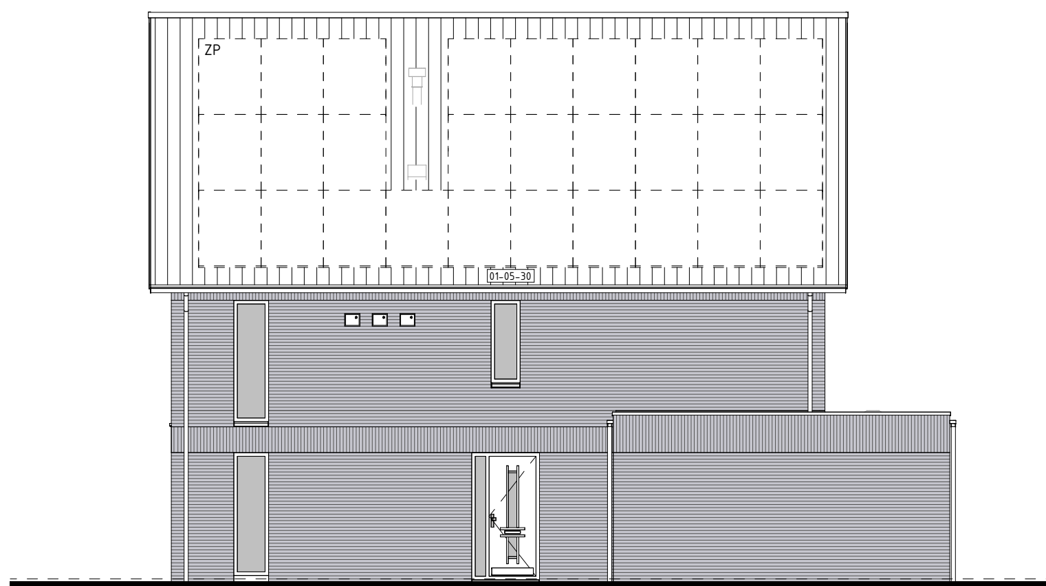
type N1sp bwnr get.:49 RECHTERGEVEL
