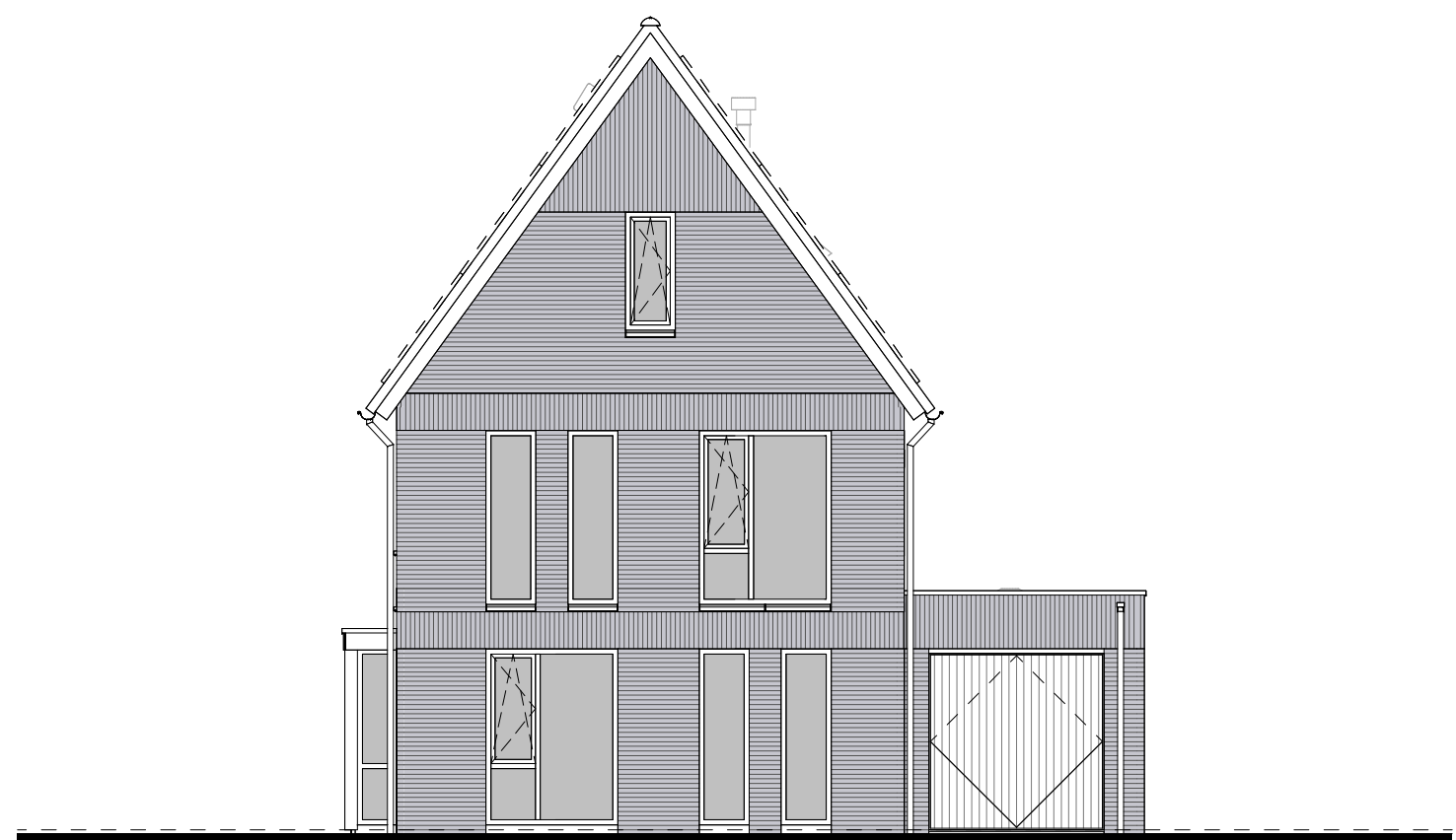
type N1sp bwnr get.:49 VOORGEVEL
