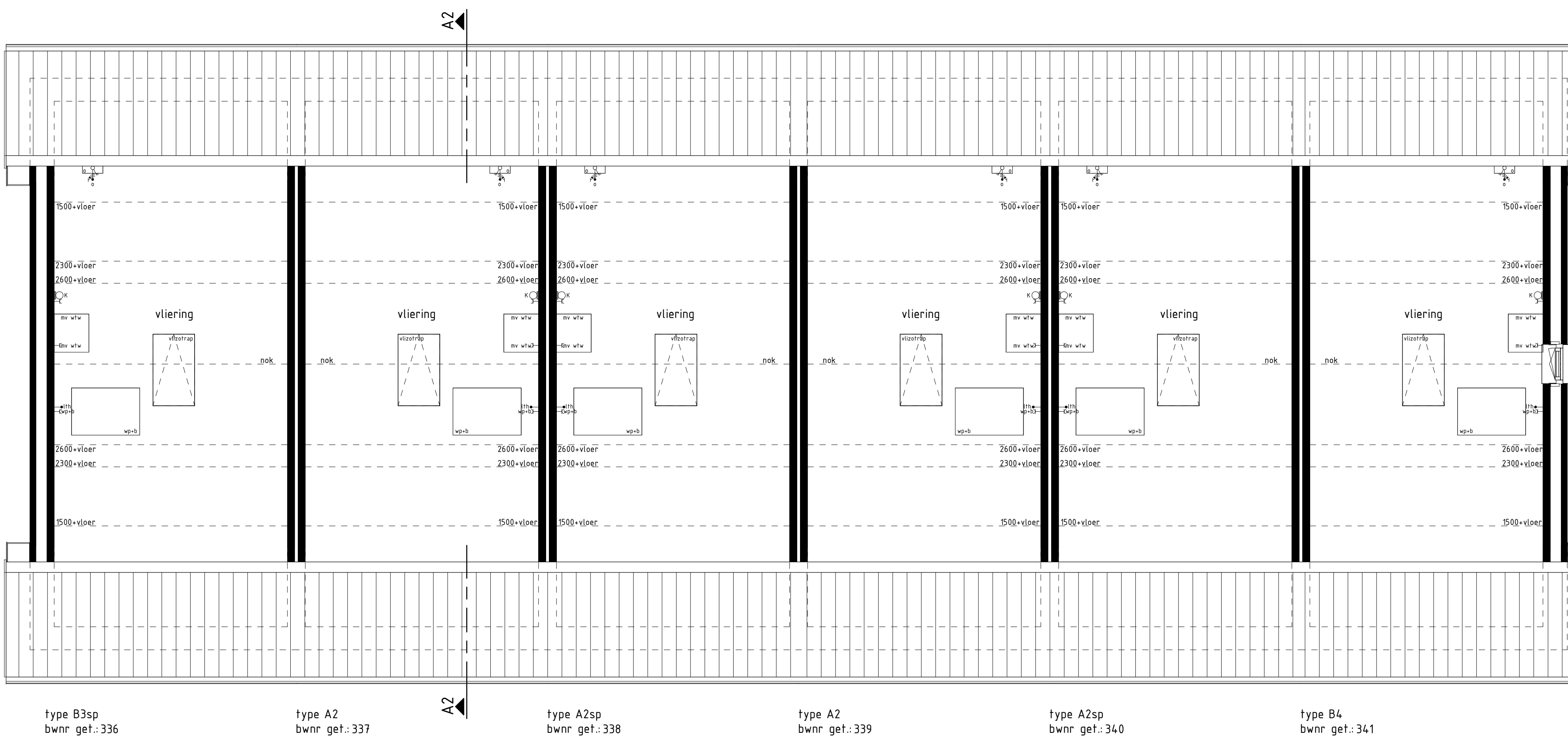
type B3sp bwnr get.:336 type A2 bwnr get.:337 type A2sp bwnr get.:338 type A2 bwnr get.:339 type A2sp bwnr get.:340 type B4 bwnr get.:341 1e VERDIEPING 1:100
