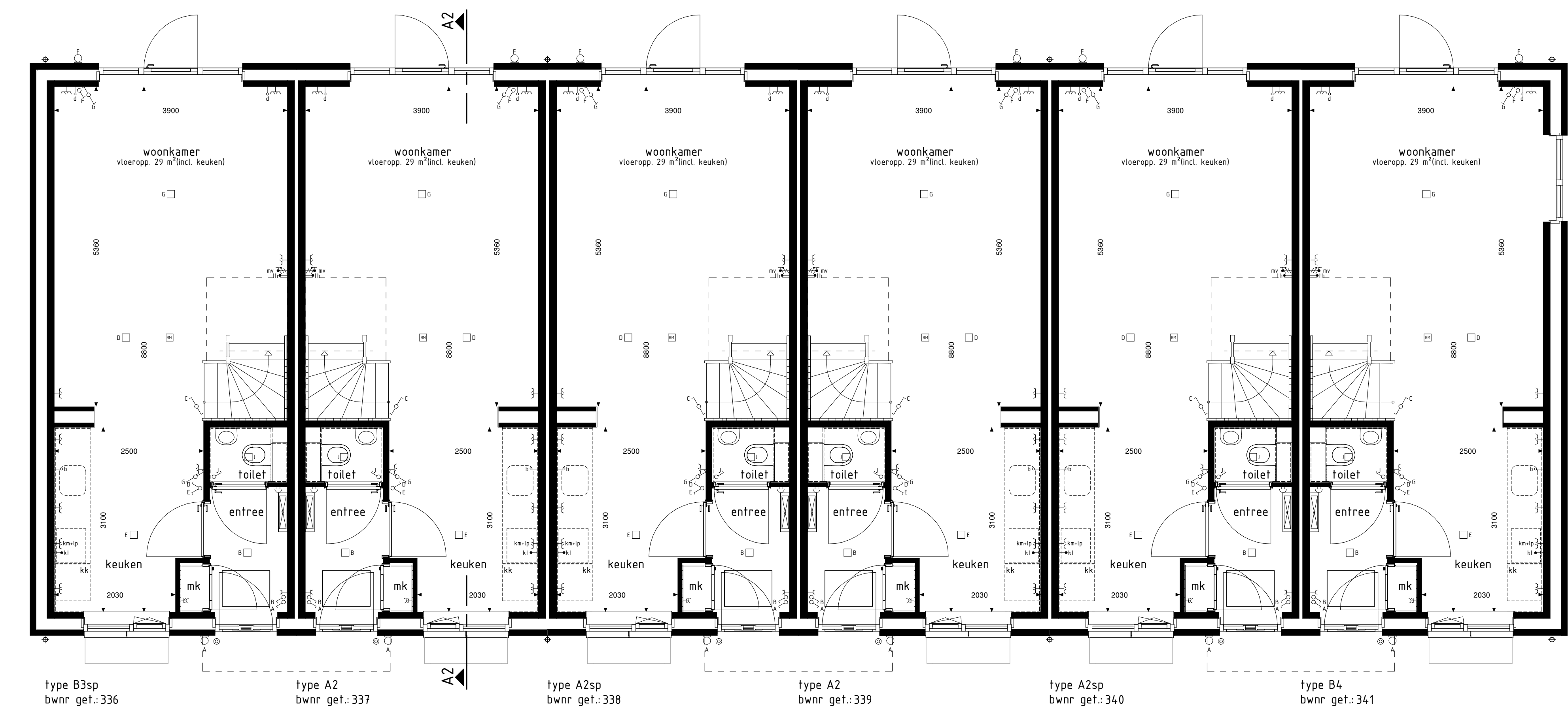
type B3sp bwnr get.:336 type A2 bwnr get.:337 type A2sp bwnr get.:338 type A2 bwnr get.:339 type A2sp bwnr get.:340 type B4 bwnr get.:341 BEGANE GROND 1:100
