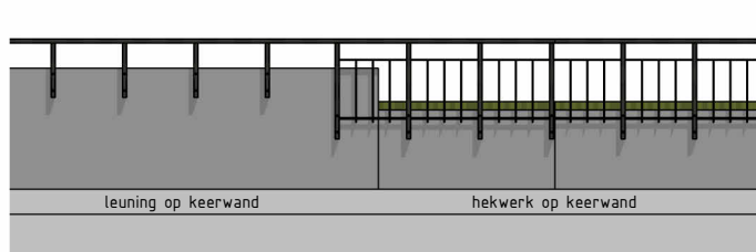
aanzicht hekwerk op keerwand
