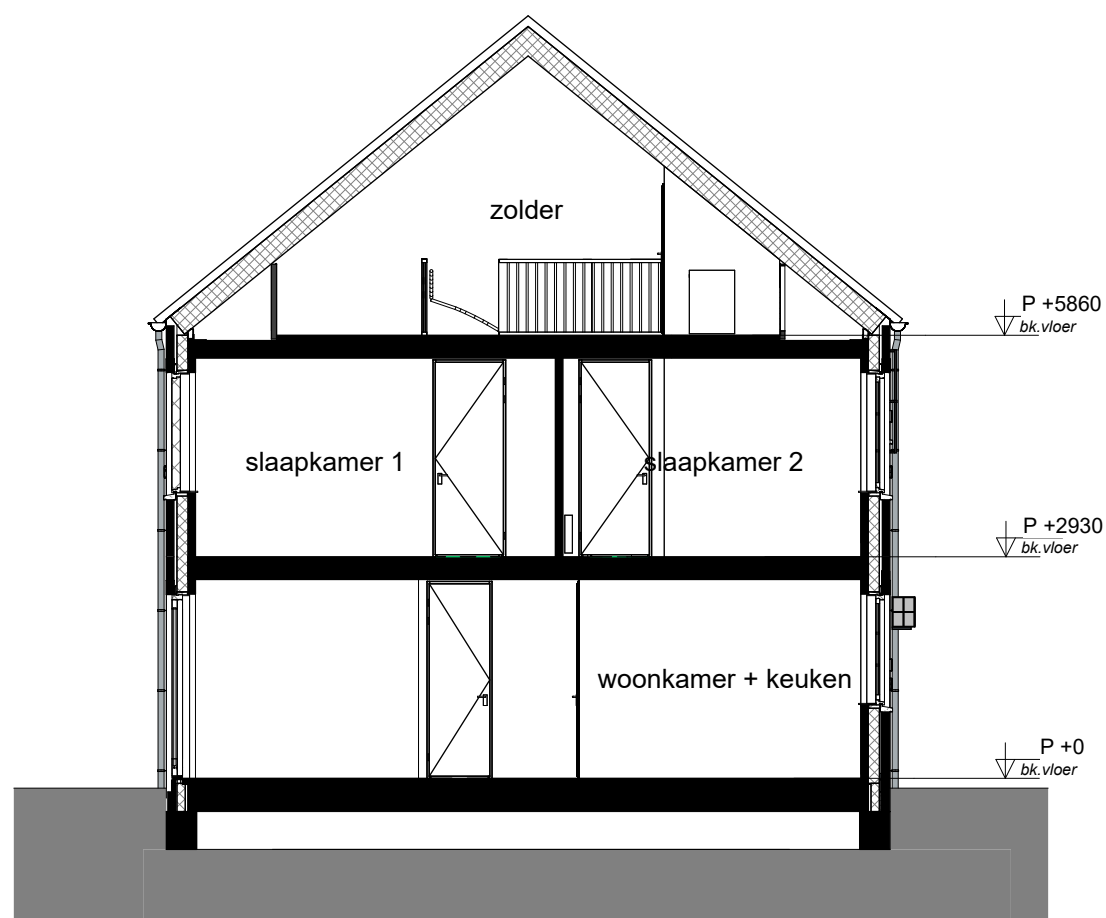
doorsnede B-B 1 : 100
