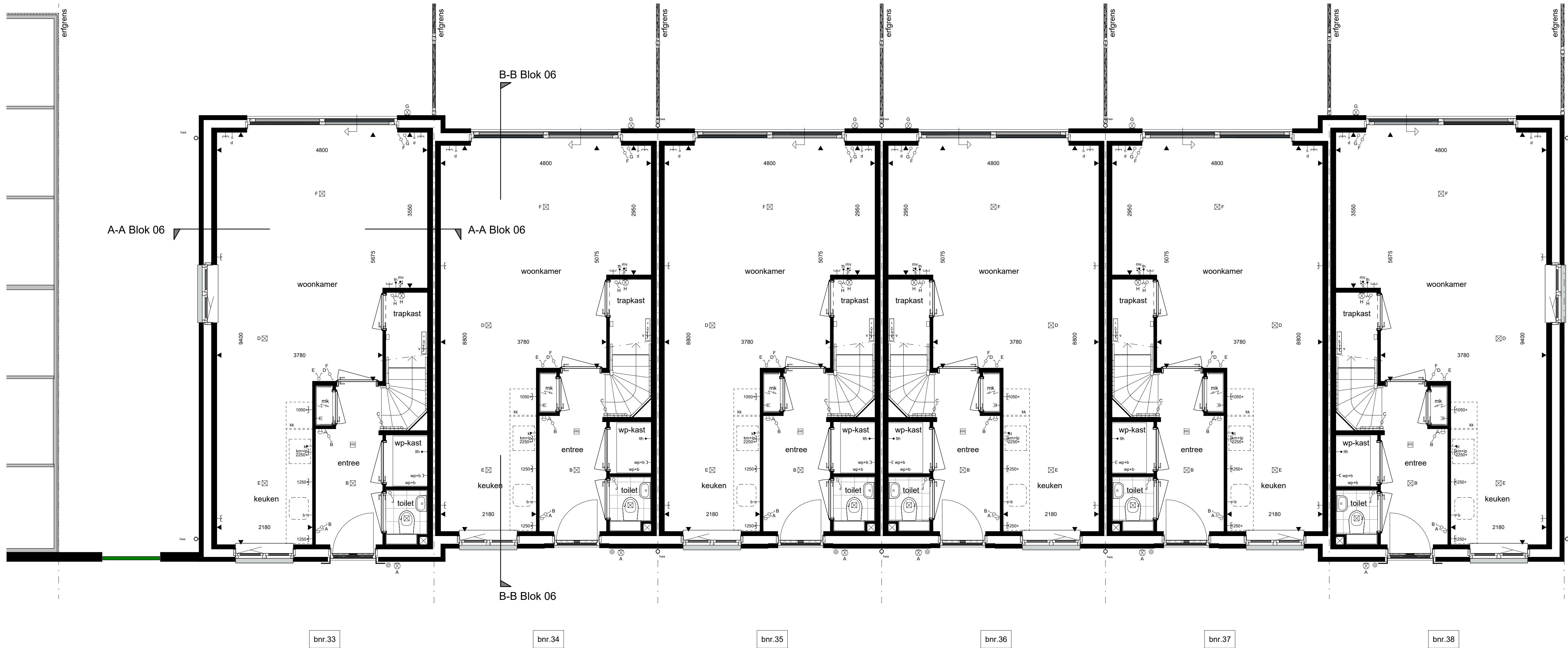
begane grond 1 : 50
