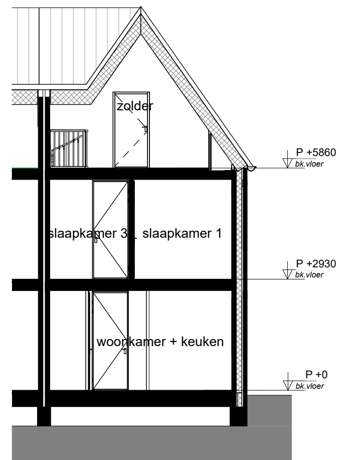
doorsnede A-A 1 : 100
