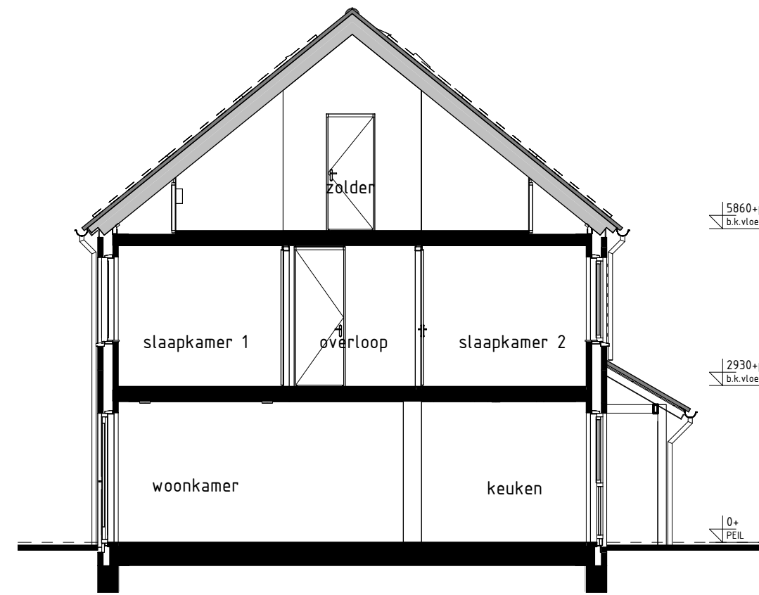
type B2 bwnr get.:150, 151 DOORSNEDE B2-B2 1:100
