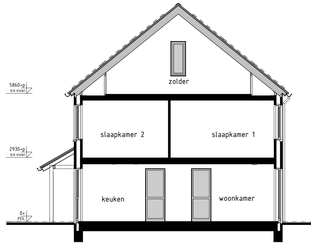
type K1s bwnr get.:149 DOORSNEDE K1s-K1s 1:100
