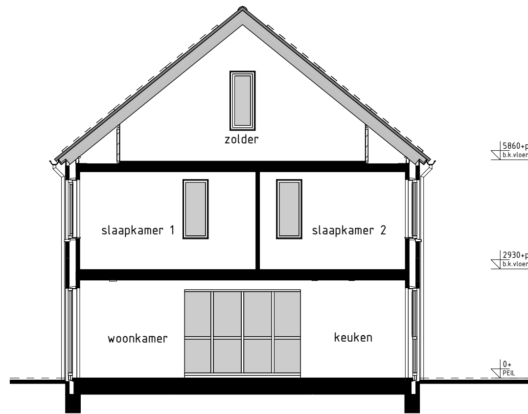
type K2 bwnr get.:154 DOORSNEDE K2-K2 1:100
