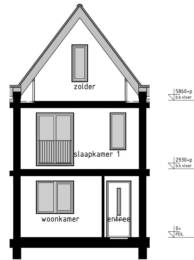
type L1 bwnr get.:153 DOORSNEDE L1-L1 1:100
