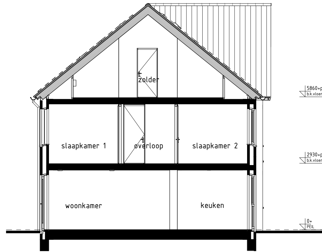
type B3 bwnr get.:152 DOORSNEDE B3-B3 1:100
