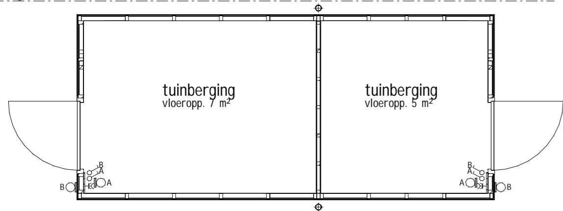
bwnr get.:421 PLATTEGROND 1 : 50
