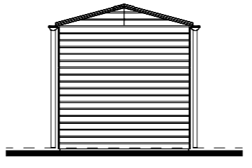
bwnr get.:428 bwnr gesp.:293, 300 LINKER ZIJGEVEL
