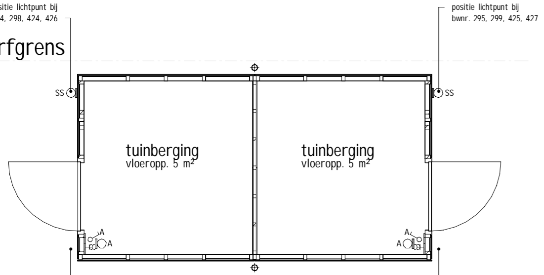
bwnr get.:294, 296, 298, 424, 426 PLATTEGROND 1 : 50
