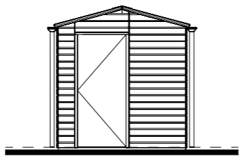
bwnr get.:428 bwnr gesp.:293, 300 RECHTER ZIJGEVEL
