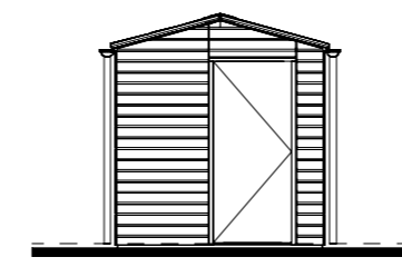
RECHTER ZIJGEVEL 1 : 100
