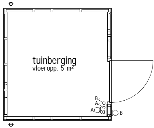
bwnr get.:423 PLATTEGROND 1 : 50
