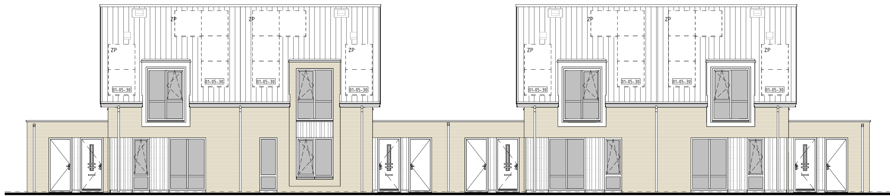
type E1 bwnr gef.:17 type E2sp bwnr gef.:18 type E3 bwnr gef.:19 type E2sp bwnr gef.:20 VÖÖRGEVEL
