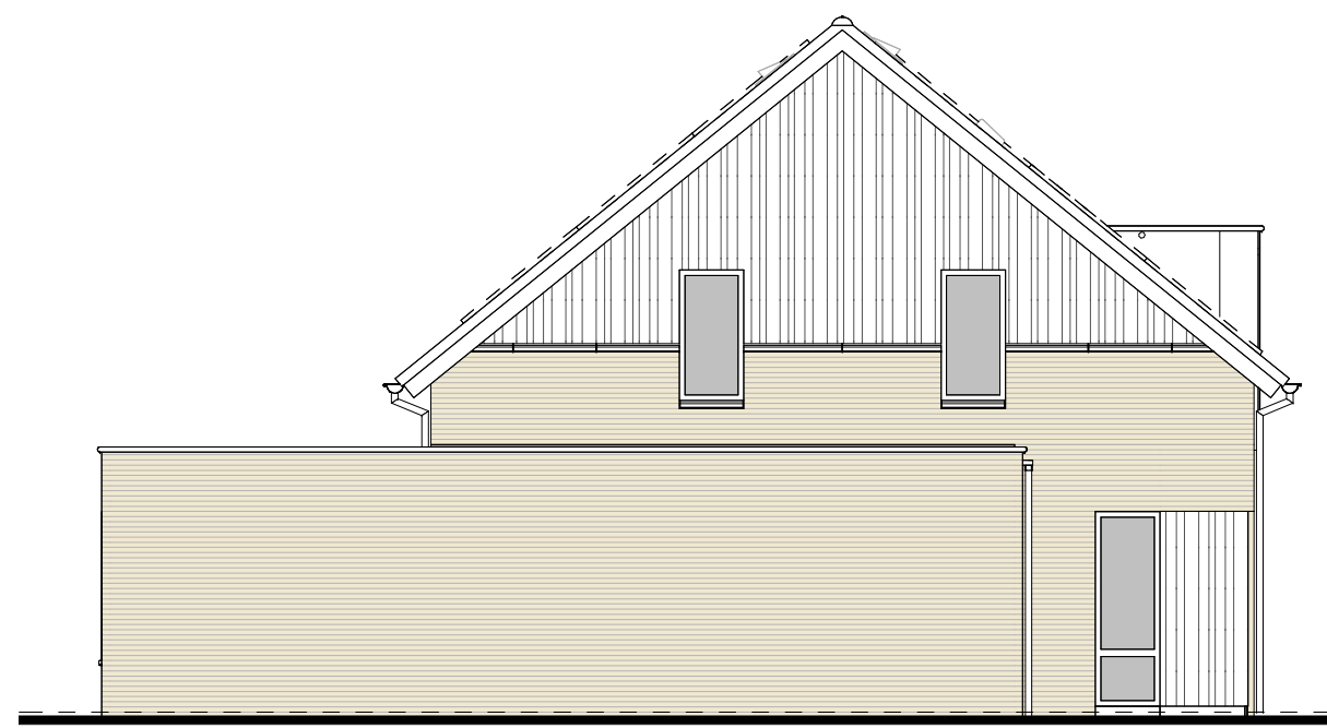
type E1 bwnr gef.:17 LINKERGEVEL
