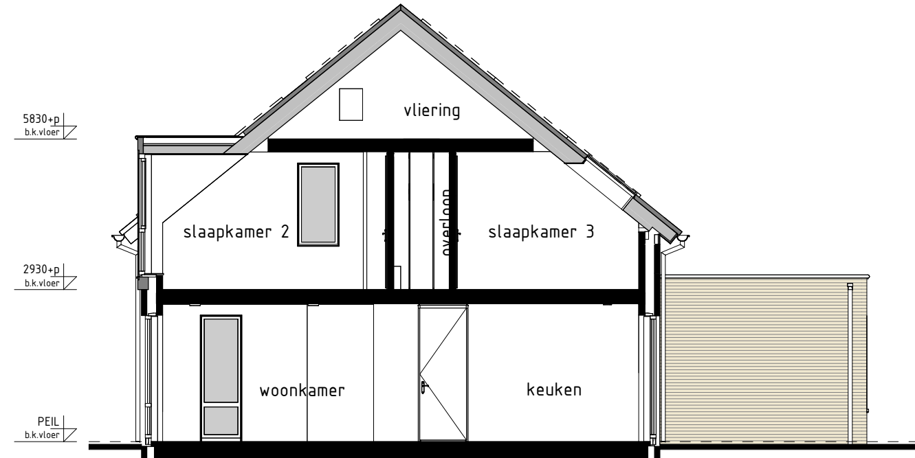
type E1, E2sp, E3 bwnr gef.:17, 19 bwnr gesp.:20 DOORSNEDE E1-E1
