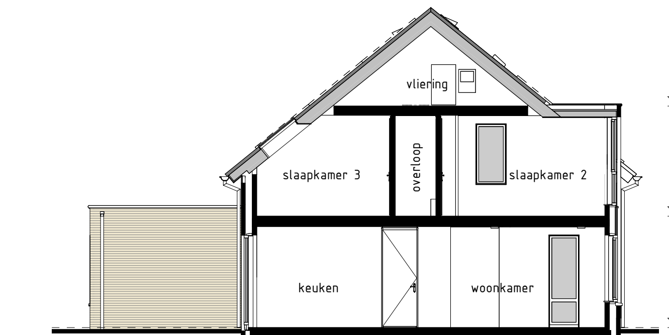
type E2sp bwnr gef.:18 DOORSNEDE E2sp-E2sp
