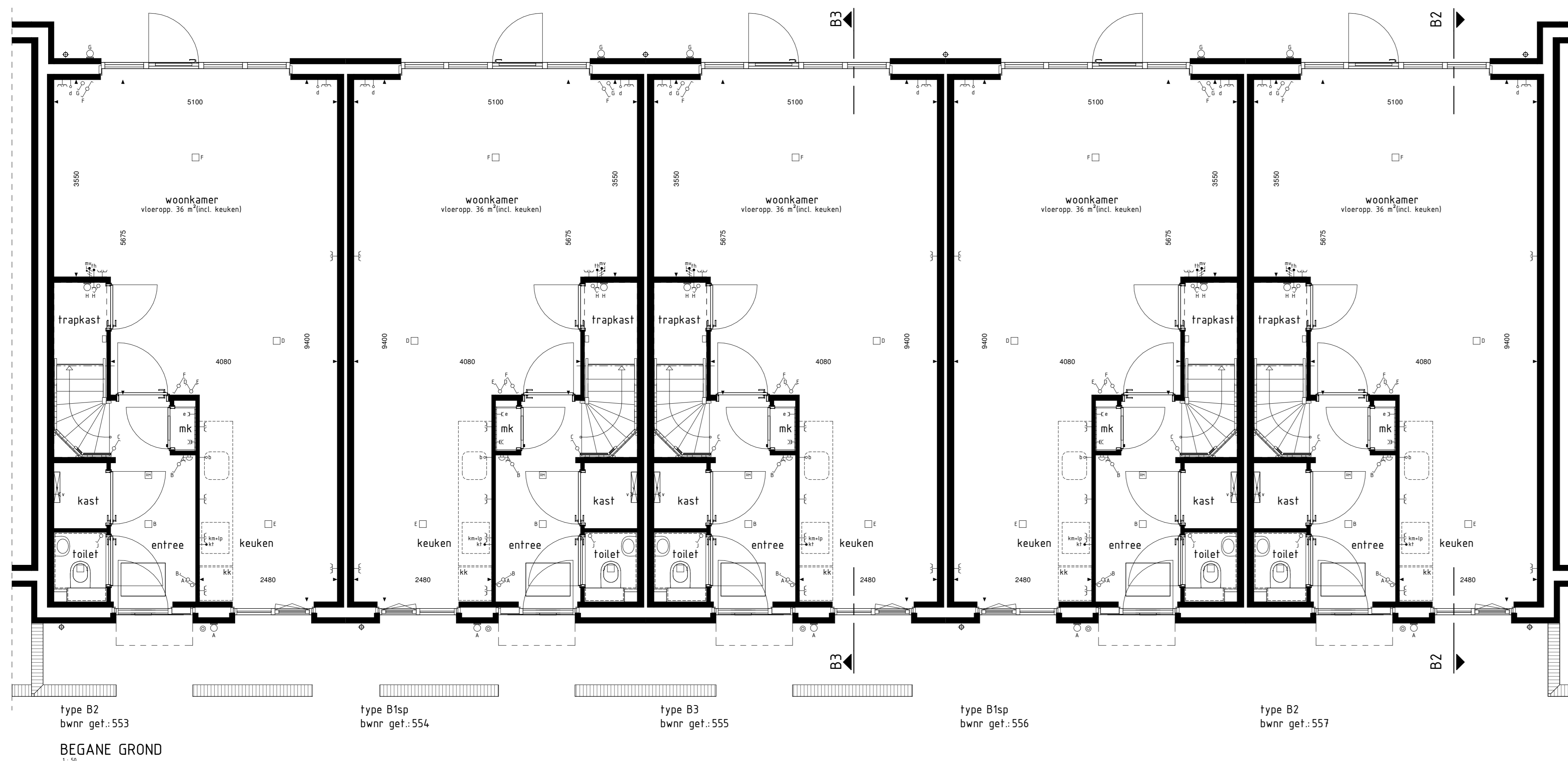
BEGANE GROND
