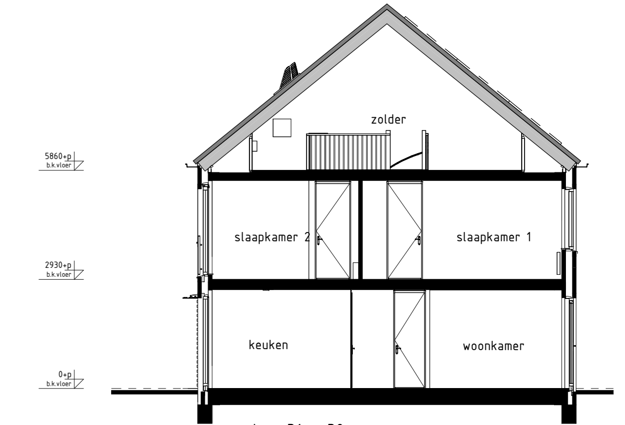
DOORSNEDE B2-B2
