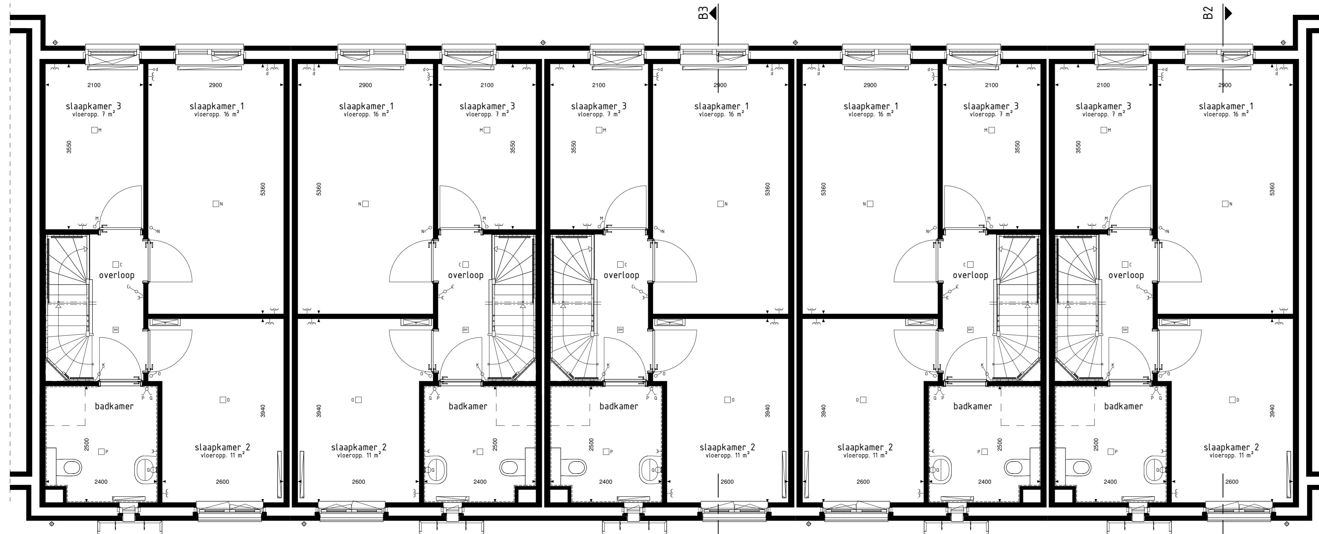
1e VERDIEPING
