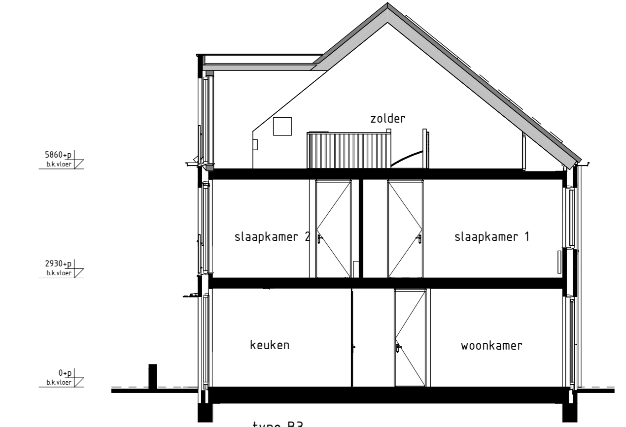
DOORSNEDE B3-B3
