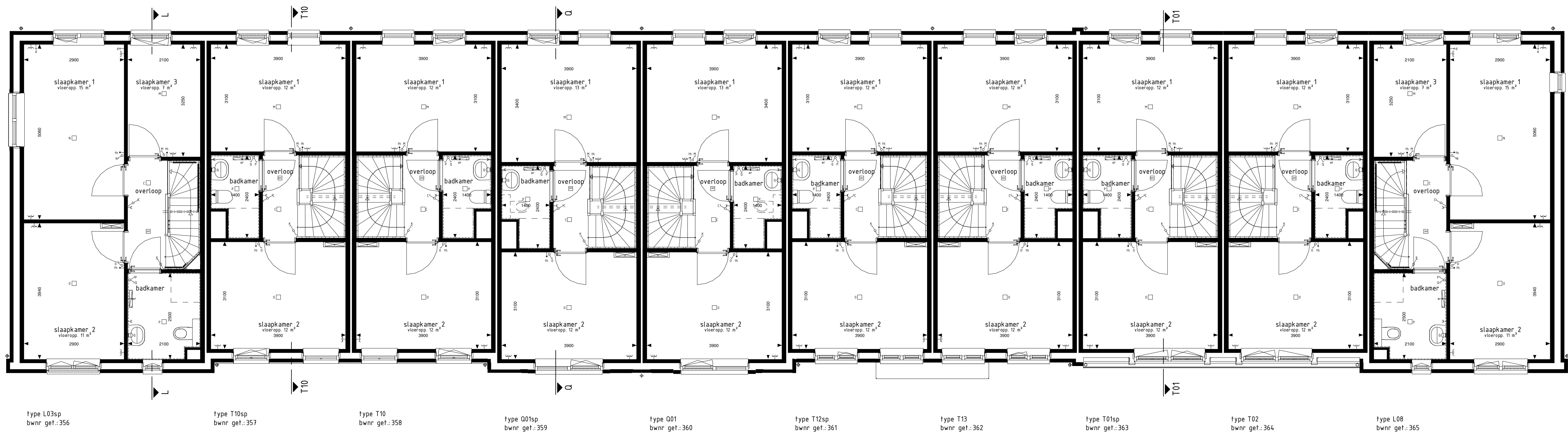
1e VERDIEPING
