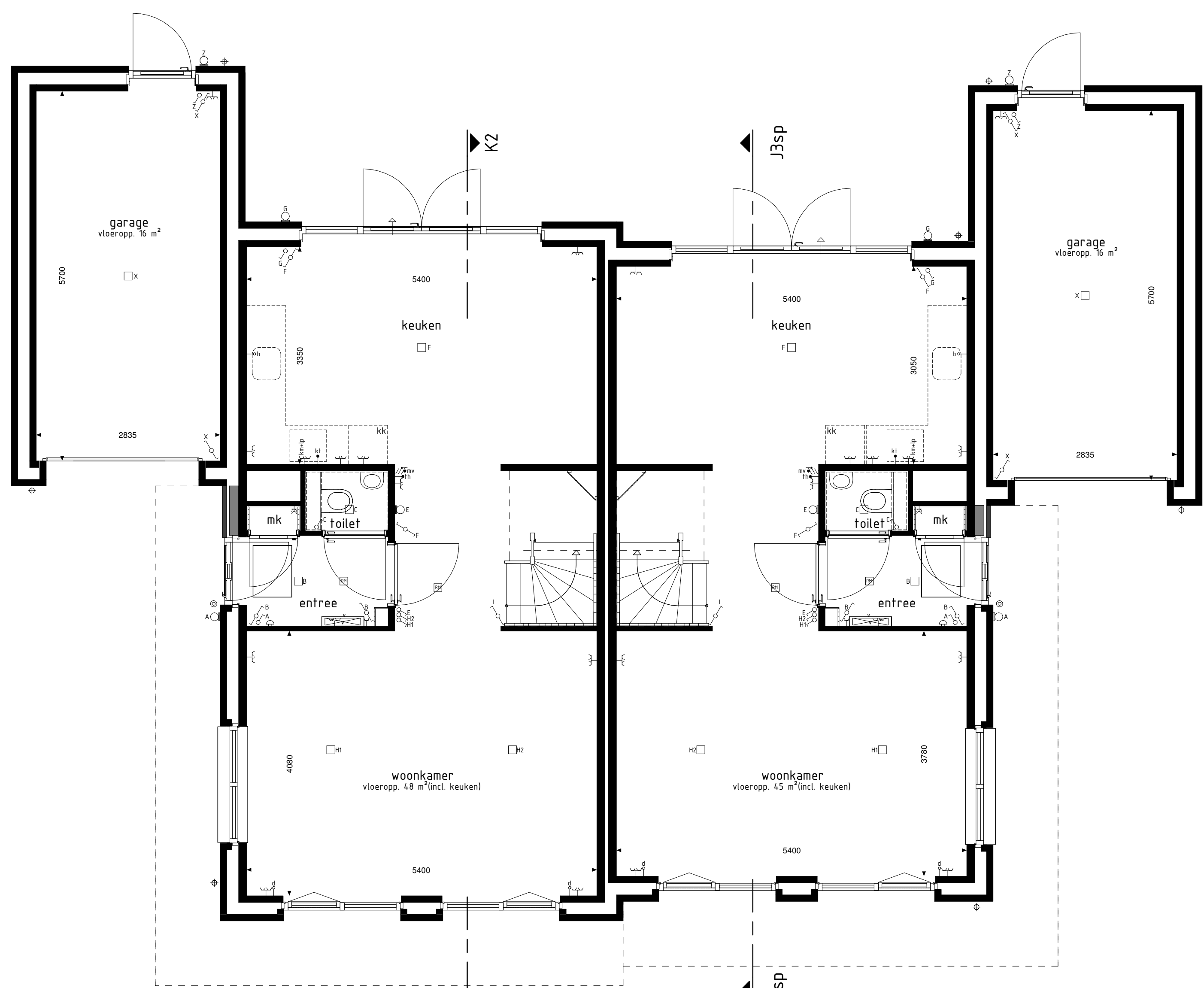
type K2 bwnr get.: 217 type J3sp bwnr get.: 218 BEGANE GROND
