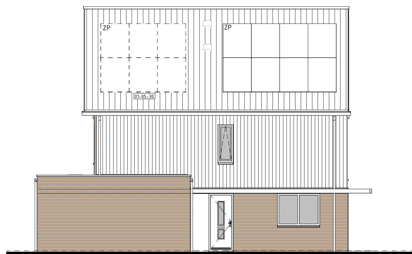
type K2 bwnr get.: 217 LINKERGEVEL
