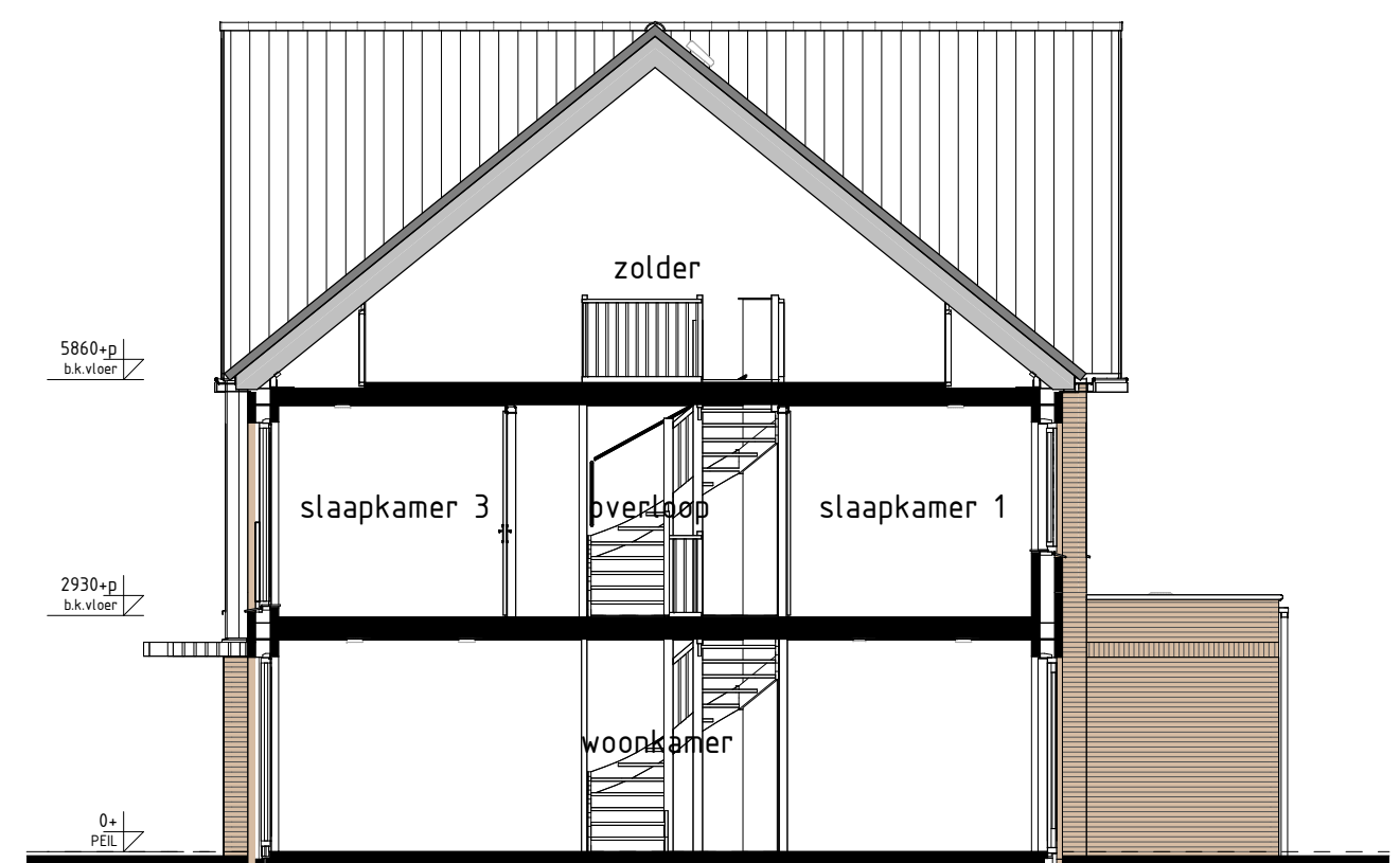
type J3sp bwnr get.: 218 DOORSNEDE J3sp-J3sp
