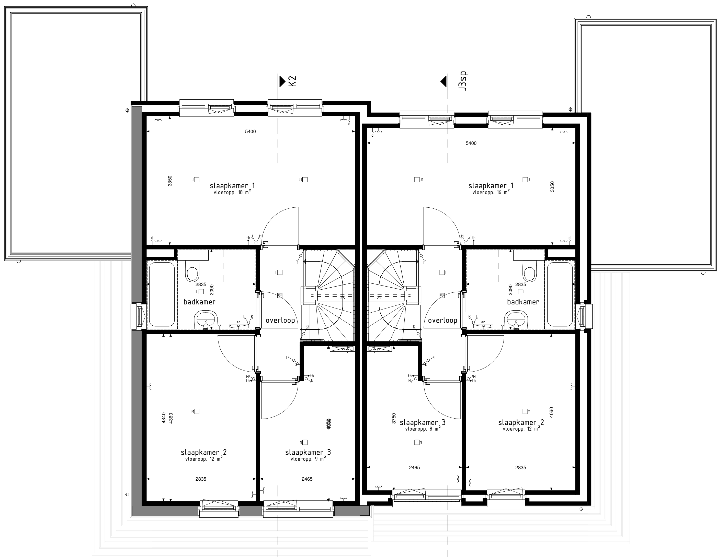
type K2 bwnr get.: 217 type J3sp bwnr get.: 218 1e VERDIEPING
