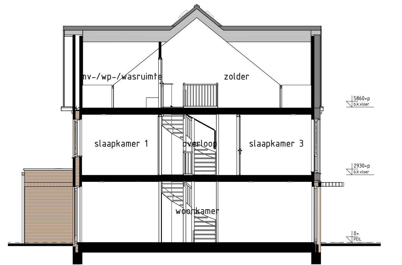
type K2 bwnr get.: 217 DOORSNEDE K2-K2
