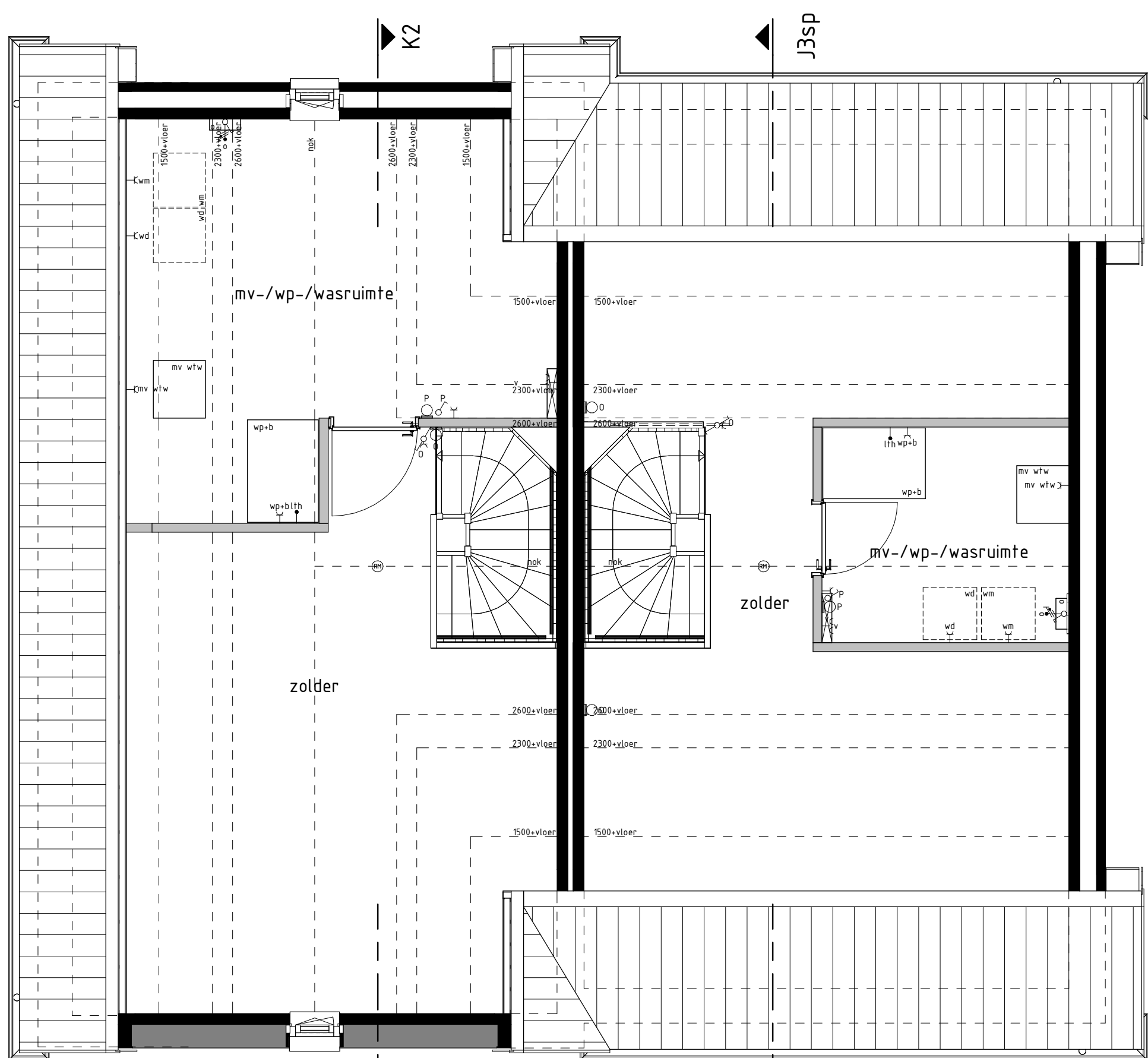
type K2 bwnr get.: 217 type J3sp bwnr get.: 218 2e VERDIEPING
