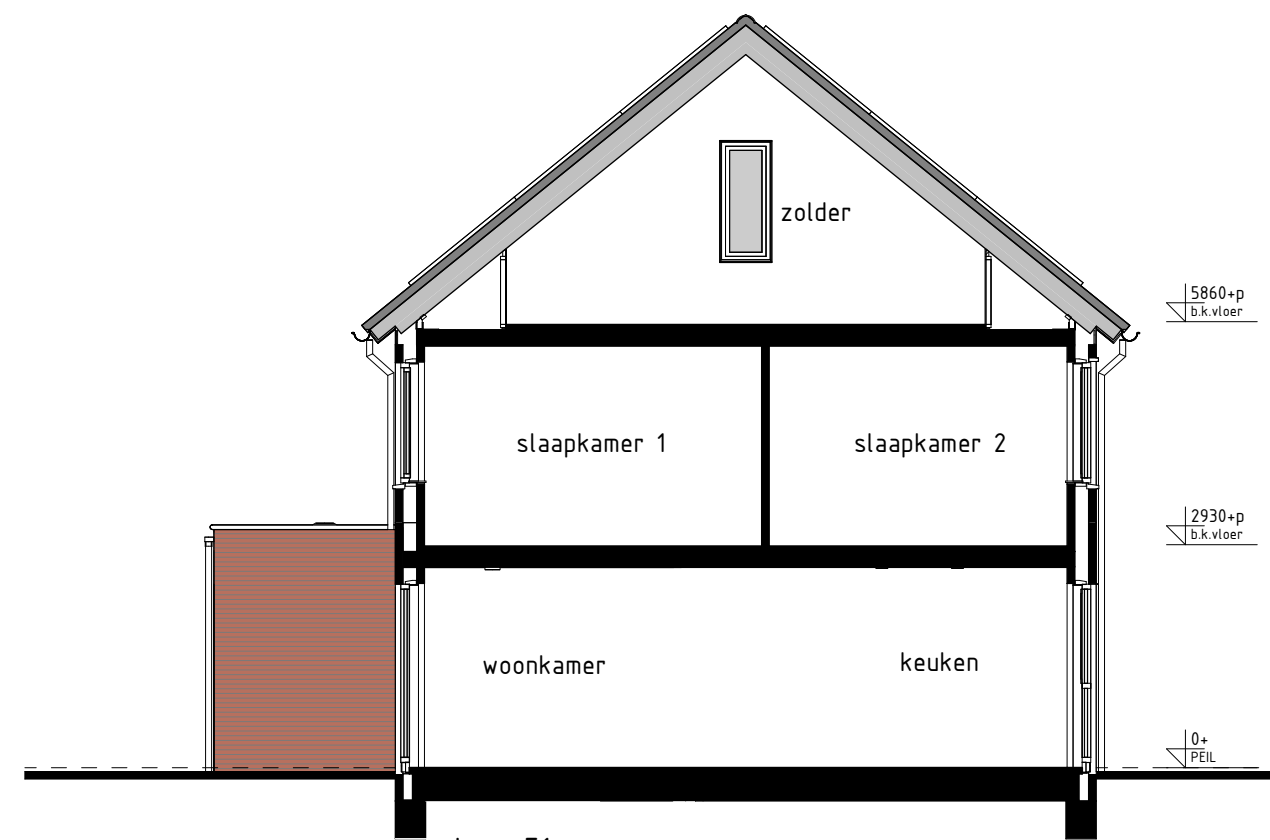
type E1 bwnr get.:114 DOORSNEDE E1-E1 1:100
