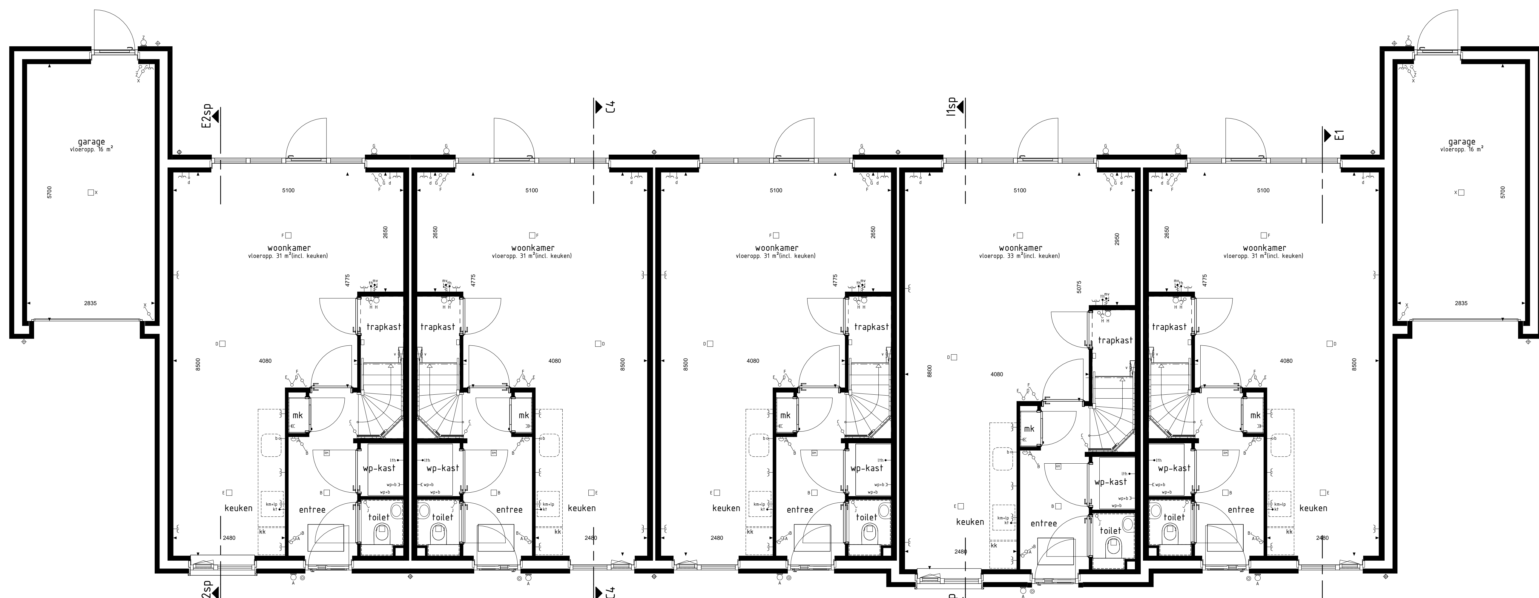
type E2sp bwnr get.:110 BEGANE GROND
