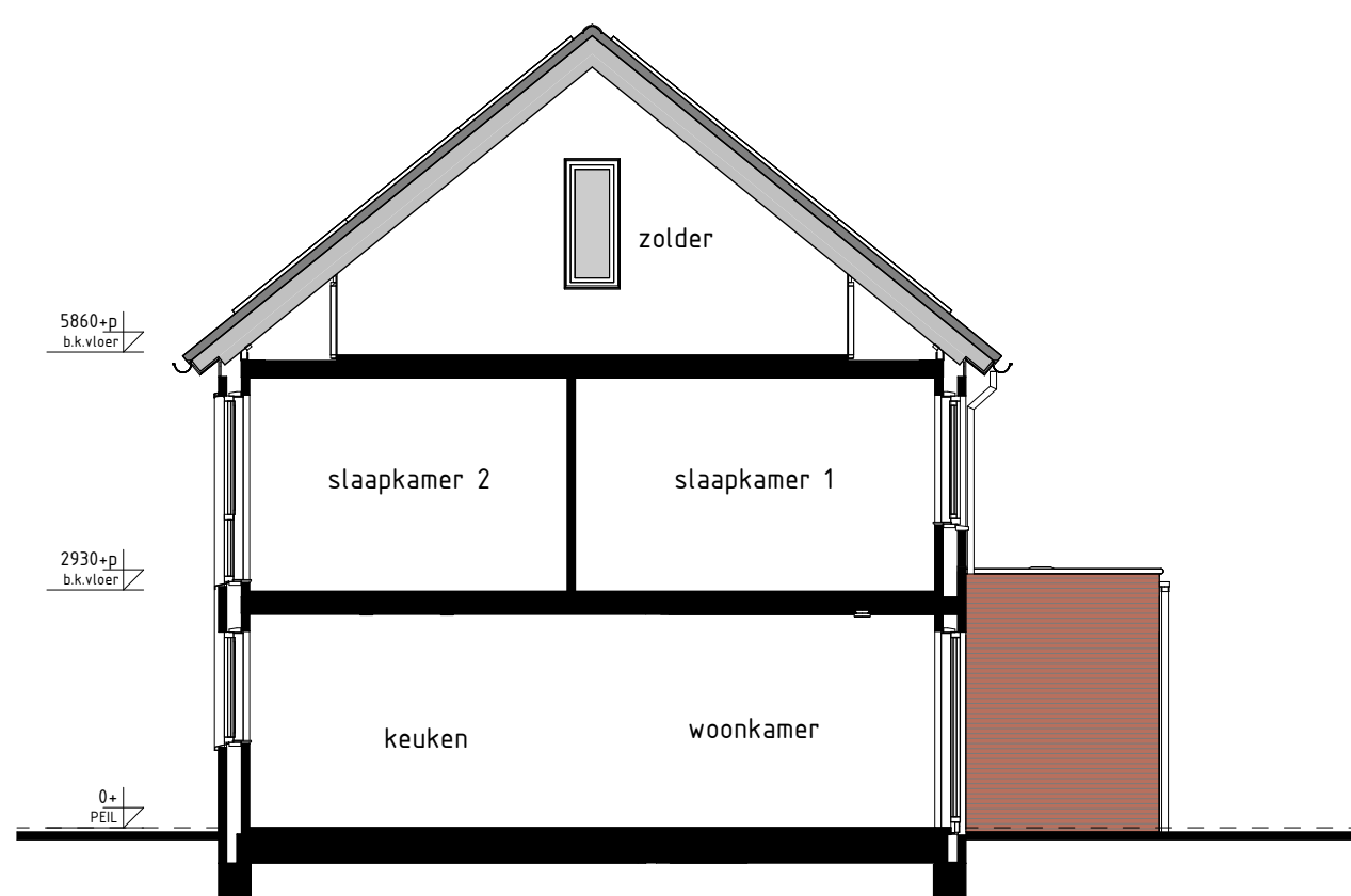
type E2sp bwnr get.:110 DOORSNEDE E2sp-E2sp 1:100
