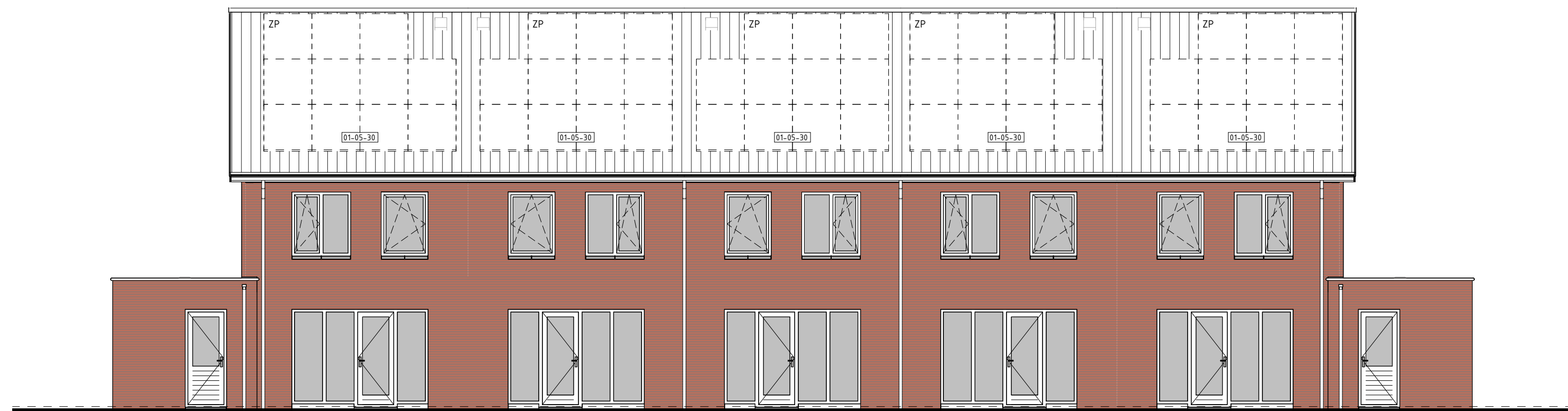
type E1 bwnr get.:114 ACHTERGEVEL 1:100
