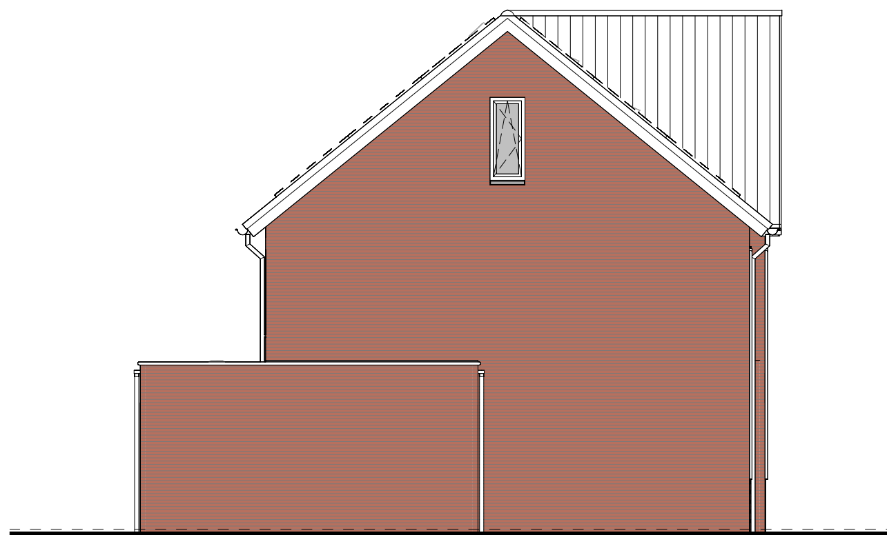
type E2sp bwnr get.:110 LINKERGEVEL 1:100
