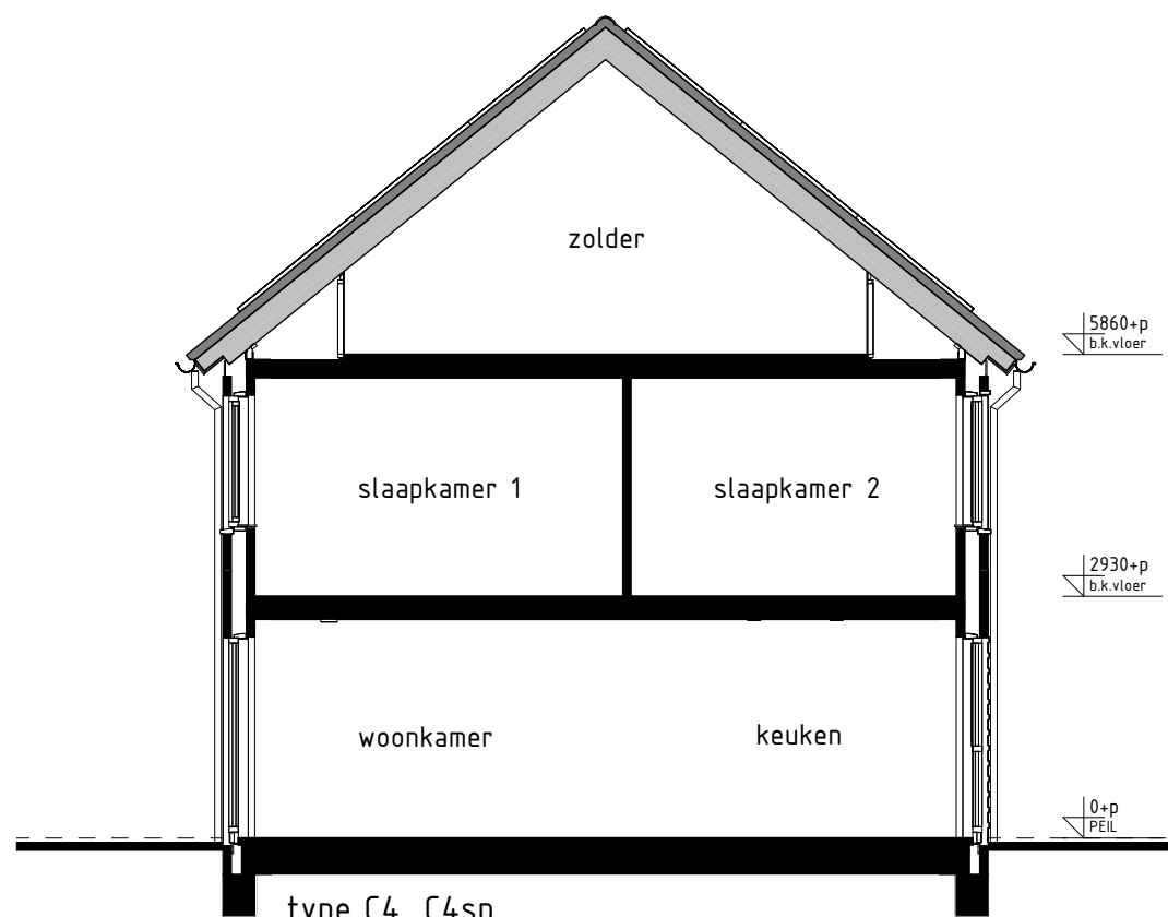
type C4, C4sp bwnr get.:111 bwnr gesp.:112 DOORSNEDE C4-C4 1:100
