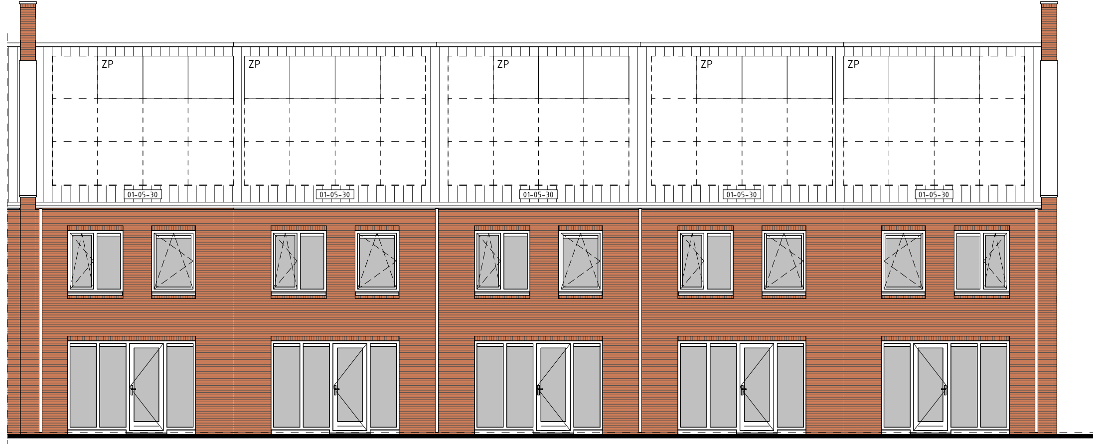
type B4 bwnr get.:539 ACHTERGEVEL 1:50
