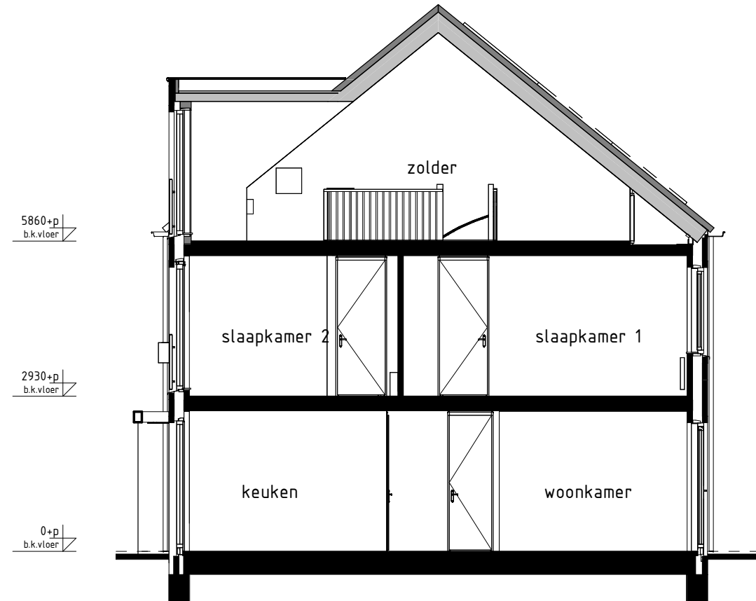
type B5 bwnr get.:538 DOORSNEDE B5-B5 1:50
