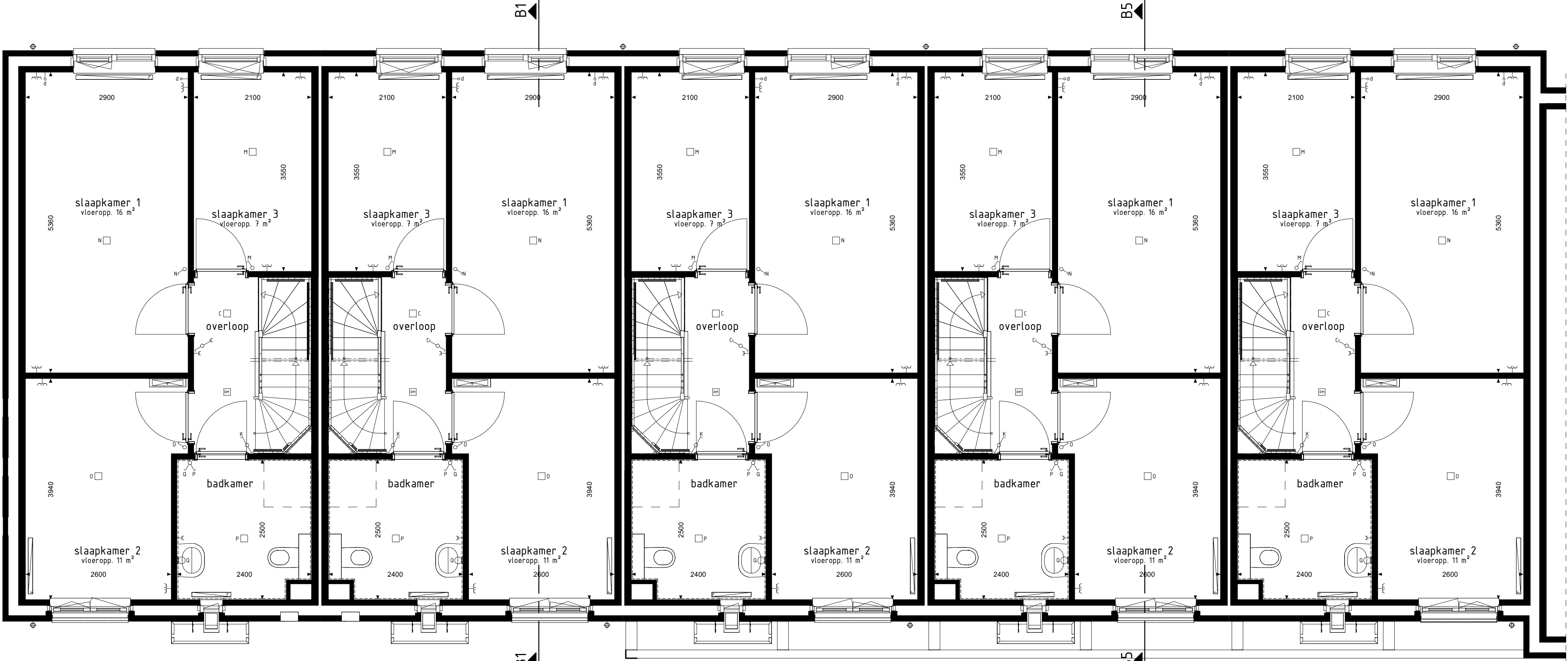
type A2sp bwnr get.:535 1e VERDIEPING 1:50
