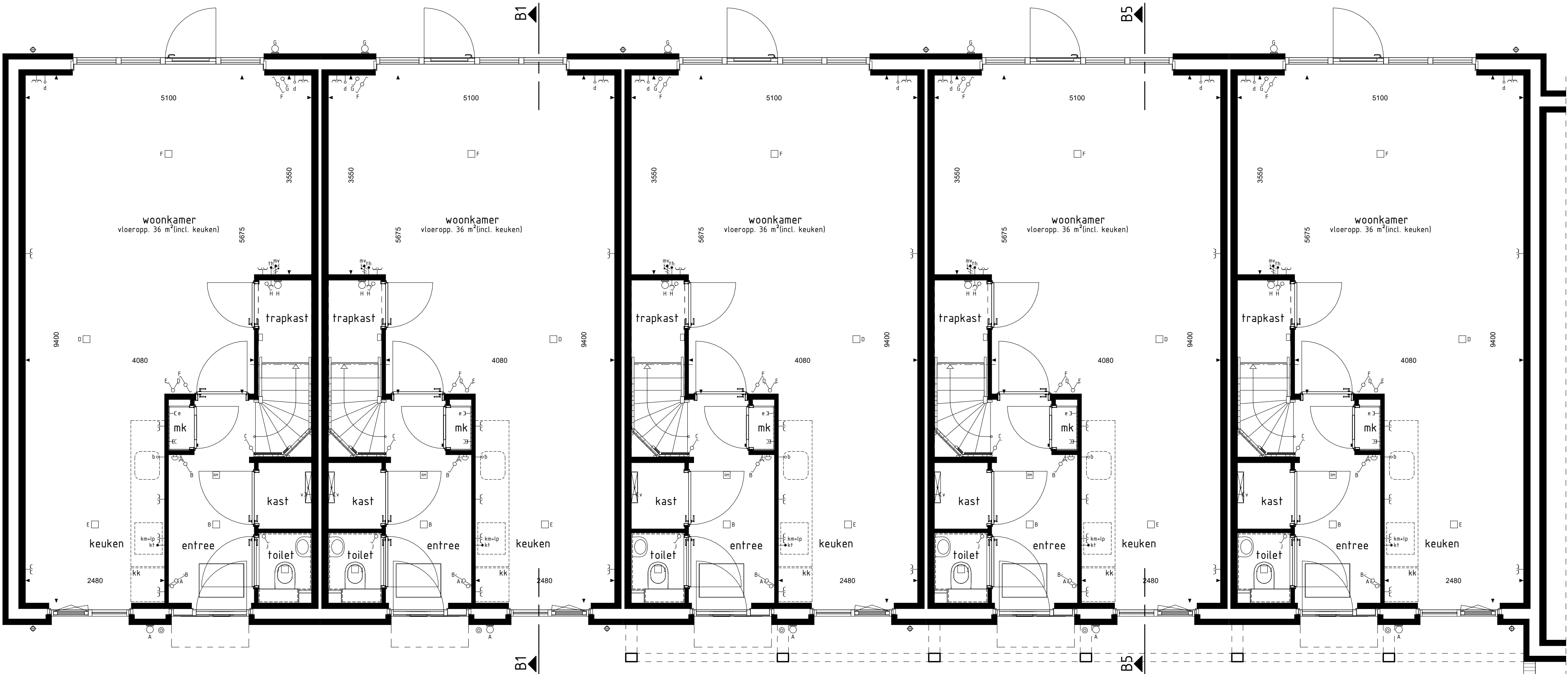
type A2sp bwnr get.:535 BEGANE GROND 1:50
