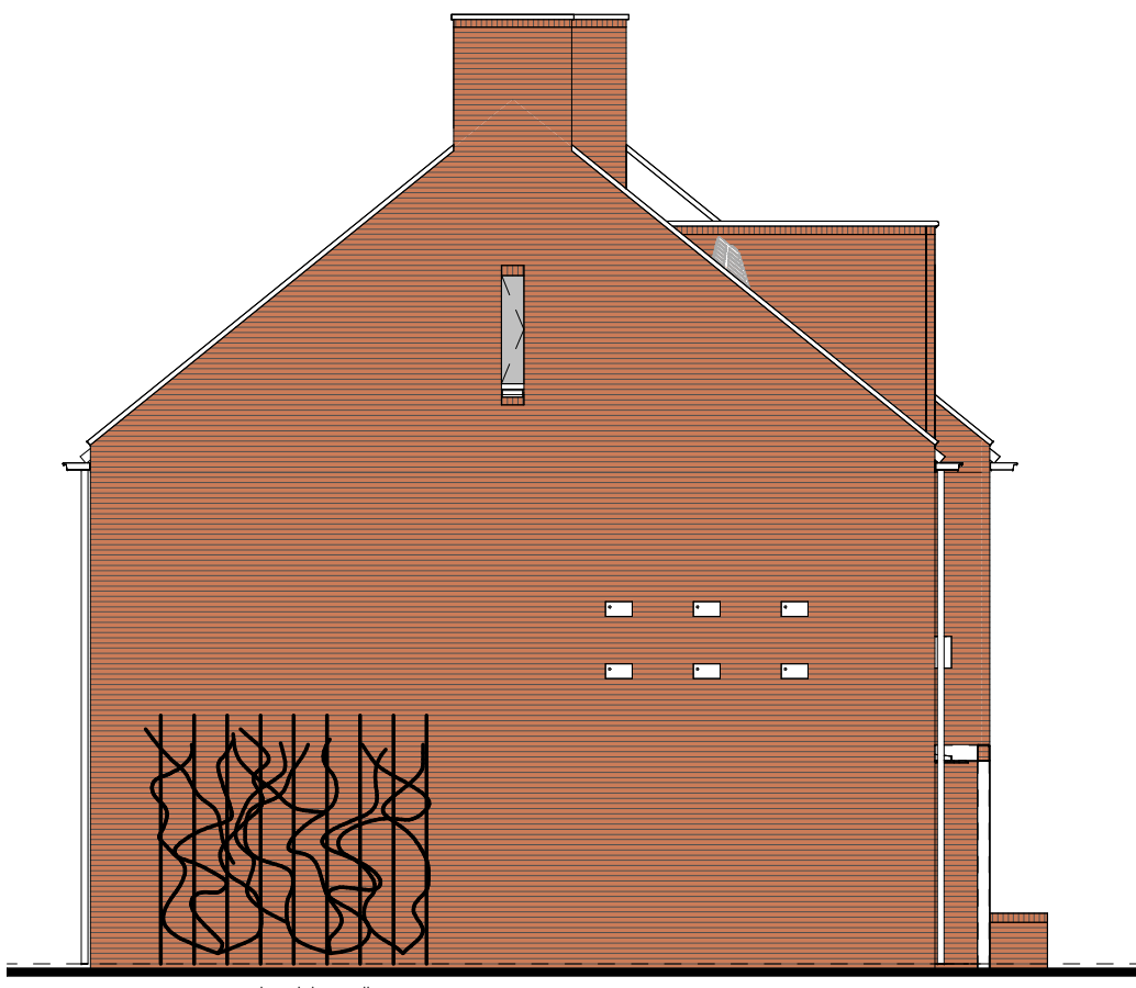
type A2sp bwnr get.:535 LINKERGEVEL 1:50
