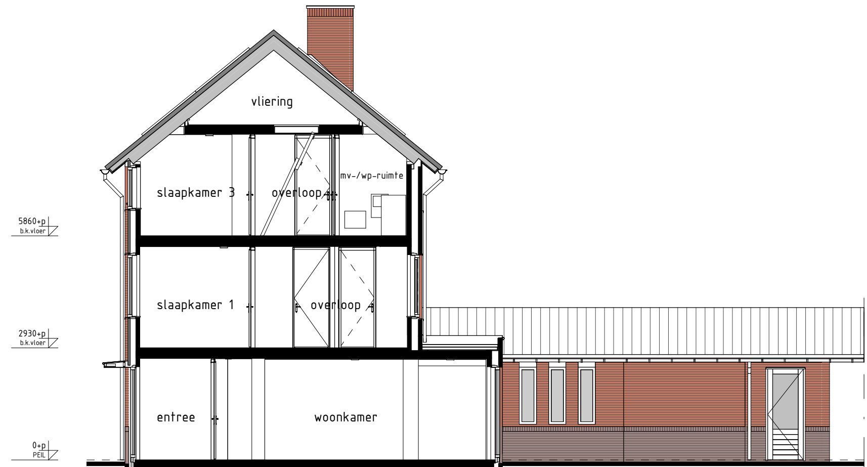
DOORSNEDE I1-I1 1:100
