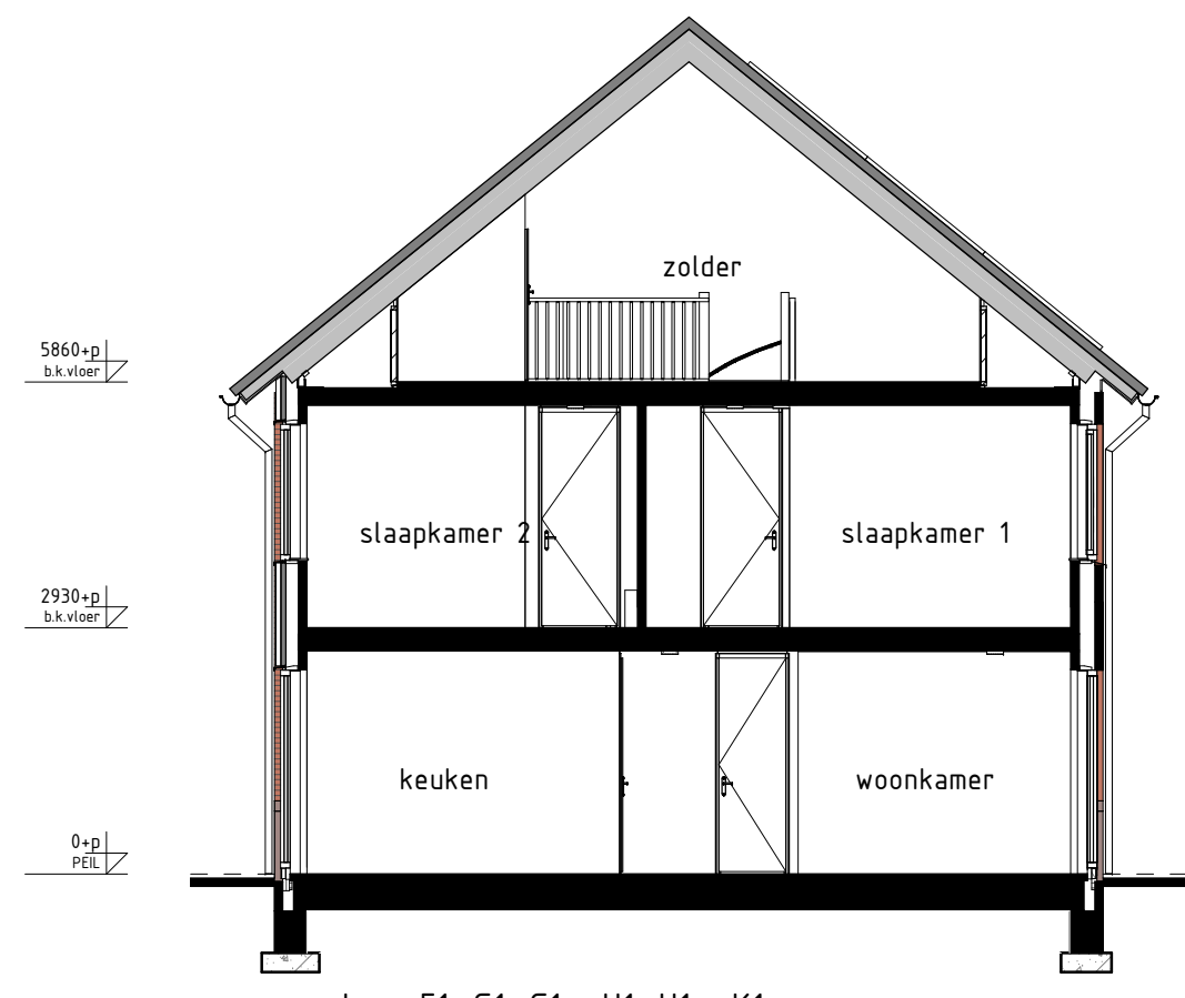
DOORSNEDE H1-H1 1:100
