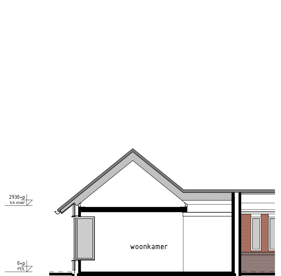
DOORSNEDE I2-I2 1:100
