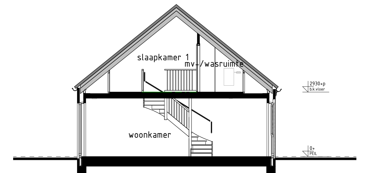
type R31, S31 bwnr get.:265, 266, 269, 270 DOORSNEDE A-A
