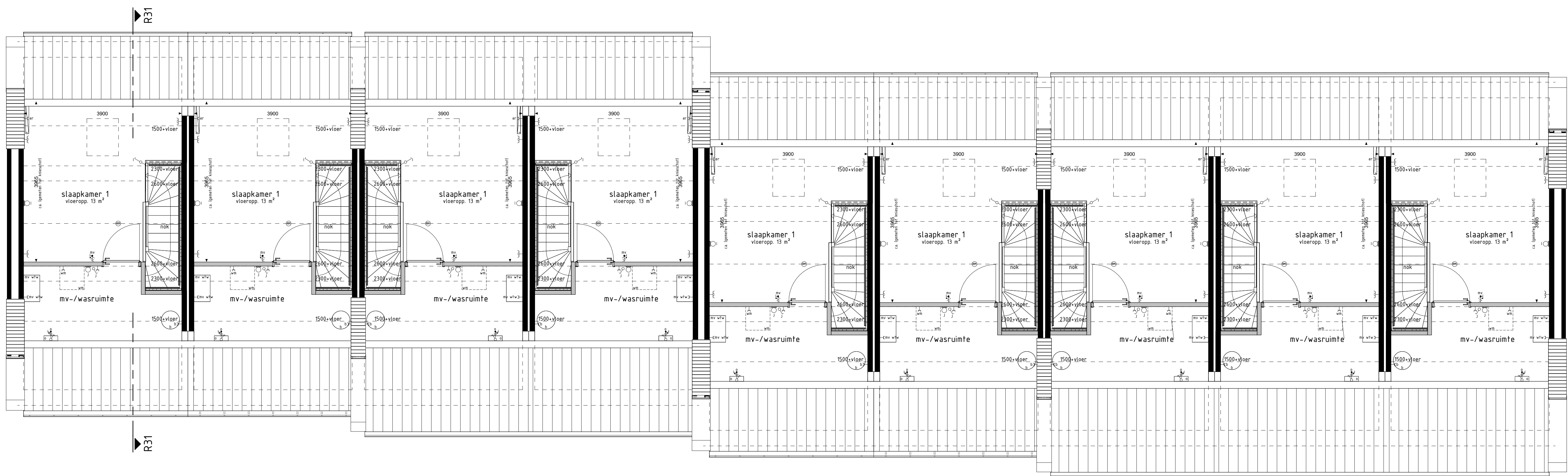
1e VERDIEPING
