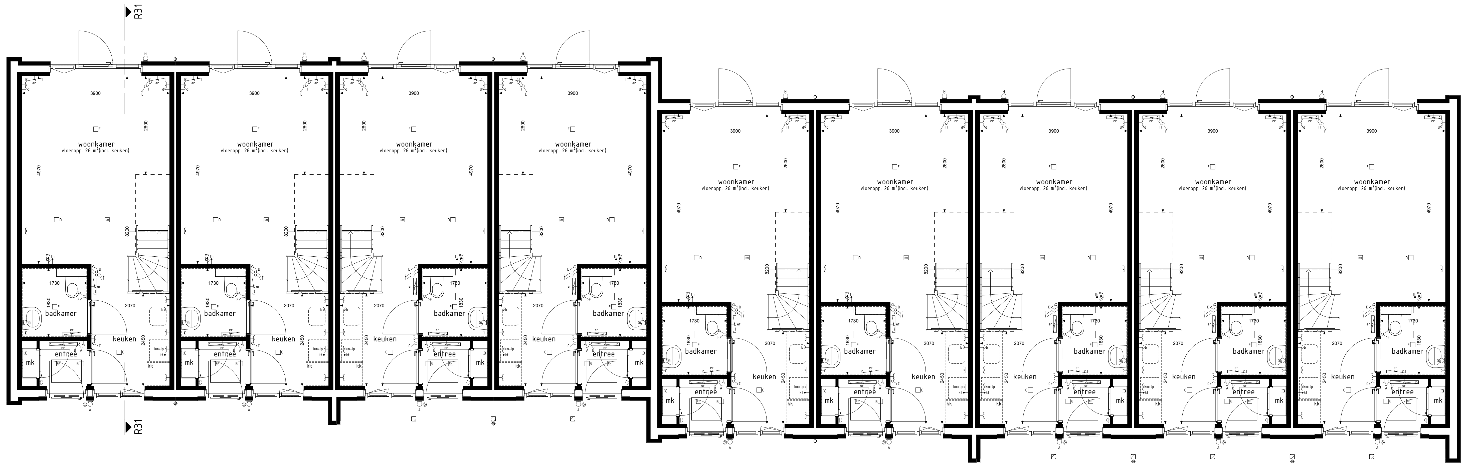
BEGANE GROND
