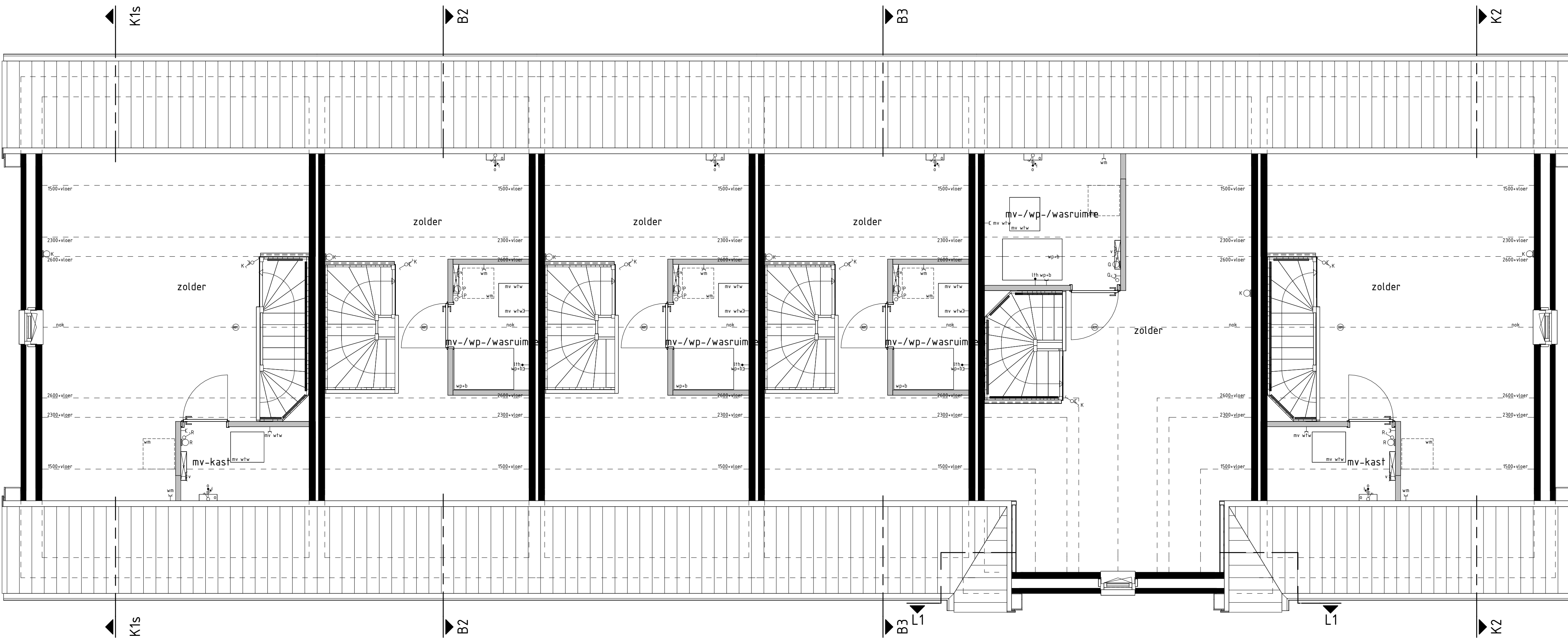
1e VERDIEPING 1:50
