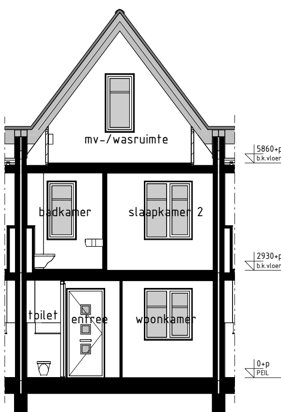
type H1s bwnr get.:175 DOORSNEDE H1s-H1s
