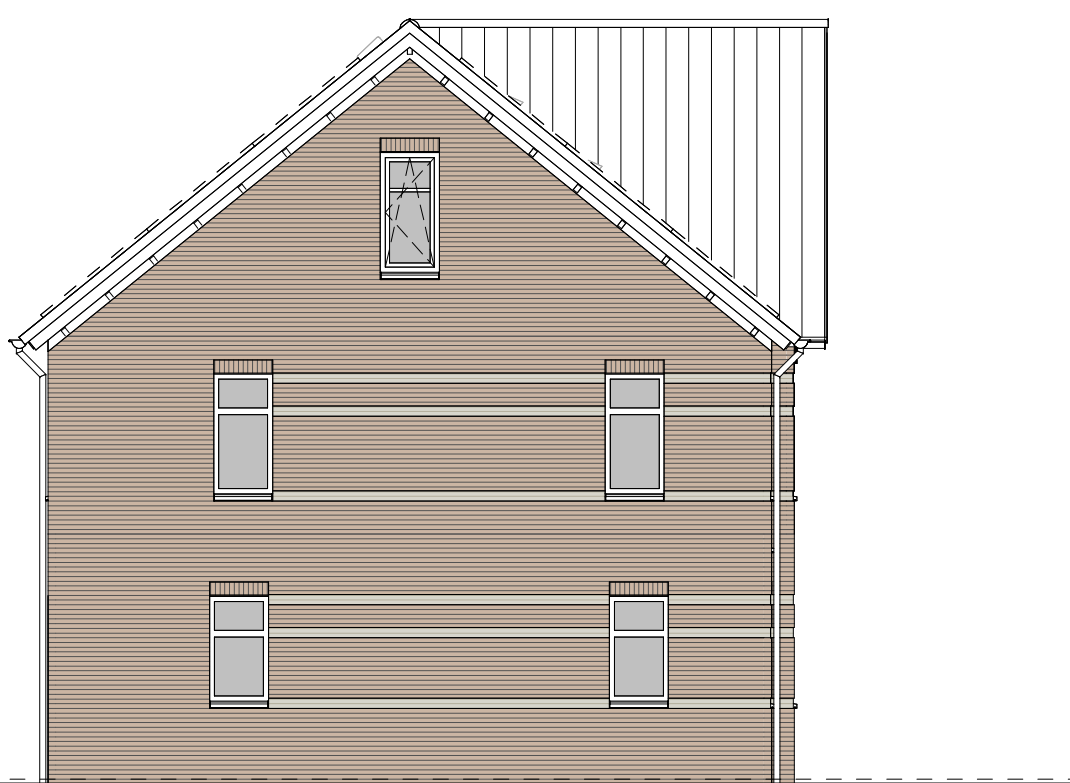
type F1s bwnr get.:172 LINKERGEVEL
