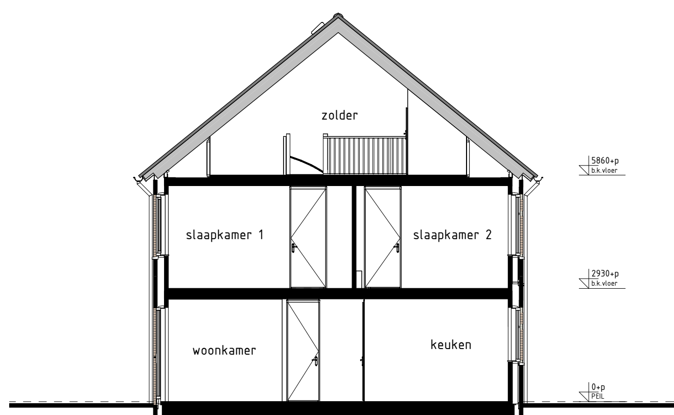
type F1, F1s bwnr get.:172 bwnr gesp.:178 DOORSNEDE F1s-F1s
