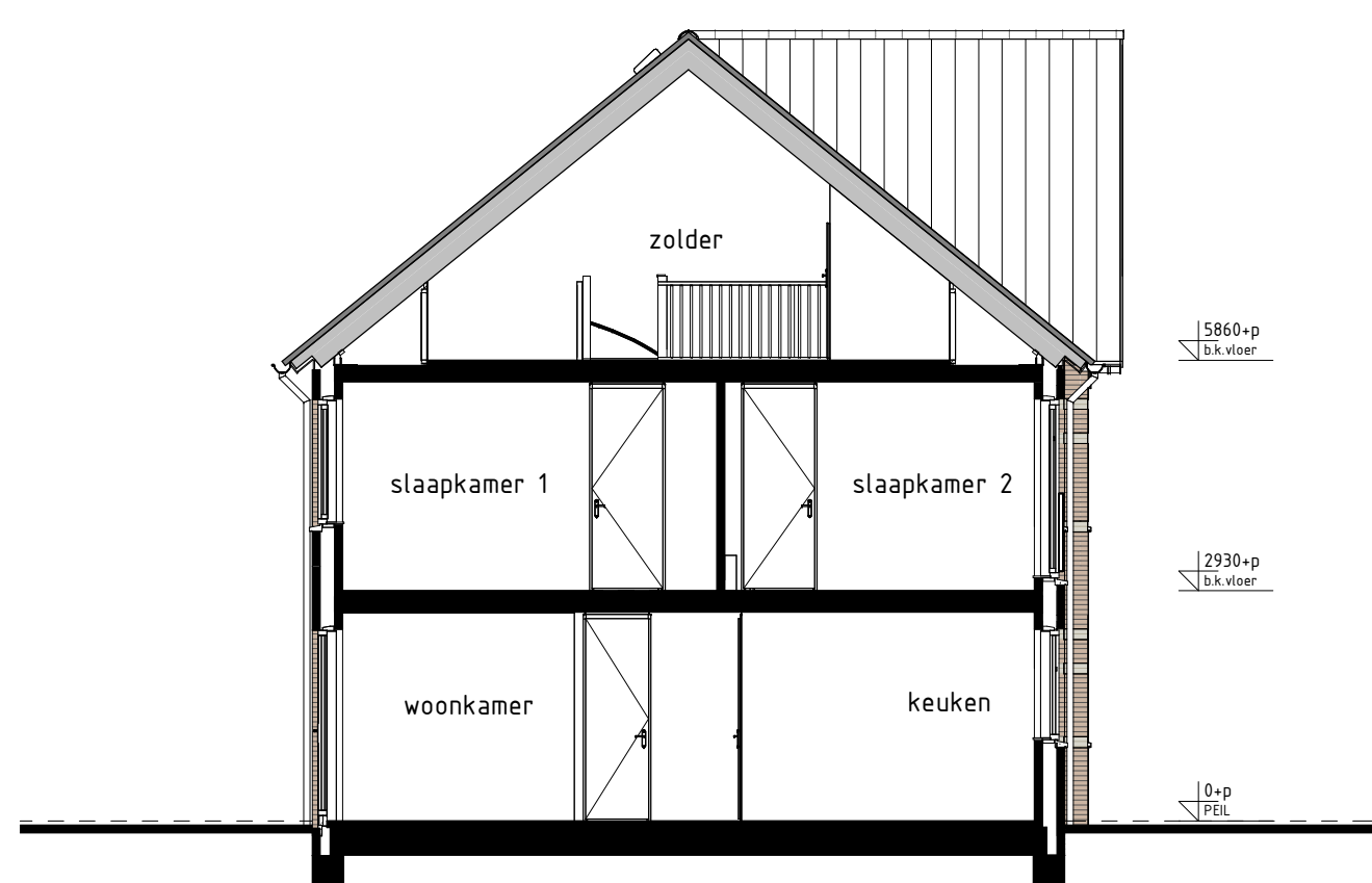
type G1, G1s bwnr get.:174,177 bwnr gesp.:173,176 DOORSNEDE G1s-G1s
