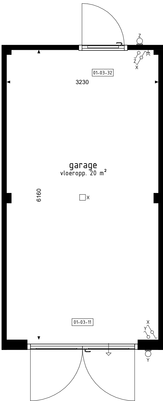
BEGANE GROND
