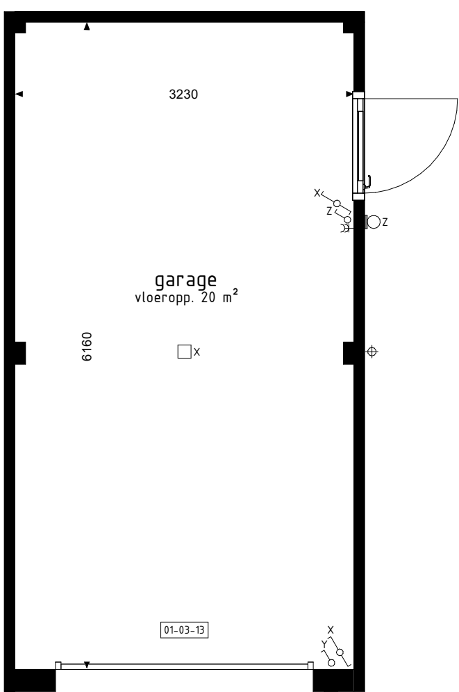
BEGANE GROND
