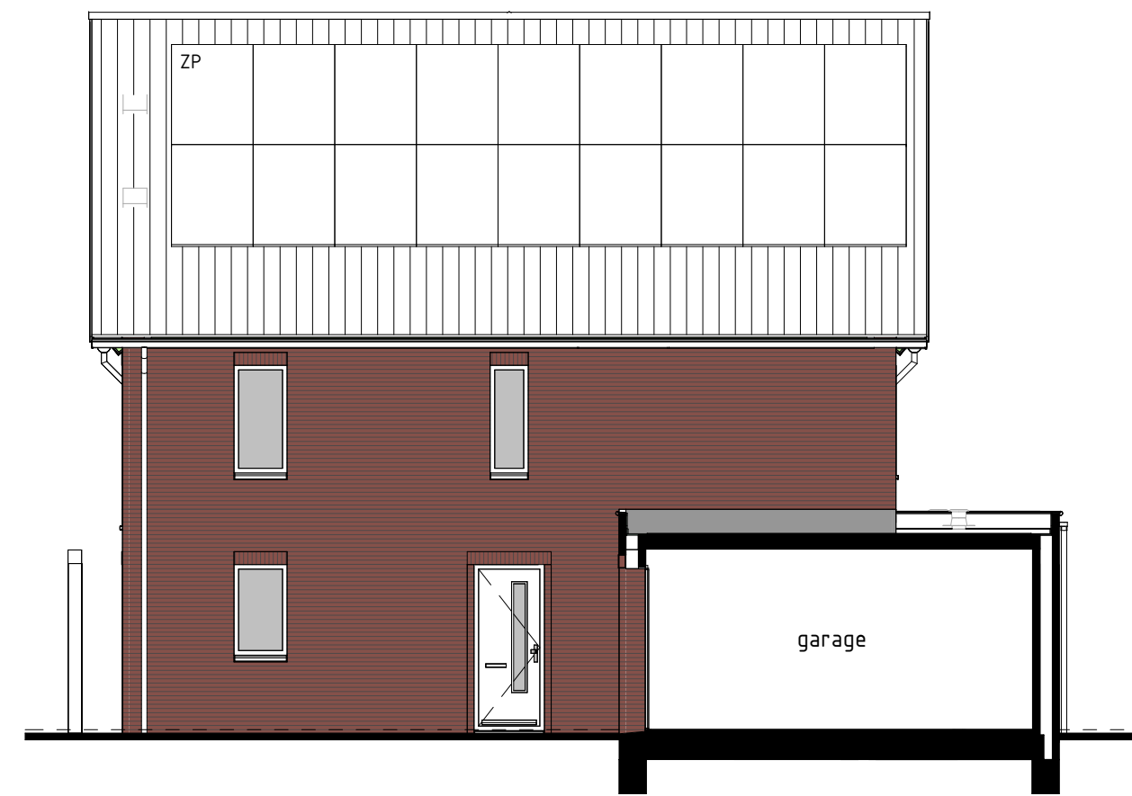
type H1sp bwnr get.:324 RECHTERGEVEL 1:100
