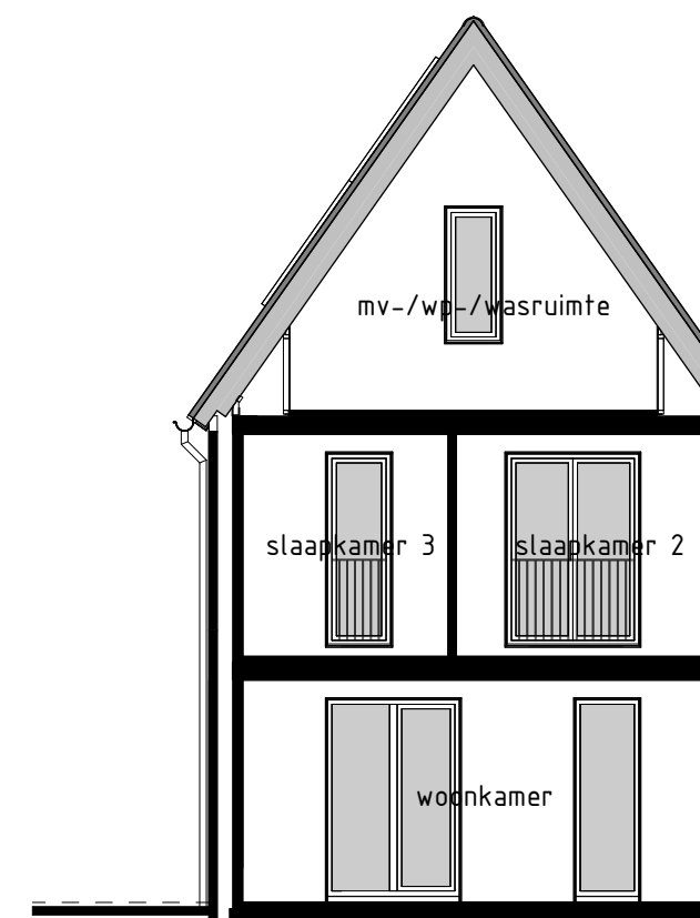
type H1sp bwnr get.:324 DOORSNEDE H1sp-H1sp 1:100
