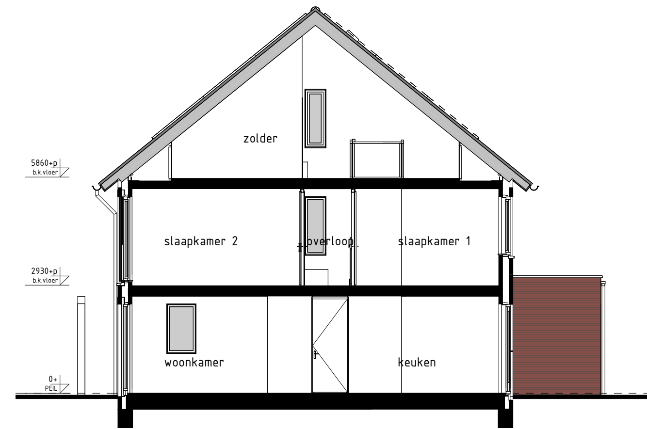
type H1, H2, H3sp bwnr get.:323, 325 bwnr gesp.:326 DOORSNEDE H1-H1 1:100
