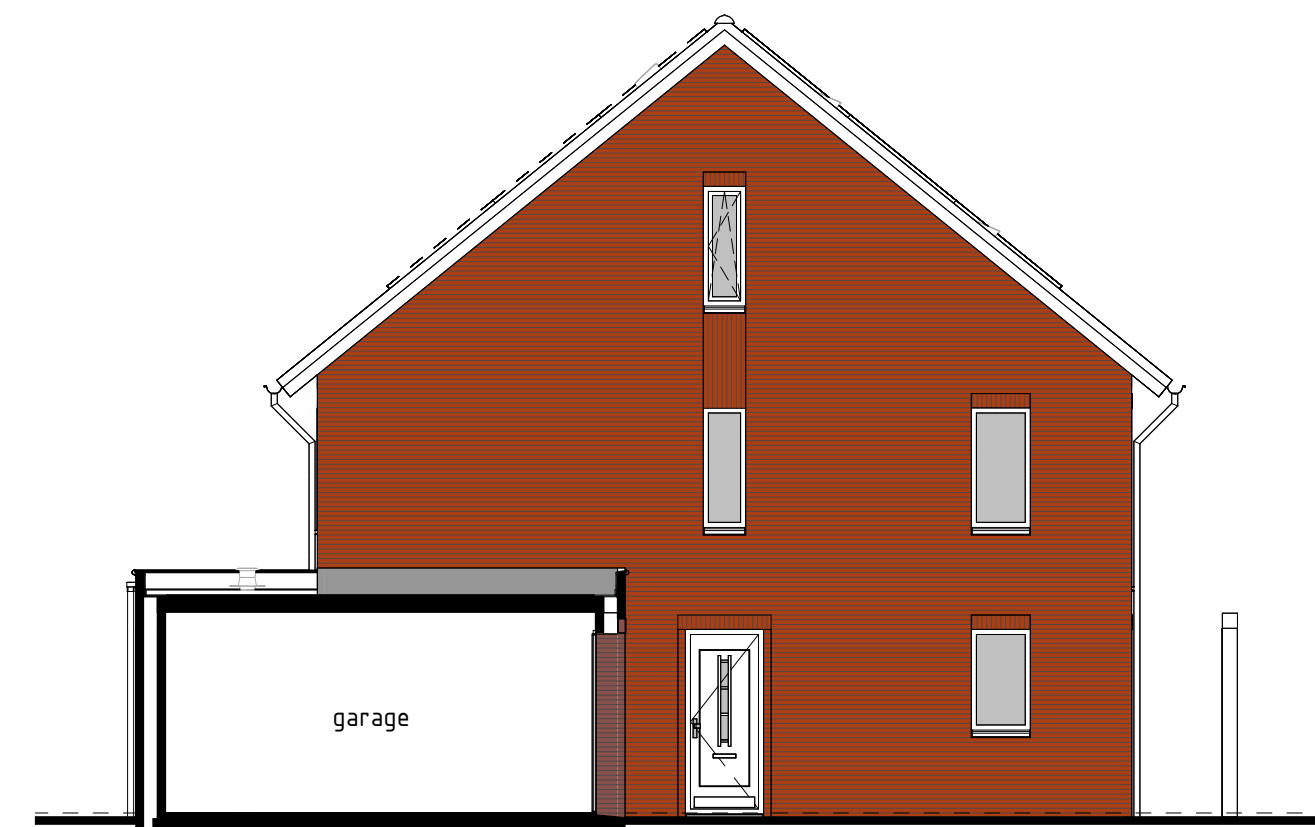
type H2 bwnr get.:325 LINKERGEVEL 1:100
