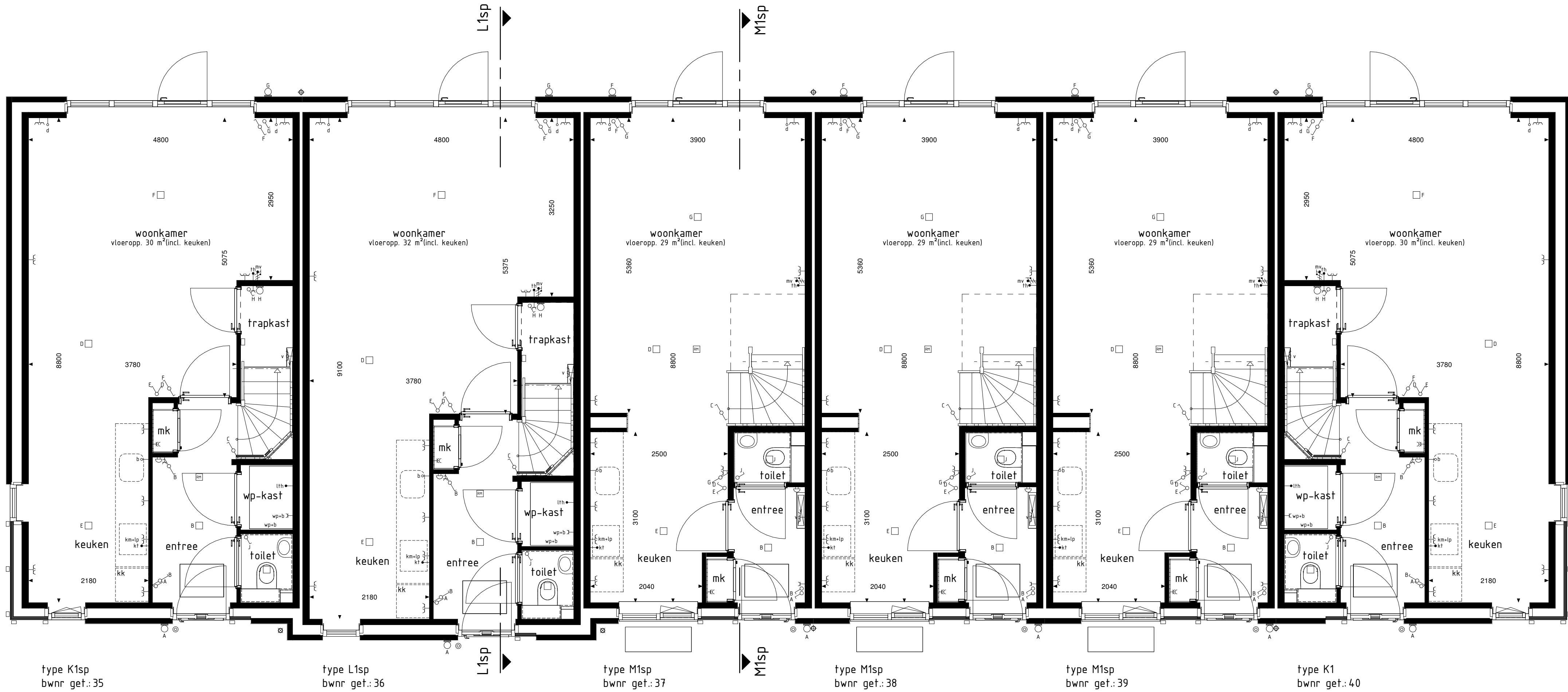
BEGANE GROND
