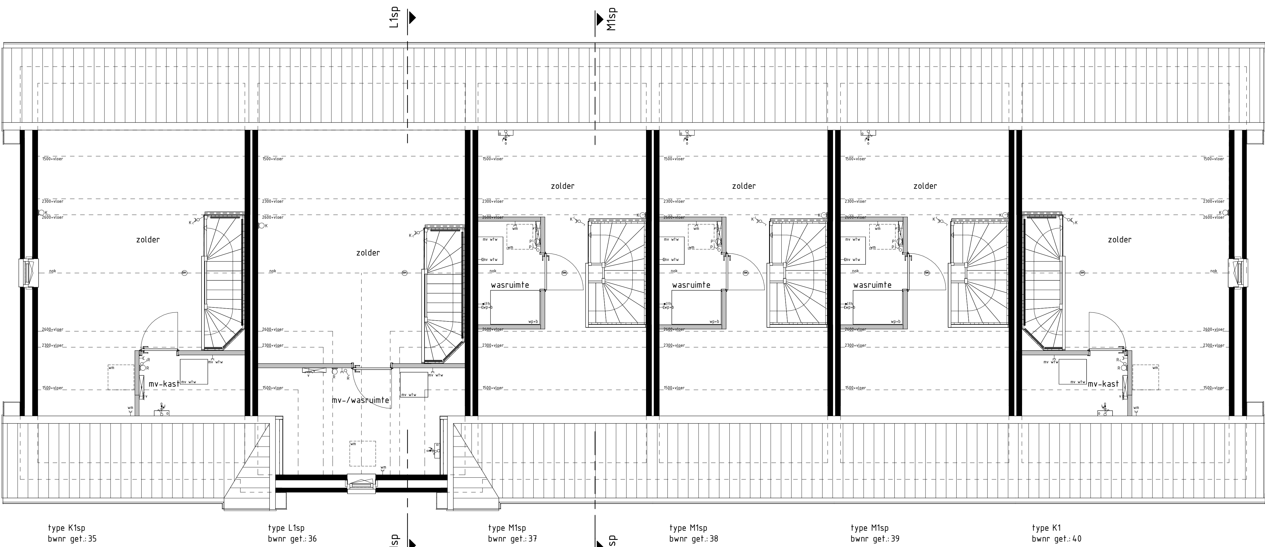
2e VERDIEPING
