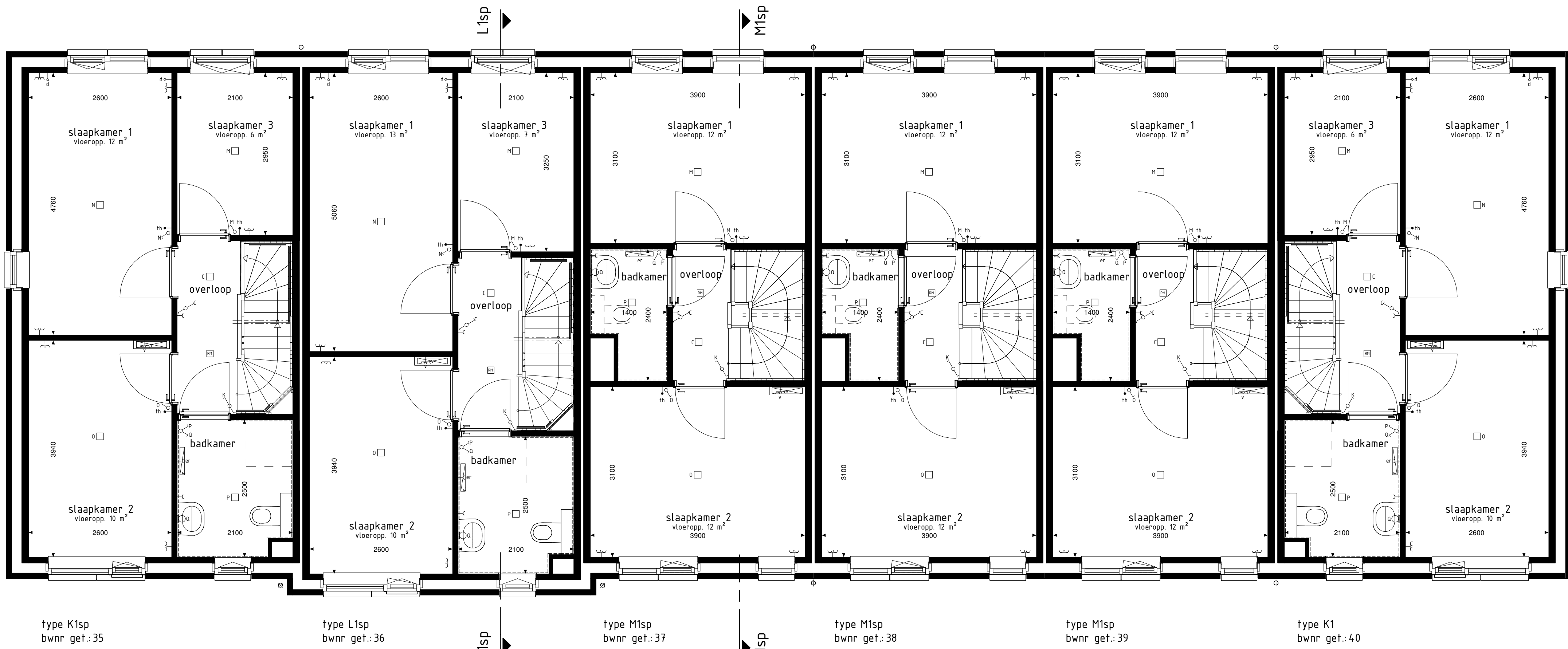
1e VERDIEPING
