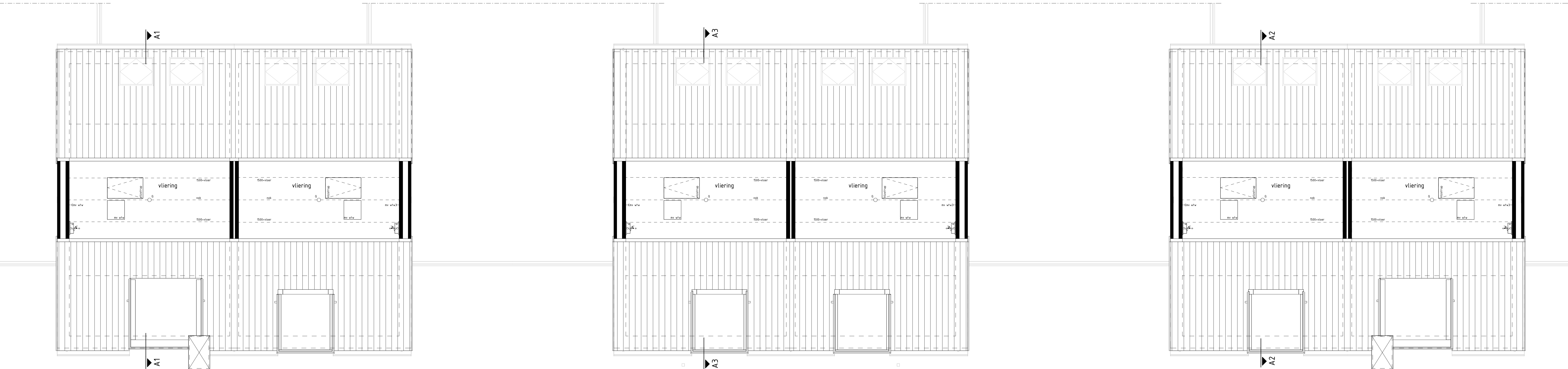
type A1 bwnr get.:1,7,13 2e VERDIEPING type A2s bwnr get.:2,8,14 type A3 bwnr get.:3,9,15 type A3s bwnr get.:4,10,16 type A2 bwnr get.:5,11,17 type A1s bwnr get.:6,12,18
