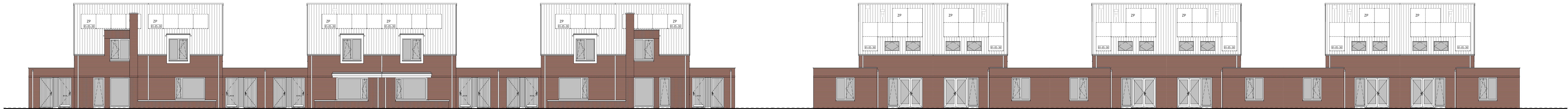
type A1 bwnr get.:1,7,13 VOERGEVEL type A2s bwnr get.:2,8,14 type A3 bwnr get.:3,9,15 type A3s bwnr get.:4,10,16 type A2 bwnr get.:5,11,17 type A1s bwnr get.:6,12,18 type A1s bwnr get.:6,12,18 ACHTERGEVEL type A2 bwnr get.:5,11,17 type A3s bwnr get.:4,10,16 type A3 bwnr get.:3,9,15 type A2s bwnr get.:2,8,14 type A1 bwnr get.:1,7,13
