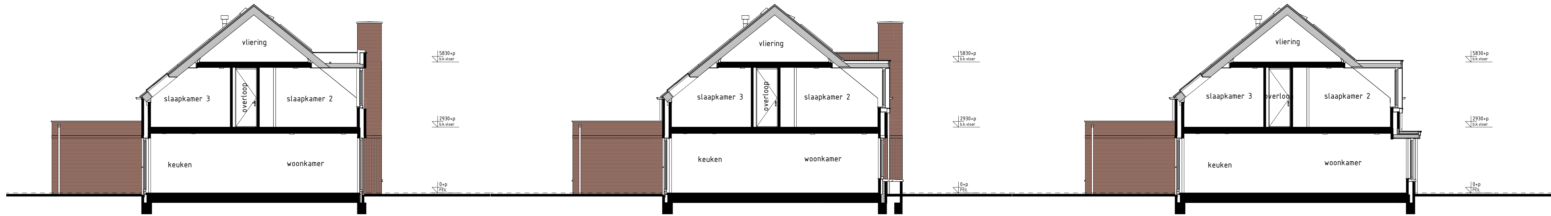
type A1 bwnr get.:1,7,13 bwnr gesp.:6,12,18 DOORSNEDE A1-A1 type A2 bwnr get.:5,11,17 bwnr gesp.:2,8,14 DOORSNEDE A2-A2 type A3 bwnr get.:3,9,15 bwnr gesp.:4,10,16 DOORSNEDE A3-A3
